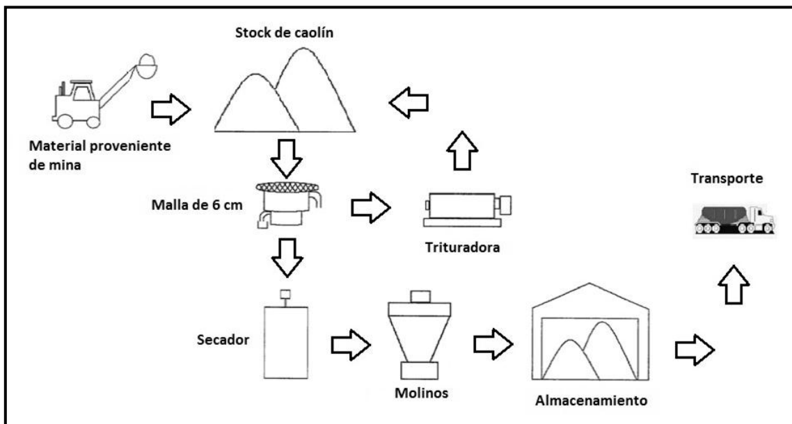
Ilustración 14. Diagrama de flujo de la operación en la planta
