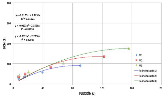
Figura 5.31 Relación entre tenacidades promedio BCN – 94 mm vs flexión: Regresión polinómica
