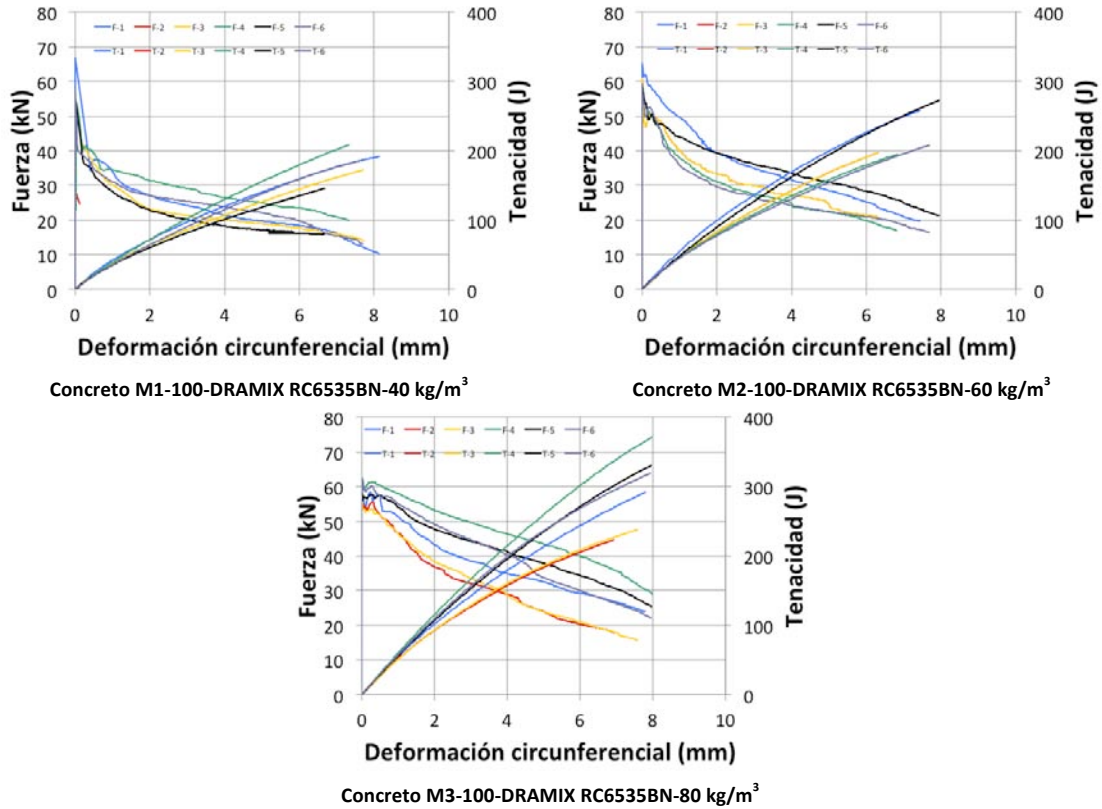
Figura 4.3 Curvas fuerza y tenacidad vs desplazamiento (probeta 100 mm)
