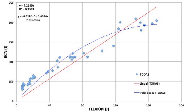
Figura 5.5 Relación entre tenacidades: BCN- 150 mm vs flexión (valores individuales)
