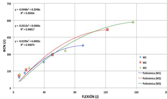
Figura 5.7 Relación entre tenacidades promedio BCN-150 mm vs flexión: Regresión polinómica.
