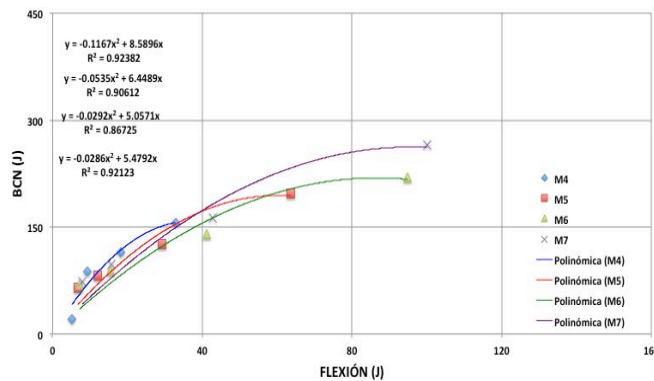
Figura 5.27 Relación entre tenacidades promedio BCN – 150 mm vs flexión: Regresión polinómica
