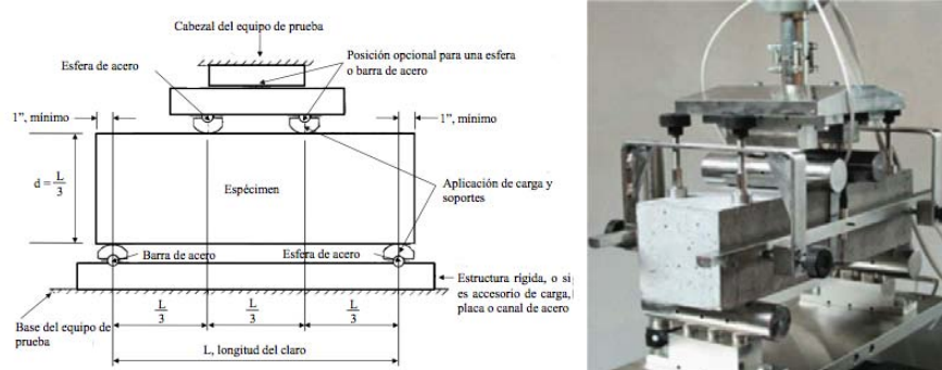
Figura 1.9 Ensayo de flexión con carga a los tercios (ASTM C1609)
