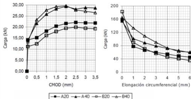
Figura 2.12 Curva de carga vs CMOD y \Delta\phi obtenidos a flexión y BCN
