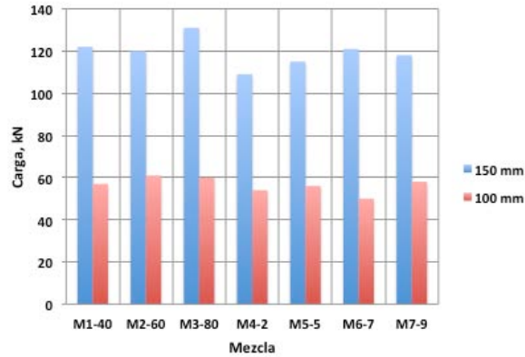
Figura 4.14 Comparación de cargas máximas para las probetas moldeadas
