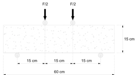
Figura 5.1 Ensayo ASTM C1609
