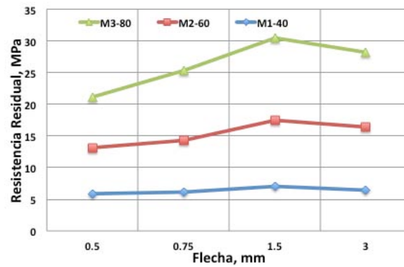
Figura 4.29 Comportamiento de resistencia residual (Fibra de acero)
