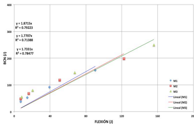
Figura 5.14 Relación entre tenacidades promedio BCN – 100 mm vs flexión: Regresión lineal.
