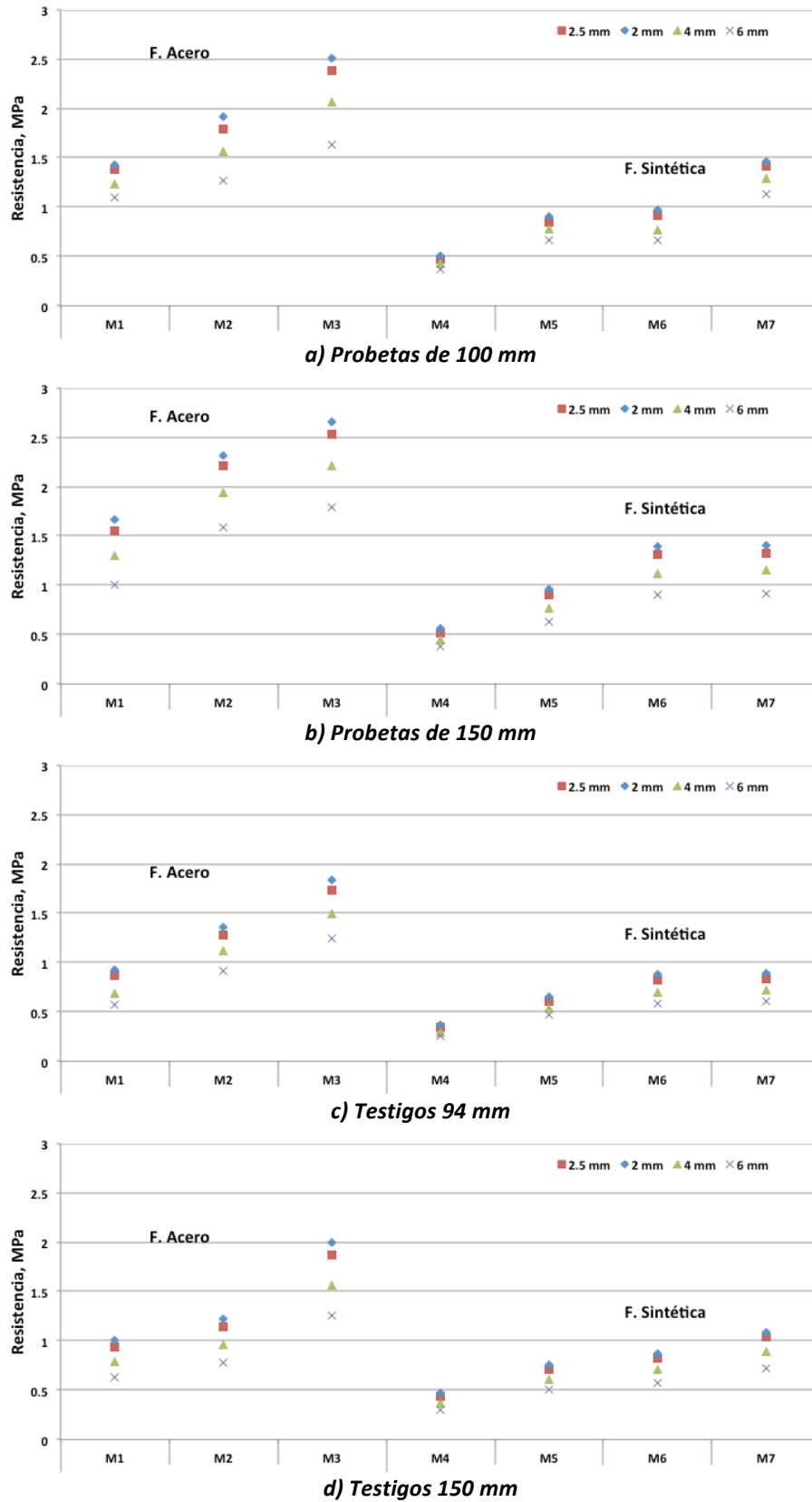
Figura 4.17 Variabilidad de la resistencia residual del ensayo Barcelona
