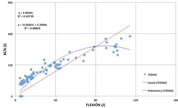
Figura 5.25 Relación entre tenacidades: BCN testigo– 150 mm vs flexión (valores individuales)
