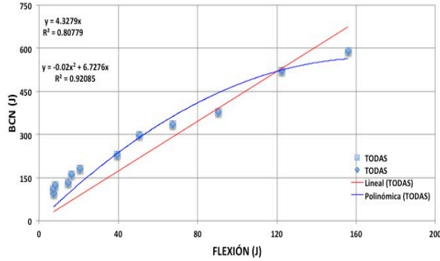
Figura 5.8 Relación entre tenacidades: BCN- 150 mm vs flexión (valores promedio)
