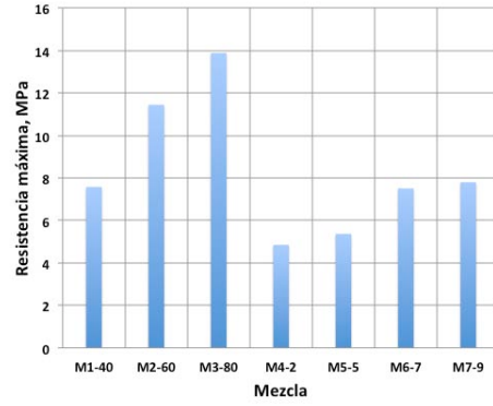
Figura 4.28 Comparación de resistencias máximas
