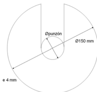
Figura 2.10 Disco de montaje
