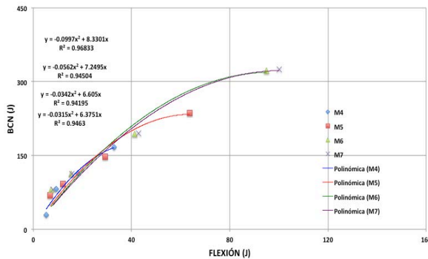
Figura 5.11 Relación entre tenacidades promedio BCN – 150 mm vs flexión: Regresión polinómica.
