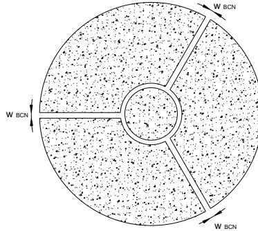
Figura 5.4 Modo de rotura asumido para el ensayo Barcelona
