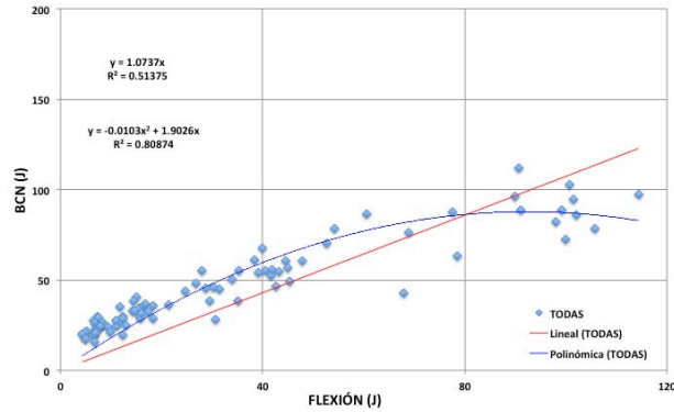
Figura 5.33 Relación entre tenacidades: BCN – 94 mm vs flexión (valores individuales)
