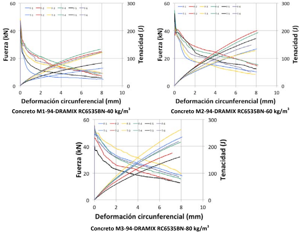
Figura 4.5 Curvas fuerza y tenacidad vs desplazamiento (testigo 94 mm)
