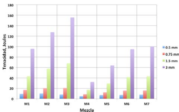
Figura 4.31 Comparación de tenacidad
