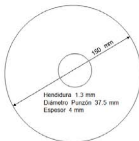
Figura 2.9 Disco de apoyo
