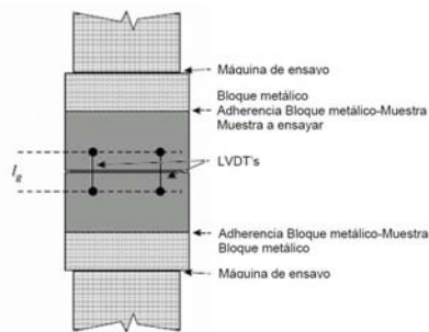
Figura 1.3 Configuración de ensayo de tracción uniaxial
