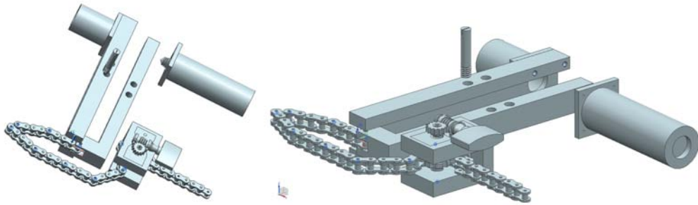
Figura 3.3 Esquema de fabricación de la cadena circunferencial y extensómetro
