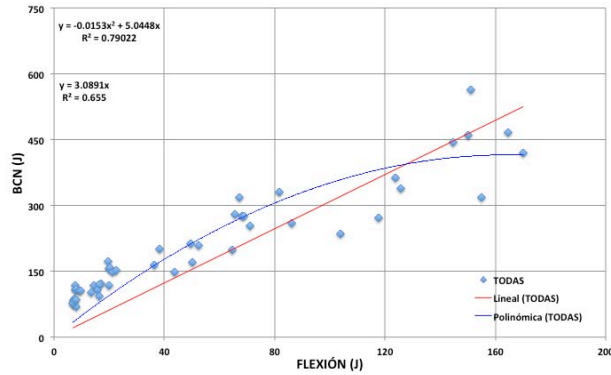
Figura 5.21 Relación entre tenacidades: BCN testigo – 150 mm vs flexión (valores individuales)
