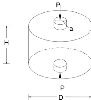
Figura 2.3 Posición de la probeta y los discos de carga (punzones)
