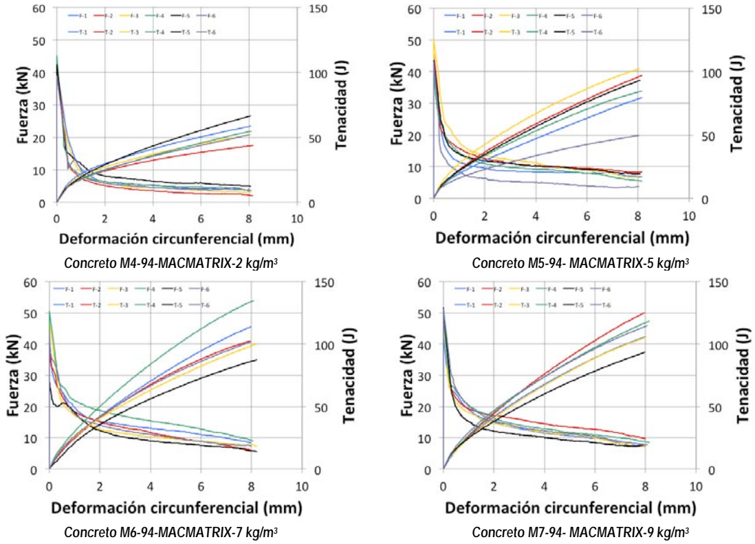
Figura 4.9 Curvas fuerza y tenacidad vs desplazamiento (testigo 94 mm)
