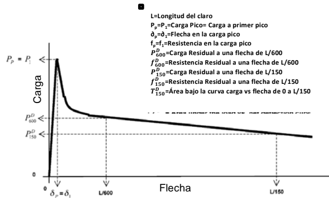
Figura 4.22 Curva carga vs flecha para determinar los parámetros de carga residual
