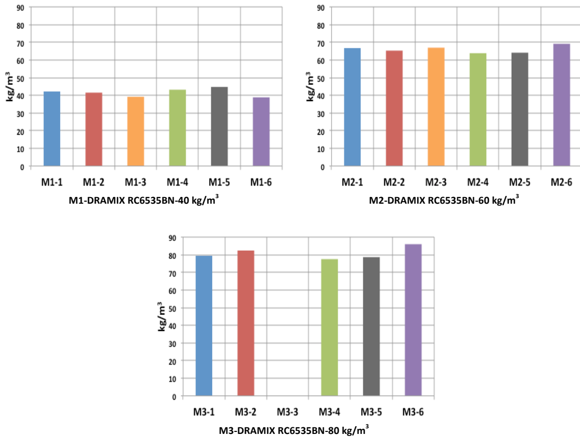
Figura 4.11 Conteo de fibras para probetas moldeadas de 150 mm
