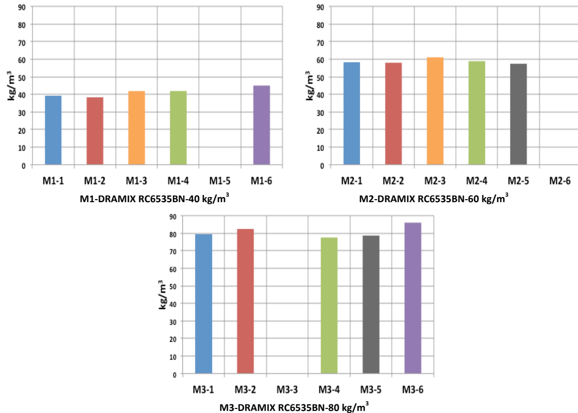
Figura 4.12 Conteo de fibras para probetas testigo de 150 mm
