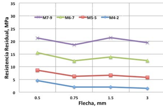
Figura 4.30 Comportamiento de resistencia residual (Fibra sintética)
