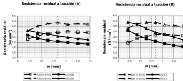
Figura 2.14 Resistencias residuales a tracción de los ensayos de flexión y Barcelona
