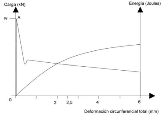
Figura 2.6 Curva de carga y energía vs deformación circunferencial
