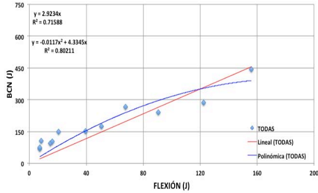
Figura 5.24 Relación entre tenacidades: BCN testigo – 150 mm vs flexión (valores promedio)
