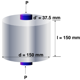
Figura 2.1 Ensayo Barcelona de doble punzonamiento
