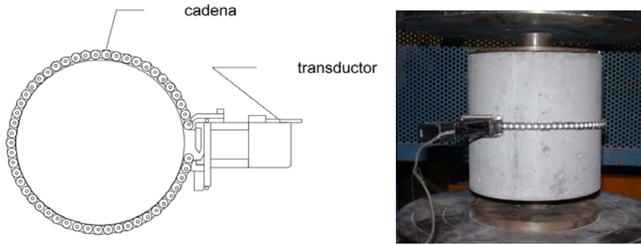
Figura 2.7 Cadena circunferencial y transductor
