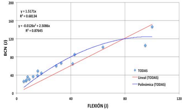
Figura 5.20 Relación entre tenacidades: BCN – 100 mm vs flexión (valores promedio)
