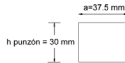
a) Esquema del disco de carga (punzón)
