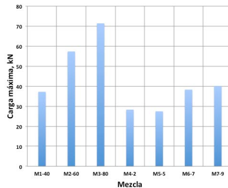
Figura 4.27 Comparación de cargas máximas
