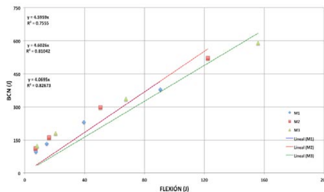
Figura 5.6 Relación entre tenacidades promedio BCN-150 mm vs flexión: Regresión lineal
