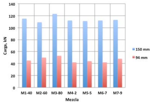
Figura 4.15 Comparación de cargas máximas para las probetas testigo
