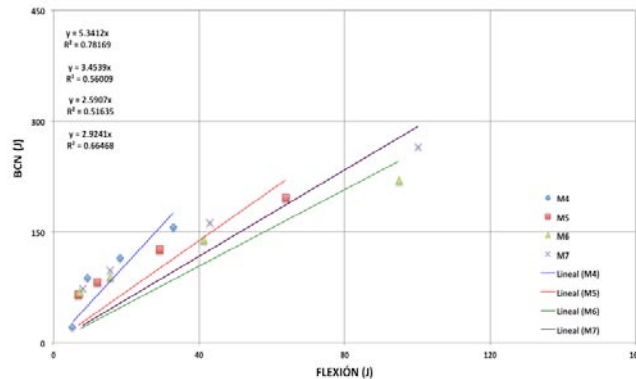
Figura 5.26 Relación entre tenacidades promedio BCN testigo– 150 mm vs flexión: Regresión Lineal
