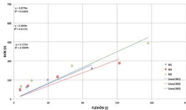
Figura 5.22 Relación entre tenacidades promedio BCN testigo – 150 mm vs flexión: Regresión lineal
