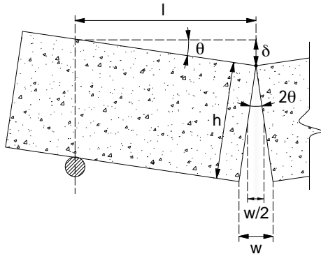
Figura 5.3 Detalle del modo de rotura asumido para el ensayo ASTM C1609
