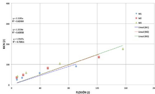
Figura 5.30 Relación entre tenacidades promedio BCN – 94 mm vs flexión: Regresión lineal
