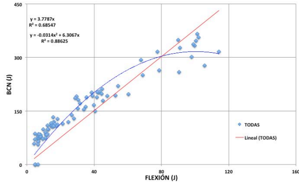
Figura 5.9 Relación entre tenacidades: BCN- 150 mm vs flexión (valores individuales)
