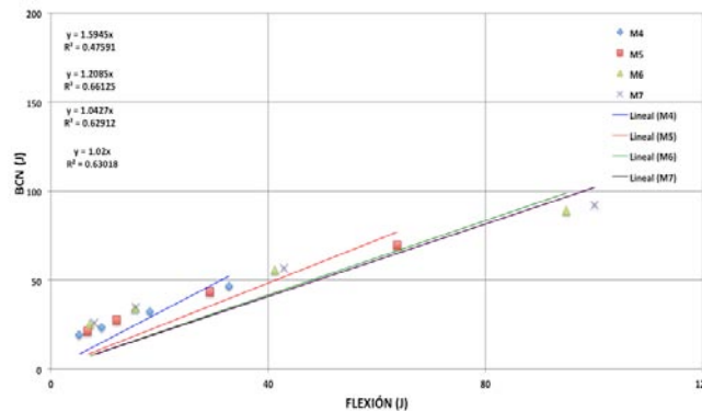
Figura 5.34 Relación entre tenacidades promedio BCN – 94 mm vs flexión: Regresión Lineal
