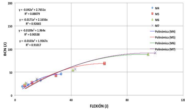
Figura 5.35 Relación entre tenacidades promedio BCN – 94 mm vs flexión: Regresión polinómica
