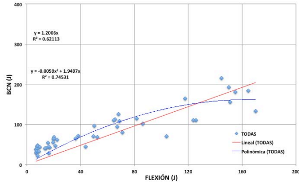
Figura 5.29 Relación entre tenacidades: BCN – 94 mm vs flexión (valores individuales)
