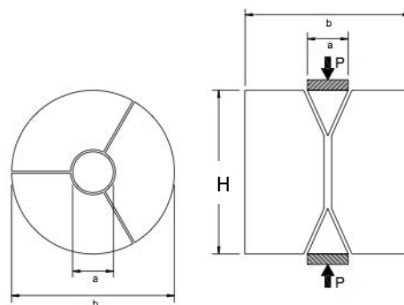
Figura 2.5 Mecanismo idealizado de rotura, vista en planta y longitudinal
