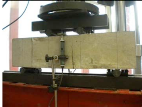
Figura 4.24 Modo de falla típico del ensayo de flexión
