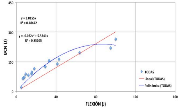
Figura 5.28 Relación entre tenacidades: BCN testigo– 150 mm vs flexión (valores promedio)
