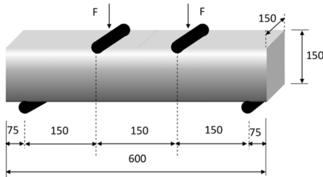
Figura 4.21 Esquema de viga de ensayo
