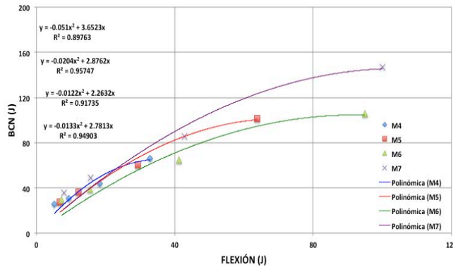
Figura 5.19 Relación entre tenacidades promedio BCN – 100 mm vs flexión: Regresión polinómica.
