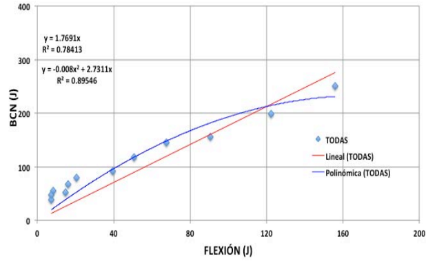
Figura 5.16 Relación entre tenacidades: BCN – 100 mm vs flexión (valores promedio)
