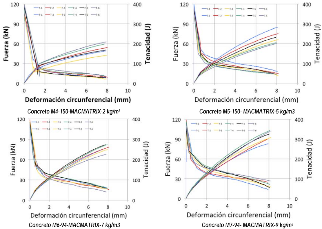
Figura 4.10 Curvas fuerza y tenacidad vs desplazamiento (testigo 150 mm)
