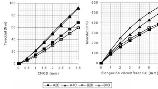
Figura 2.13 Curva de tenacidad vs CMOD y \Delta\phi obtenidos a flexión y BCN
