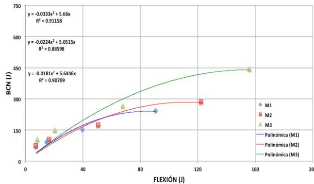
Figura 5.23 Relación entre tenacidades promedio BCN testigo – 150 mm vs flexión: Regresión polinómica.
