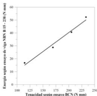
Figura 2.11 Regresión entre los resultados del ensayo Barcelona (BCN) y Belga (NBN)
