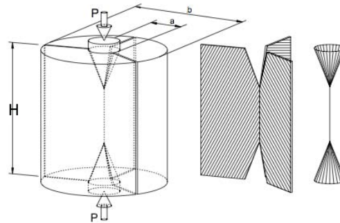
Figura 2.4 Esquema del mecanismo de falla
