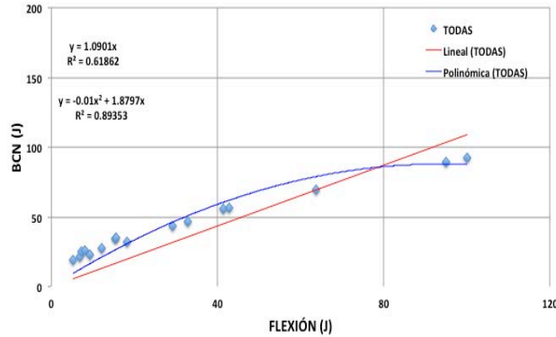
Figura 5.36 Relación entre tenacidades: BCN – 94 mm vs flexión (valores promedio)
