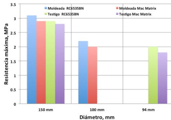
Figura 4.16 Comparación de resistencia máxima de probetas moldeadas y testigo.
