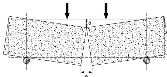
Figura 5.2 Hipótesis de fisuración para el ensayo ASTM C1609
