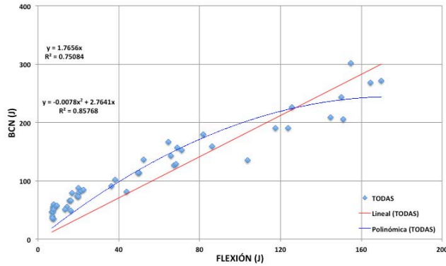
Figura 5.13 Relación entre tenacidades: BCN – 100 mm vs flexión (valores individuales)
