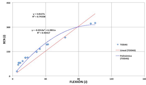
Figura 5.12 Relación entre tenacidades: BCN – 150 mm vs flexión (valores promedio)
