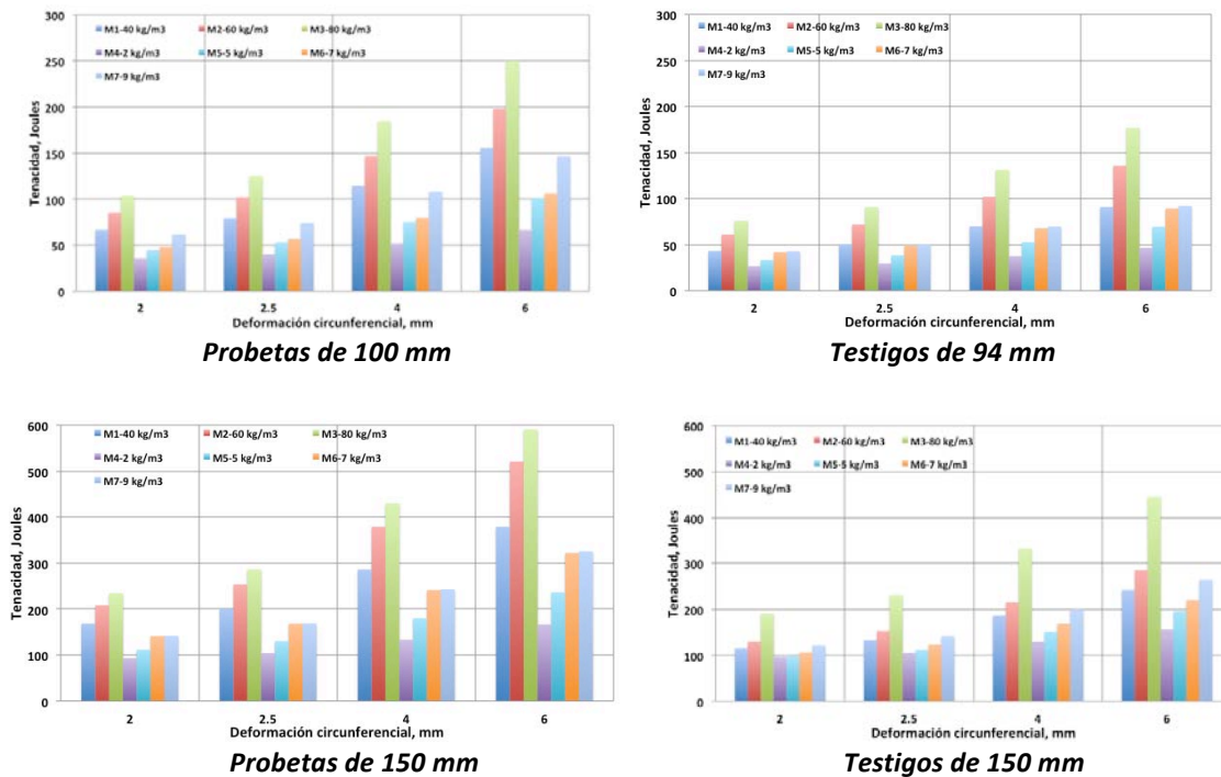
Figura 4.19 Resultados de tenacidad del ensayo Barcelona
