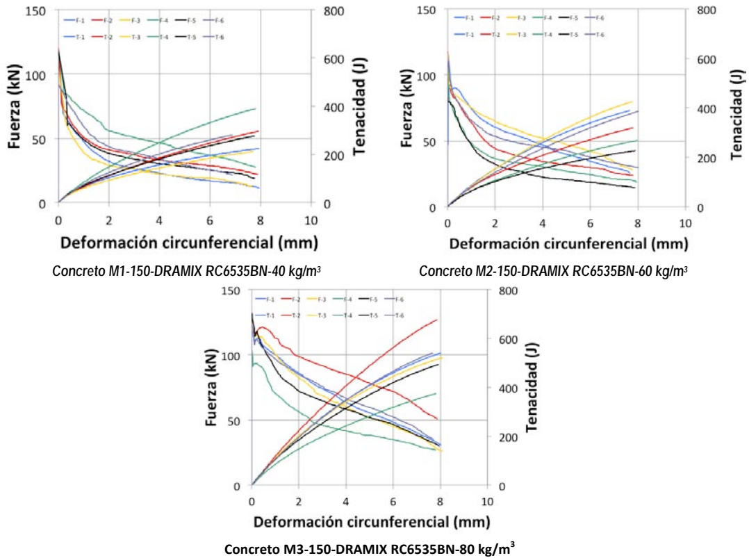
Figura 4.6 Curvas fuerza y tenacidad vs desplazamiento (testigo 150 mm)
