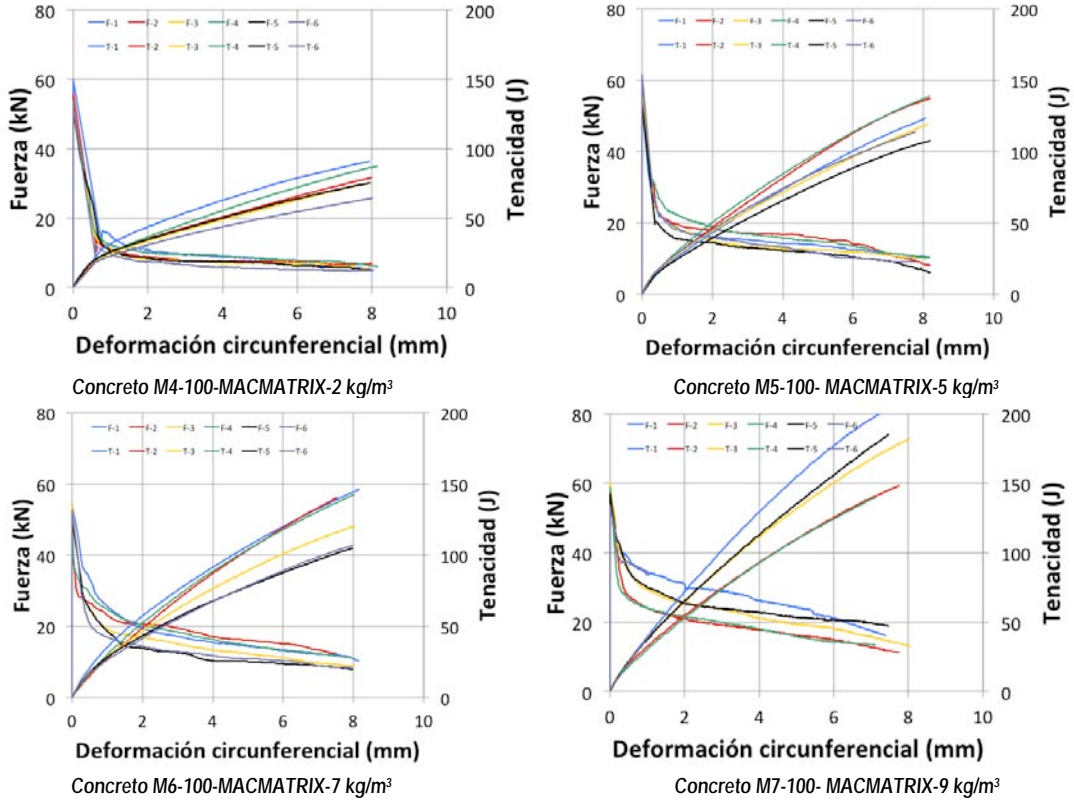
Figura 4.7 Curvas fuerza y tenacidad vs desplazamiento (probeta 100 mm)
