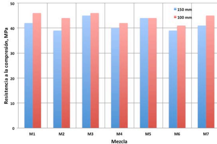
Figura 4.1 Resistencia a compresión promedio
