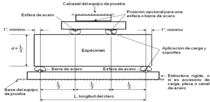
Figura 4.20 Dispositivo de carga a los tercios
