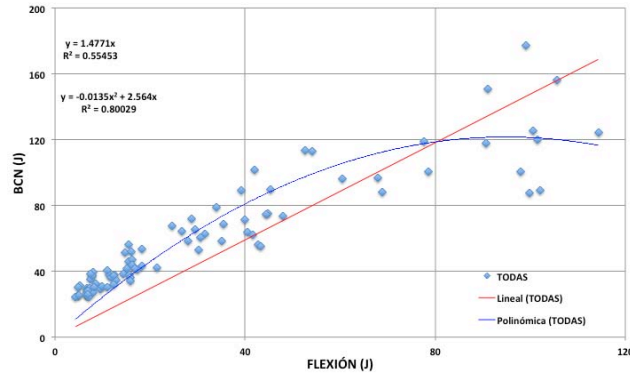
Figura 5.17 Relación entre tenacidades: BCN – 100 mm vs flexión (valores individuales)
