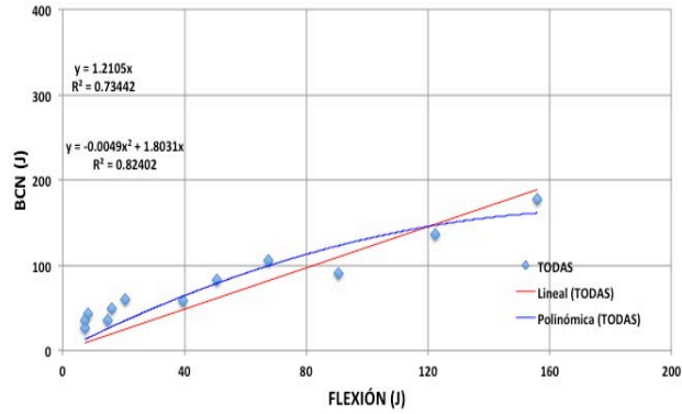
Figura 5.32 Relación entre tenacidades: BCN – 94 mm vs flexión (valores promedio)
