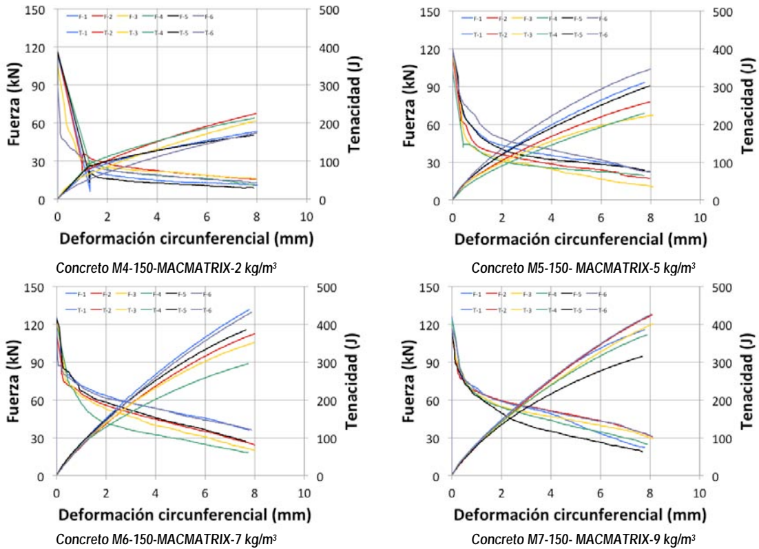
Figura 4.8 Curvas fuerza y tenacidad vs desplazamiento (probeta 150 mm)
