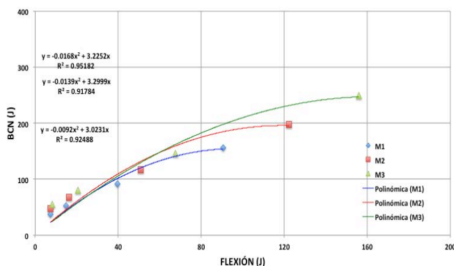
Figura 5.15 Relación entre tenacidades promedio BCN – 100 mm vs flexión: Regresión polinómica.
