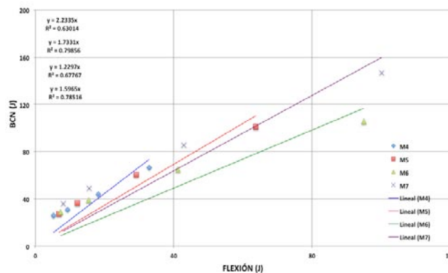
Figura 5.18 Relación entre tenacidades promedio BCN – 100 mm vs flexión : Regresión lineal.
