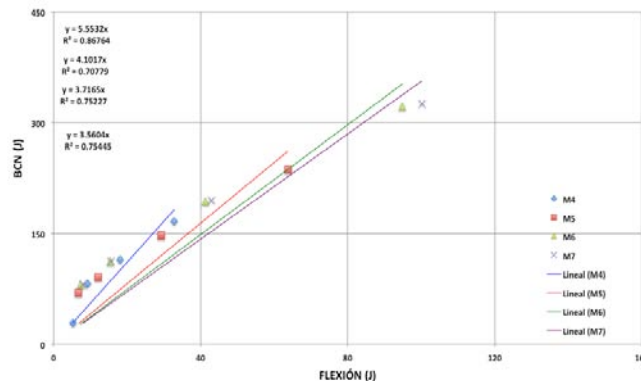
Figura 5.10 Relación entre tenacidades promedio BCN – 150 mm vs flexión : Regresión lineal
