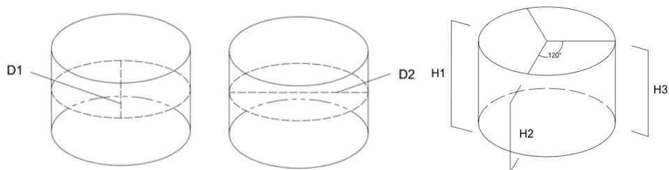
Figura 2.2 Determinación del diámetro y altura de la probeta
