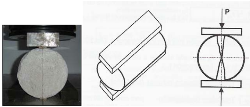
Figura 1.7 Ensayo brasileño - esquema de rotura y fisuración
