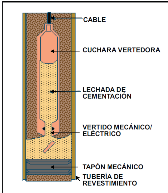
FIG.2.3 Método de cuchara vertedora
