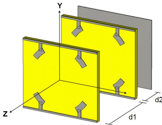
Fig. 4.23. Vista de la celda unitaria de la estructura de dos capas de anillos interconectados. Modelo optimizado para operar en la banda Ku-K-Ka.
