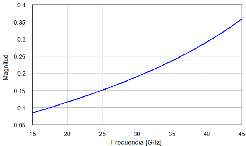
Fig. 3.9. Coeficiente de reflexión para una polarización vertical. Simulación del circuito equivalente para un arreglo de anillos ranurados ( L=1 [nH], C=0.015 [pF] y C1=0.00658 [pF])
