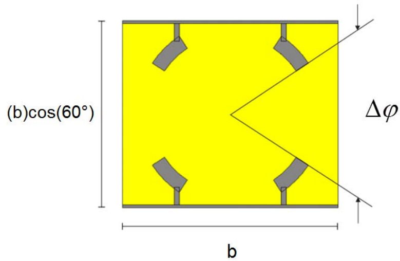
Fig. 4.7. Vista frontal de la celda unitaria de la estructura basada en anillos interconectados. Ambas capas contienen celda de la misma configuración y medidas.
