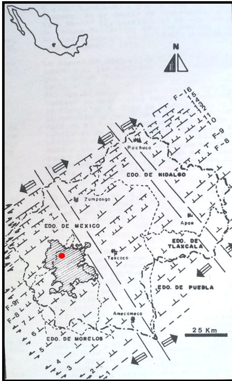
Figura 3.5. Modelo estructural de la Cuenca de México (Aguayo Camargo, et. al., 1989).
