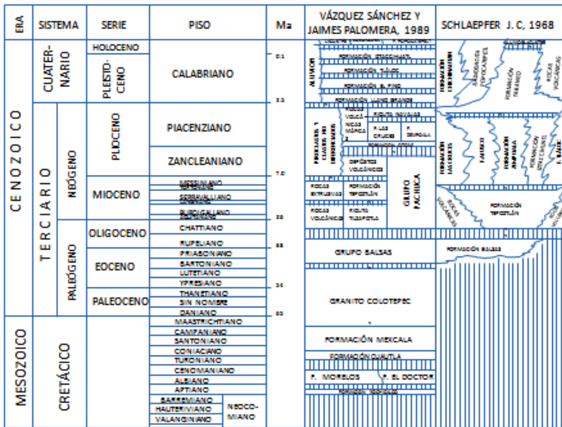
Figura 3.4. Estratigrafía de la Cuenca de México, modificada de Vázquez Sánchez y Jaimes Palomera en 1989. (tomada de Enciso De la Vega, 1992).
