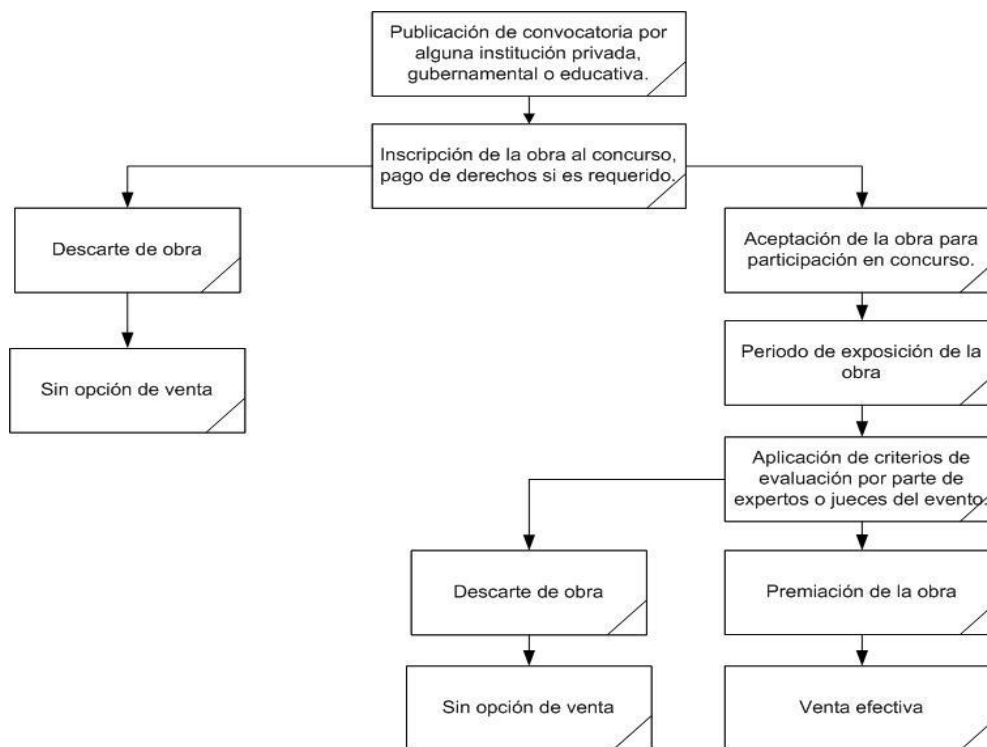
Figura 3.1.1 Concursos
