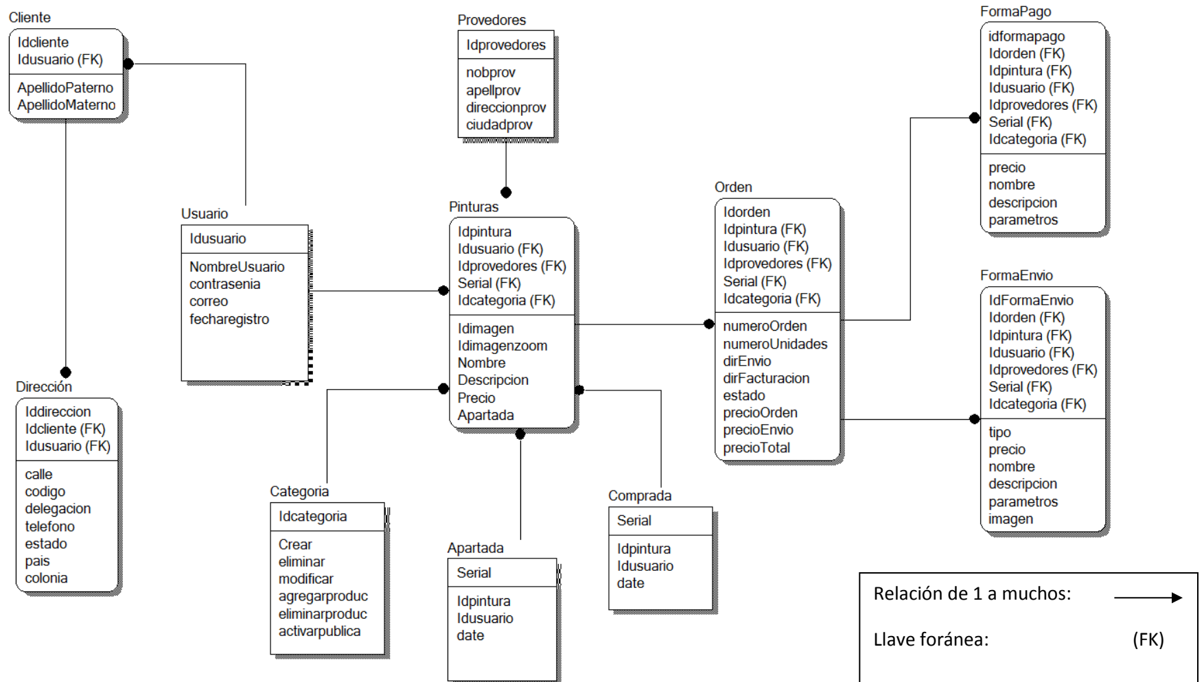
Imagen 4.1.4.1. Diagrama Entidad-Relación
