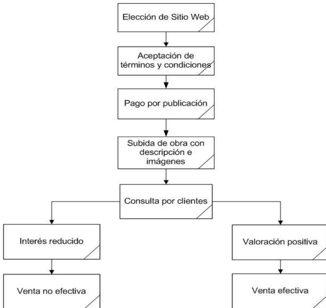
Fig. 3.1.7 Páginas Web
