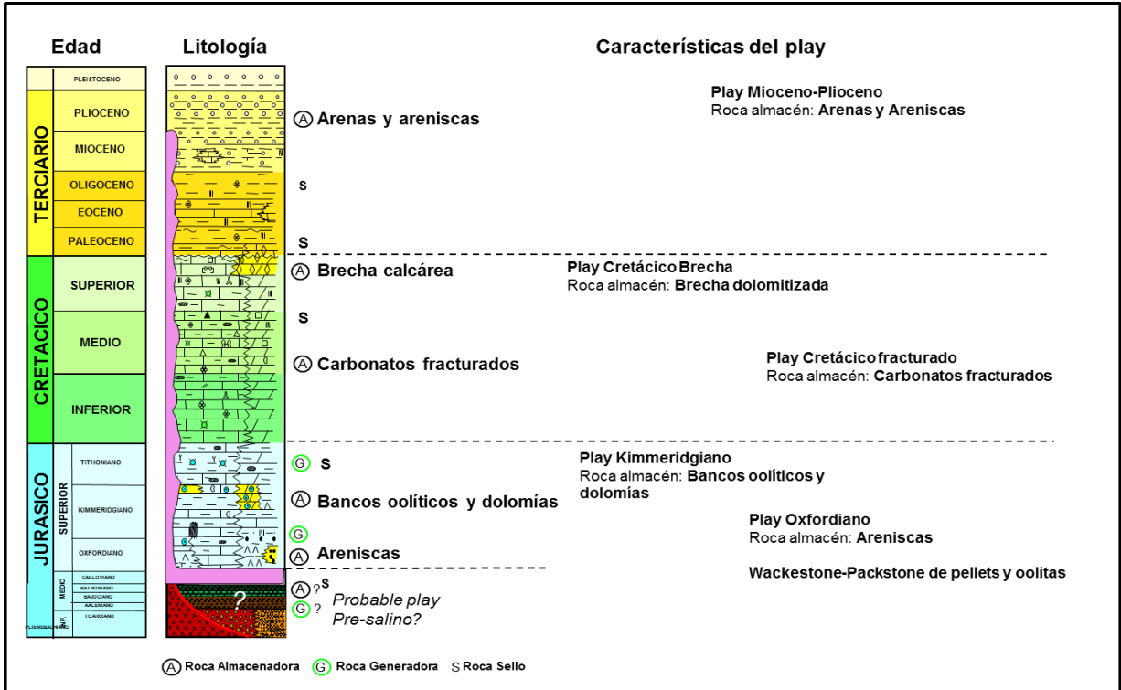
Figura 3.3. Modelo estratigráfico para las Op1 y Op2. (PEMEX, 2012).
