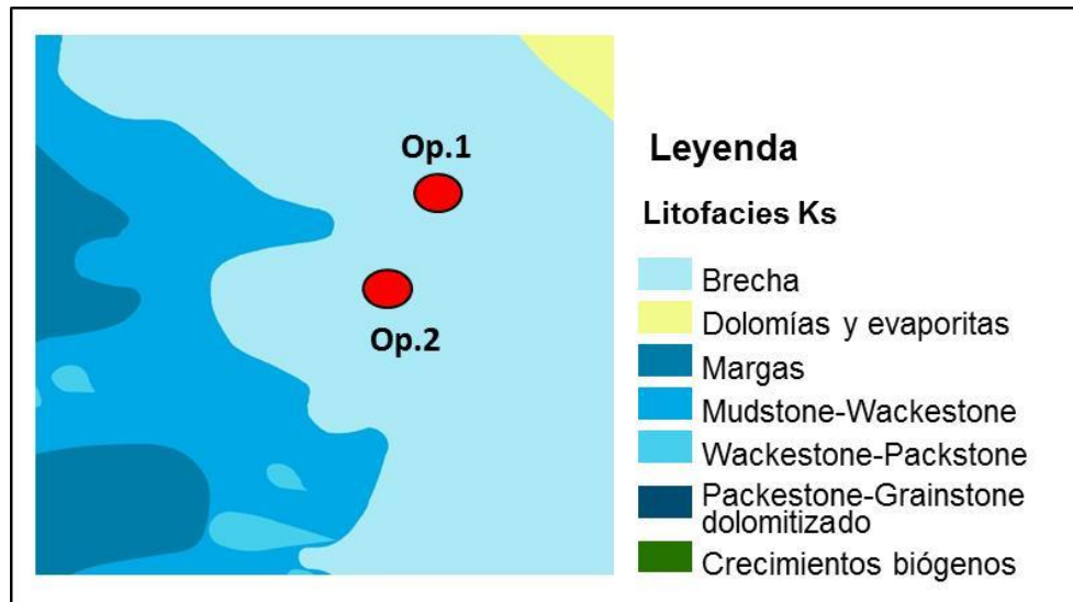
Figura 3.8. Mapa de distribución de Litofacies del Cretácico Superior. (PEMEX, 2013).
