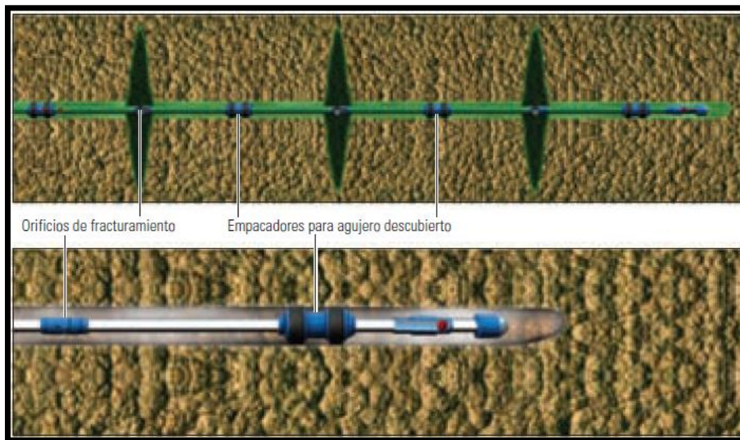
Figura 4.15. Sistema Permanente con Orificios de Fracturamiento. Recuperado de [ El tratamiento correcto para el yacimiento correcto . Bader al-Matar, Byung O. Lee, et al. (2008).]
