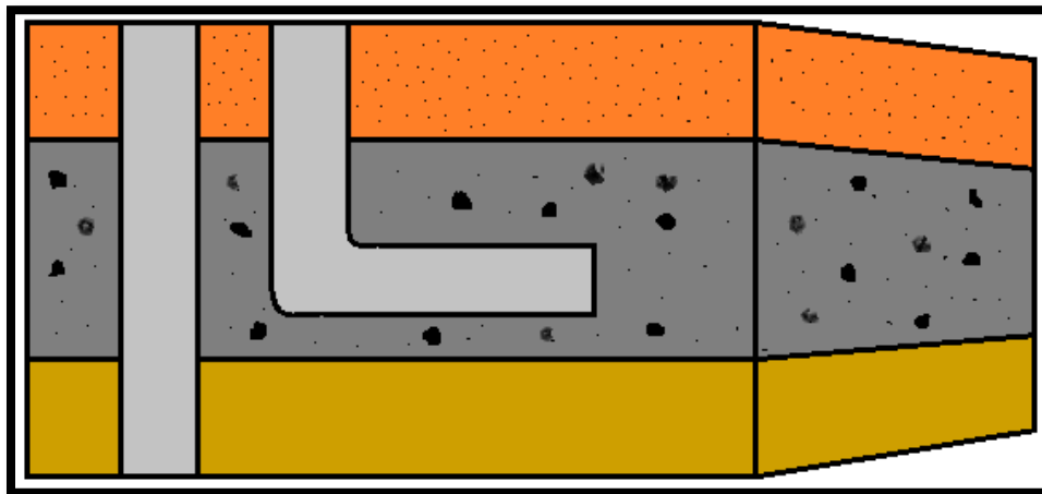
Figura 1.5. Formaciones de Baja Permeabilidad. Recuperado de [Terminación de pozos petroleros Hernández Tapia R. (1991). UNAM, Facultad de Ingeniería]
