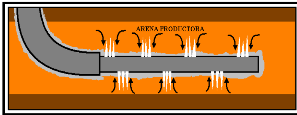
Figura 1.11. Terminación con liner cementado y cañoneado. Recuperado de [Pozos horizontales, diseño de pozos, campo Socorro. Espinoza D. & Solano A.. (Diciembre 2005).]
