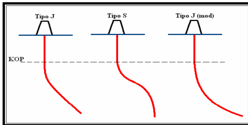
Figura 1.8. Tipos de pozos direccionales. Recuperado de [Pozos horizontales, diseño de pozos, campo Socorro. Espinoza D. & Solano A. (Diciembre 2005).]
