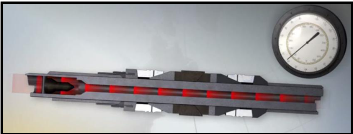
Figura 4.5. Contraflujo Proppet style frac plug. Recuperado de [http://www.youtube.com/watch?v=oPgZnZqp87k]
