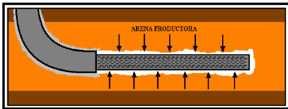
Figura 1.10 Terminación con liner ranurado No cementado. Recuperado de [Pozos horizontales, diseño de pozos, campo Socorro. Espinoza D. & Solano A.. (Diciembre 2005).]
