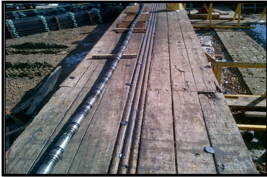
Figura 5.12. Recuperación de arreglo de camisas y tapones. Recuperado de [Multizone isolation system. (2013) Surestack]
