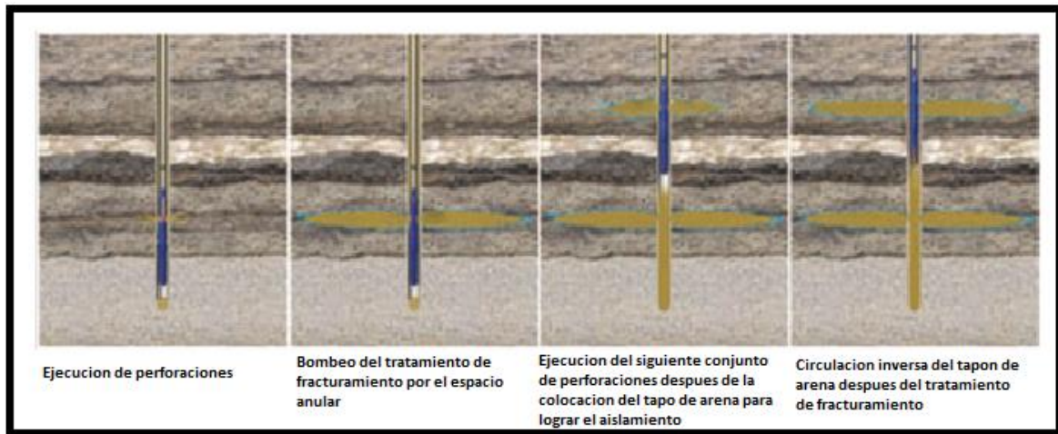
Figura 4.7. Sistema de disparos abrasivos. Recuerdo de [El tratamiento correcto para el yacimiento correcto. Bader al-Matar, Byung O. Lee, et al. (2008).]
