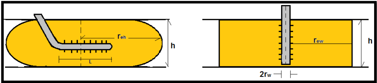
Figura 2.9. Esquema del radio de drenaje en un pozo horizontal. Recuperado de [Terminación de pozos petroleros. UNAM, Facultad de Ingeniería (1991)].
