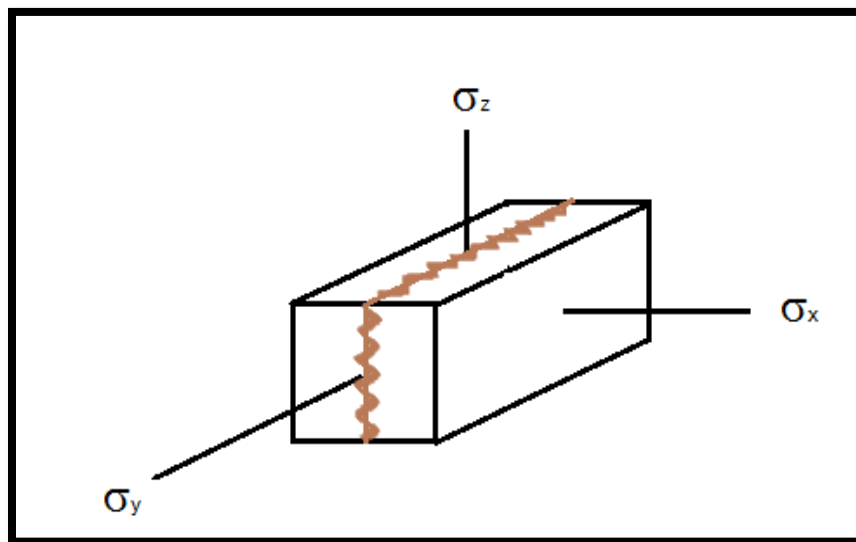
Figura 3.9. Fractura perpendicular en la dirección del menor esfuerzo de la roca. Recuperado de [Hydraulic fracturing. G.C. Howard, Society of petroleum engineers of AIME. (1970)]
