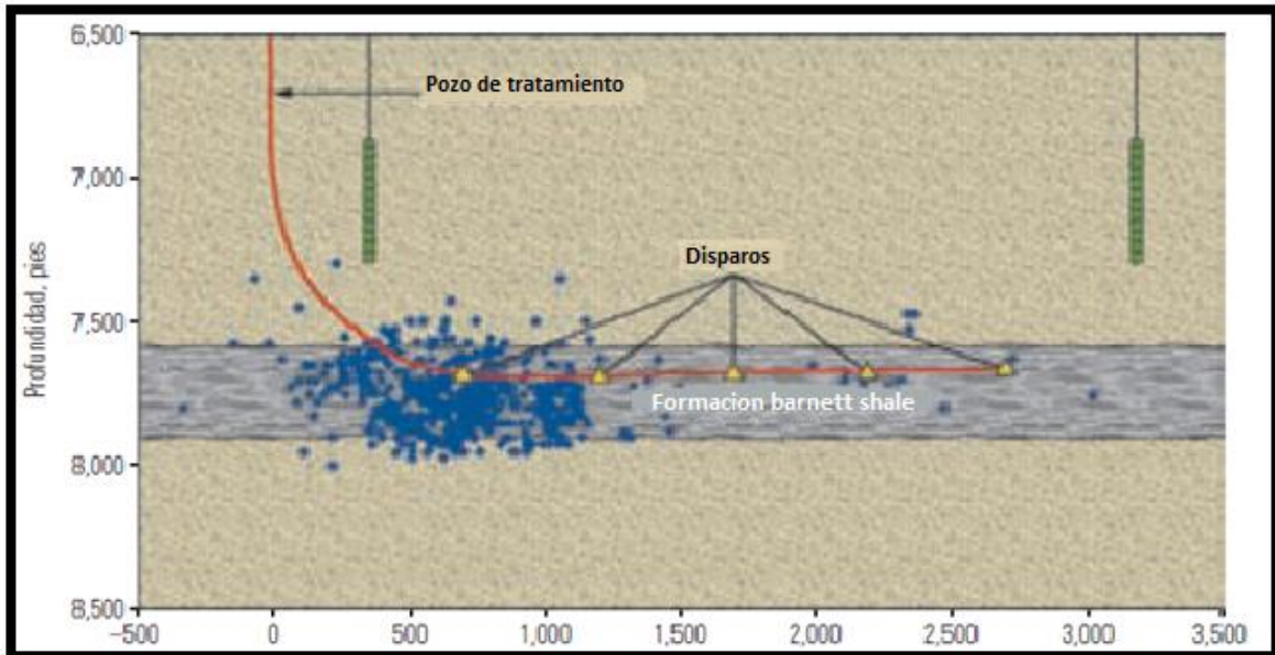
Figura 4.2. Fracturamiento de pozo horizontal terminado en agujero descubierto. Recuperado de [El tratamiento correcto para el yacimiento correcto. Bader al-Matar, Byung O. Lee, et al. (2008).]
