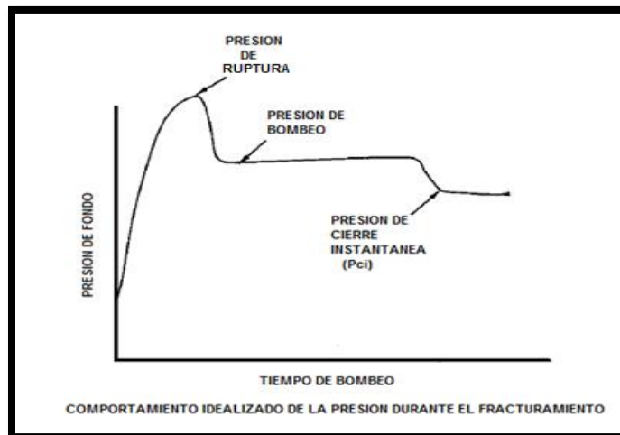
Figura 3.4 Comportamiento de la presión durante el fracturamiento. Recuperado de [ Oil well stimulation . Schechter S. R. (1992).]
