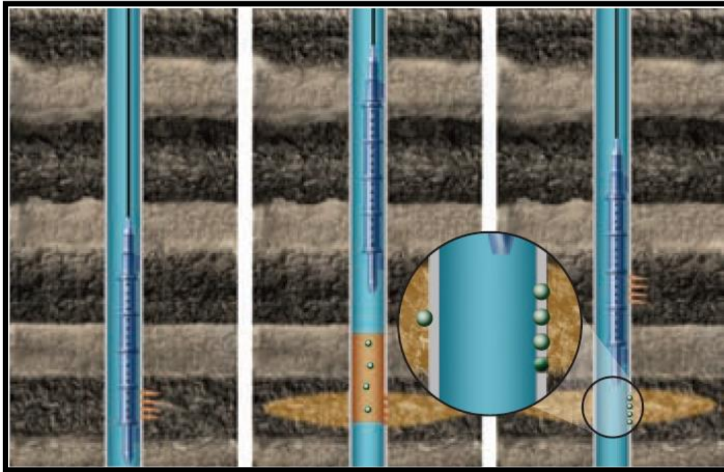
Figura 4.8. Operación del sistema de estimulación con esferas selladoras. Recuperado de [ El tratamiento correcto para el yacimiento correcto . Bader al-Matar, Byung O. Lee, et al. (2008).]
