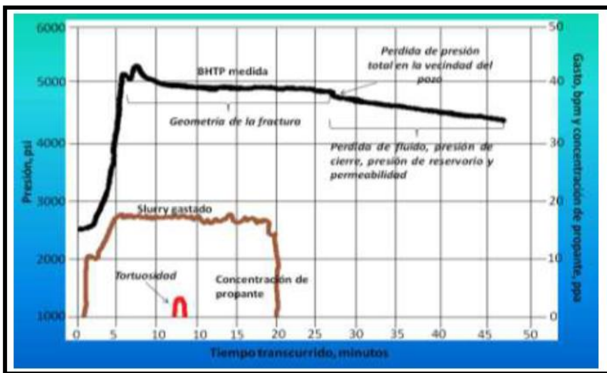
Figura 3.3 Ejemplo del empleo de una gráfica minifrac. Recuperado de [Backer Hughes (2013)]
