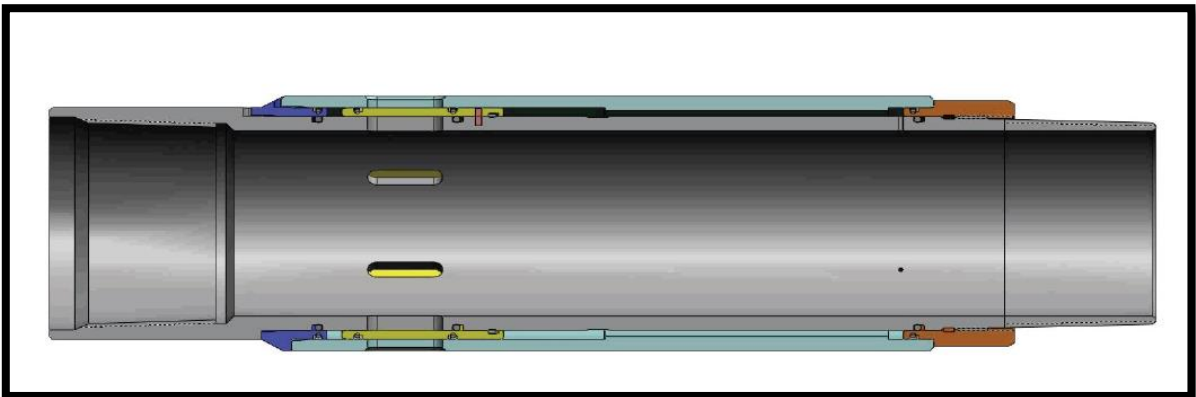
Figura 4.10. Ensamble de Fracturamiento de camisas deslizables en la tubería flexible. Recuperado de [Cased-Hole Multistage Fracturing: A new Coiled-tubing-enabled completion. Ravensberg J. & Baker Hughes. (2011).]
