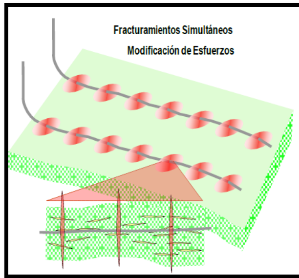
Figura 4.19. Fracturamientos Simultáneos modificación de esfuerzos. Recuperado de [ Retos y avances en el desarrollo y operación de un yacimiento no convencional, "Chicontepepec". Narváez A.. (2012).]
