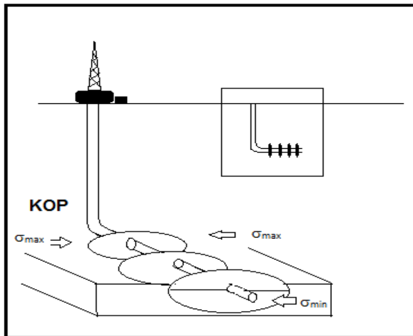
Figura 3.1 Fracturas verticales a la sección horizontal, perpendiculares al esfuerzo mínimo. Recuperado de [Terminación de pozos petroleros. UNAM, Facultad de Ingeniería (1991)]
