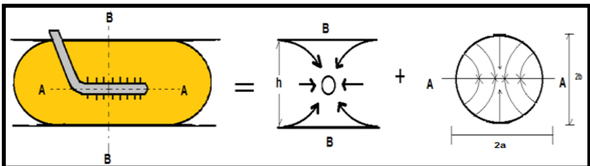
Figura 2.10. Problema de flujo tridimensional. Recuperado de [Terminación de pozos petroleros. UNAM, Facultad de Ingeniería (1991)]
