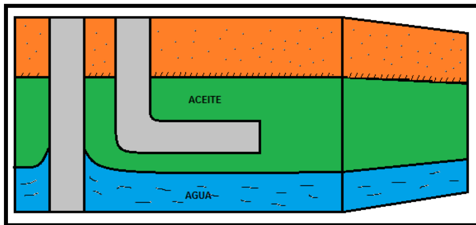
Figura 1.1 Conificación de agua. Recuperado de [Terminación de pozos petroleros Hernández Tapia R. (1991). UNAM, Facultad de Ingeniería ]
