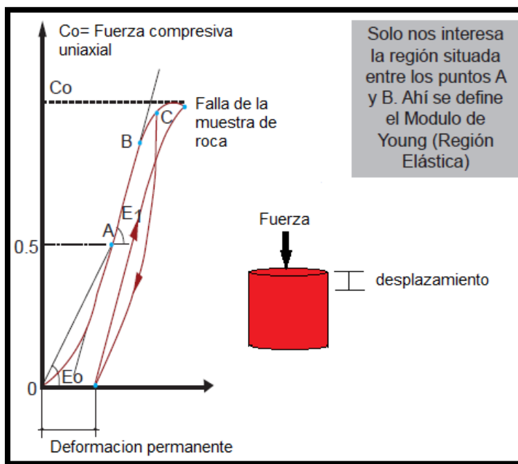
Figura 3.10 Representación de la prueba de compresión realizada a una muestra de roca. Recuperado de [Guía de diseño para fracturamientos hidráulicos PEMEX, UPMP. (2008)]
