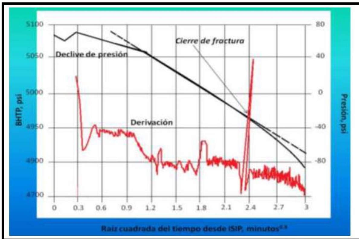
Figura 3.5 Ejemplo de una grafica minifrac del declive de presión y la raíz cuadrada del Tiempo. Recuperado de [Backer Hughes (2013)]
