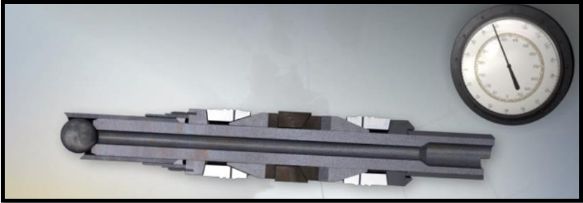
Figura 4.6. Ball Frac Plug. Recuperado de [http://www.youtube.com/watch?v=oPgZnZqp87k]
