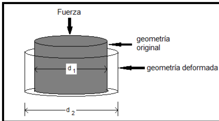
Figura 3.11 Representación de la relación de Poisson. Recuperado de [Hydraulic fracturing. G.C. Howard, Society of petroleum engineers of AIME. (1970)]
