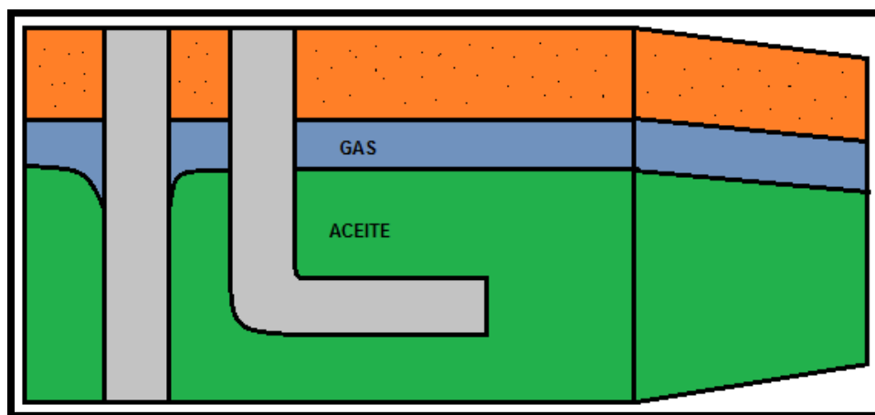
Figura 1.2. Conificación de gas. Recuperado de [Terminación de pozos petroleros Hernández Tapia R.. (1991). UNAM, Facultad de Ingeniería]
