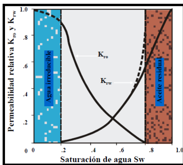
Figura 2.3. Permeabilidad relativa. Recuperado de [Taller: estimulación de pozos. Villahermosa tabasco. (2011).]
