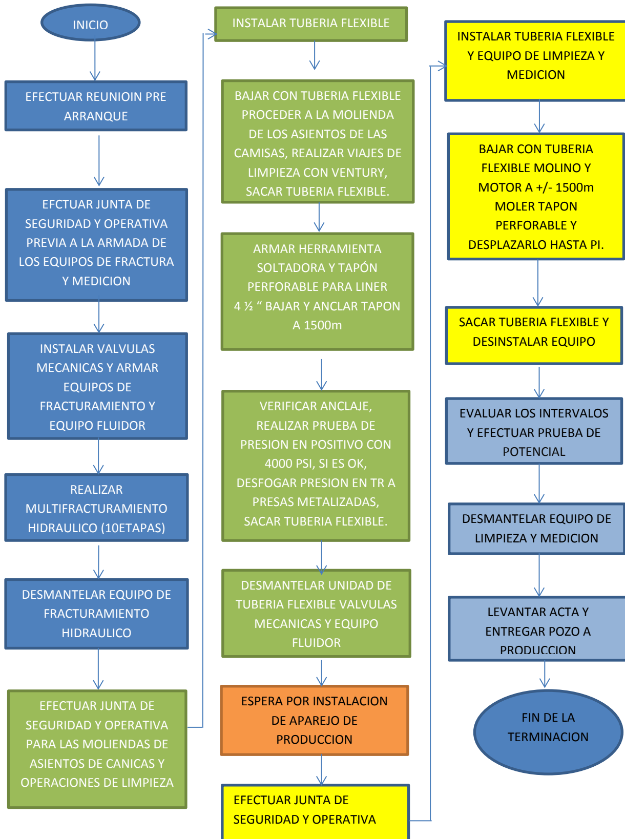
Figura 5.9. Flujo de Programa de Trabajo para los Trabajos de Terminación. Recuperado de [PEMEX. (2013). Programa de terminación Humapa .
