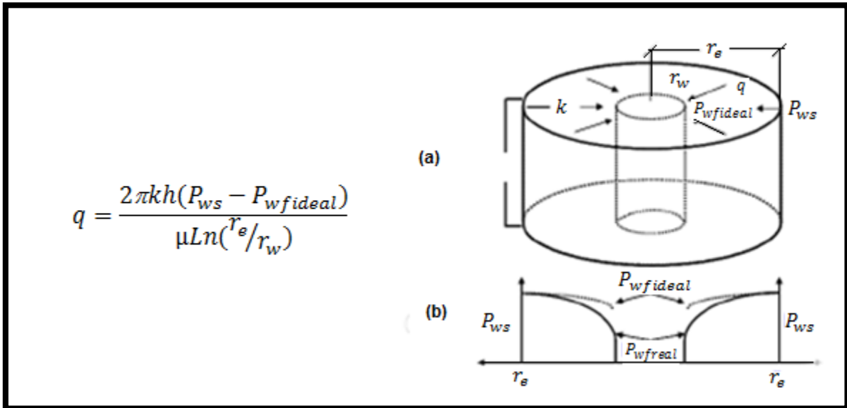
Figura 2.2 Condiciones esquemáticas del flujo Darcy en un yacimiento radial circulado. Recuperado [Taller: estimulación de pozos. Villahermosa tabasco. (2011).]
