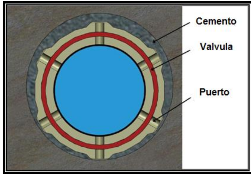
Figura 4.18. Localización de los puertos del ensamble de fracturamiento. Recupearado de [Cased-Hole Multistage Fracturing: A new Coiled-tubing-enable completion. Ravensberg J. & baker hughs. (2011).]
