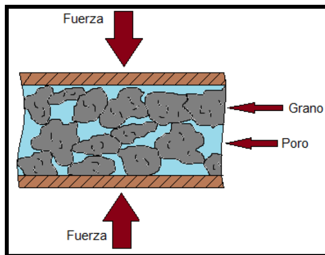
Figura 3.7. Carga por presión de poro. Recuperado de [Hydraulic fracturing. G.C. Howard, Society of petroleum engineers of AIME. (1970)]
