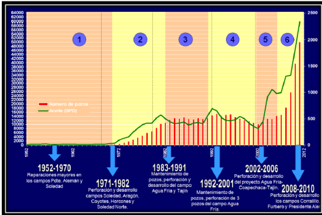
Figura 5.3. Comportamiento histórico de producción del Paleocanal de Chicontepec. Recuperado de [Terminación con Multifracturas en Pozos de Máximo Contacto con el yacimiento Estrada Aguilar E. (2012)].
