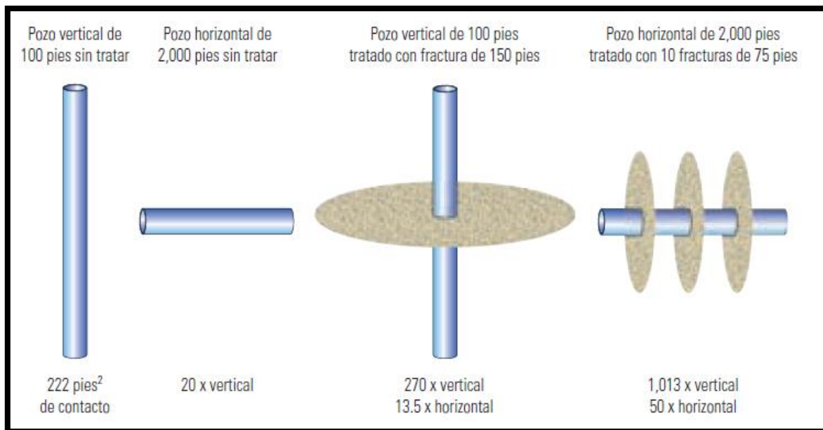
Fig. 4.1 Mejoramiento del contacto con la formación en pozos verticales y horizontales. Recuperado de [ El tratamiento correcto para el yacimiento correcto. Bader al-Matar, Byung O. Lee, et al. (2008).]
