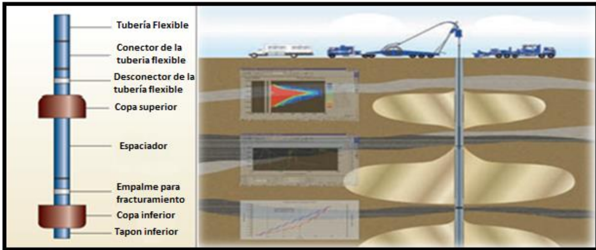
Figura 4.9. Arreglo de tubería flexible con empacadores. Recuperado de [El tratamiento correcto para el yacimiento correcto. Bader al-Matar, Byung O. Lee, et al. (2008).]
