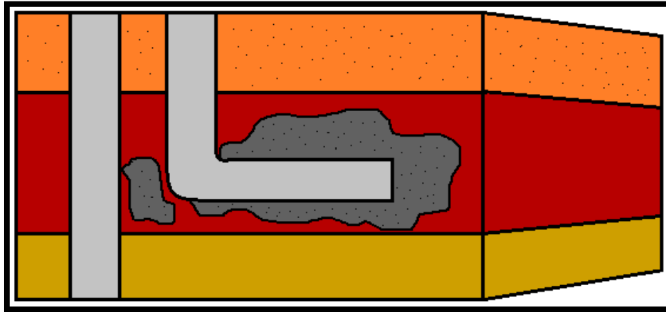
Figura 1.4. Formaciones Irregulares. Recuperado de [Terminación de pozos petroleros Hernández Tapia R.. (1991). UNAM, Facultad de Ingeniería]
