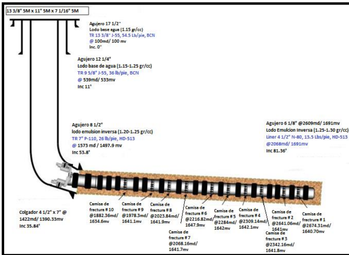
Figura 5.8.Estado mecánico de pozo Humapa. Recuperado de [Programa de terminación Humapa,PEMEX. (2013).]
