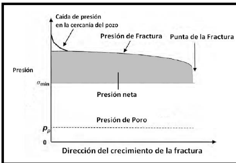
Figura 3.6 Perfil de presión en una fractura apuntalada. Recuperado de [Oil well stimulation. Schechter S. R. (1992).]
