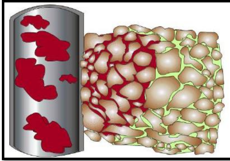
Figura 2.6. Daño por bloqueo de aceite. Recuperado de [Taller: estimulación de pozos. Villahermosa tabasco. (2011).]
