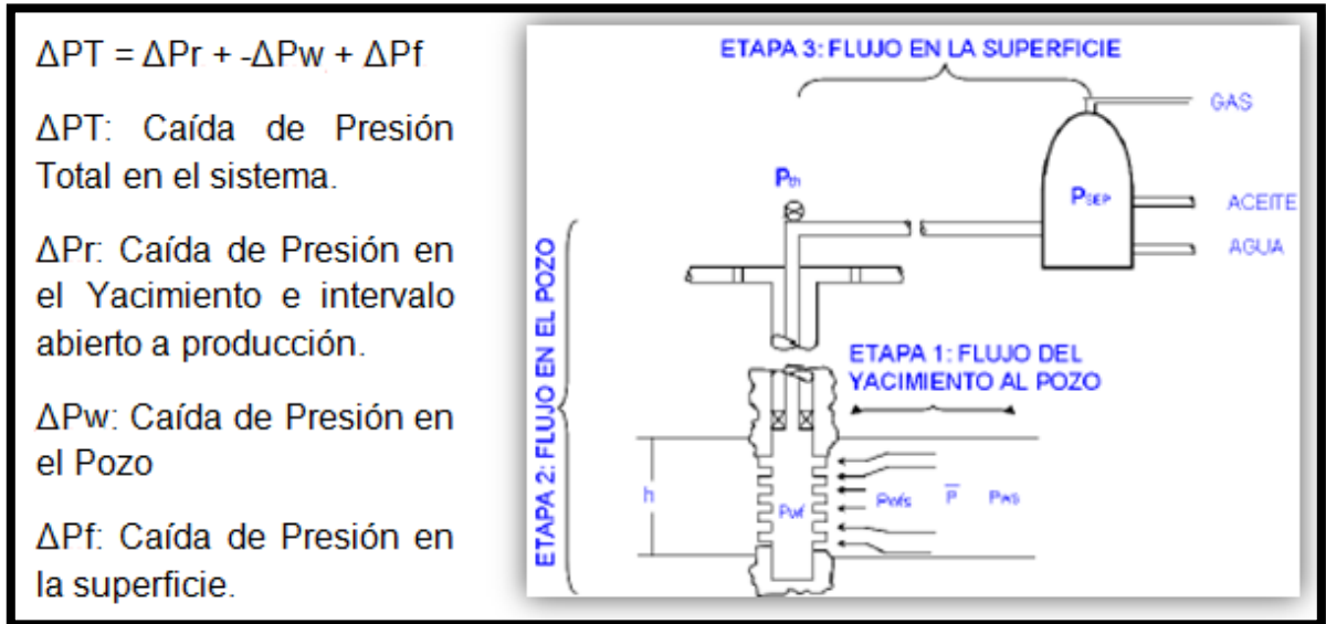
Figura 2.1. Esquema del Sistema Integral de Producción. Recuperado de [Taller: estimulación de pozos. Villahermosa tabasco (2011)]
