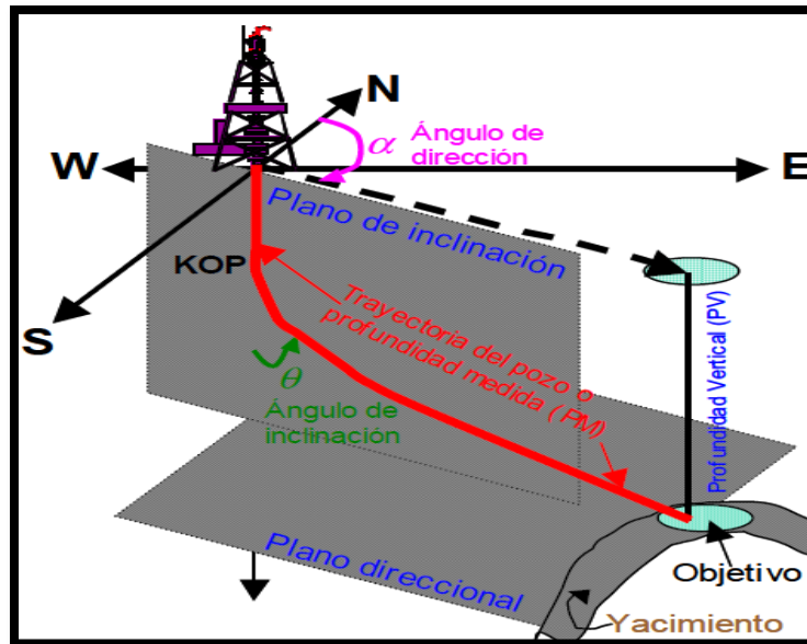
Figura 1.7. Componentes de un pozo direccional. Recuperado de [Pozos horizontales, diseño de pozos, campo Socorro. Espinoza D. & Solano A. (Diciembre 2005).]
