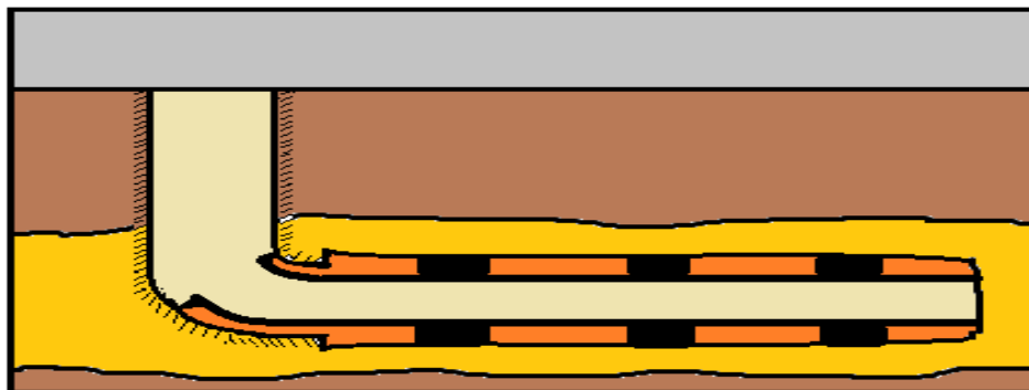
Figura 1.12. Terminación Con TR, Empacadores Externos Recuperado de [ Terminación de pozos petroleros Hernández Tapia R.. (1991). UNAM, Facultad de Ingeniería]
