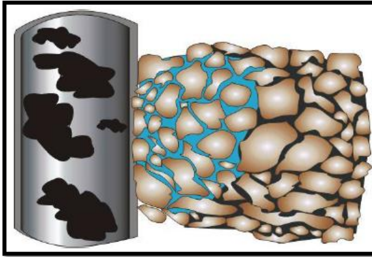
Figura 2.5. Daño por bloqueo de agua. Recuperado de [Taller: estimulación de pozos. Villahermosa tabasco. (2011).]
