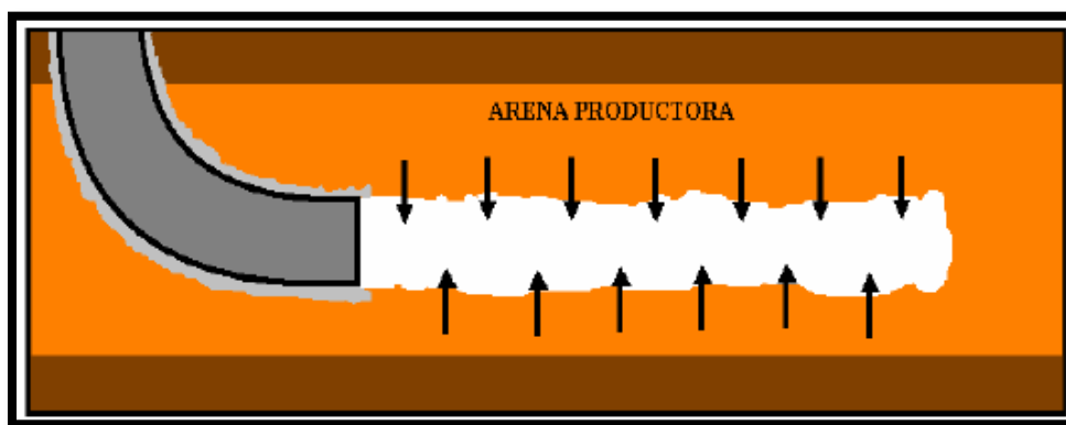
Figura 1.9 Terminación a agujero abierto. Recuperado de [Pozos horizontales, diseño de pozos, campo Socorro. Espinoza D. & Solano A.. (Diciembre 2005).]
