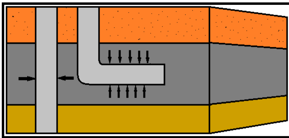
Figura 1.6. Recuperación Mejorada de Aceite. Recuperado de [Terminación de pozos petroleros Hernández Tapia R. (1991). UNAM, Facultad de Ingeniería]
