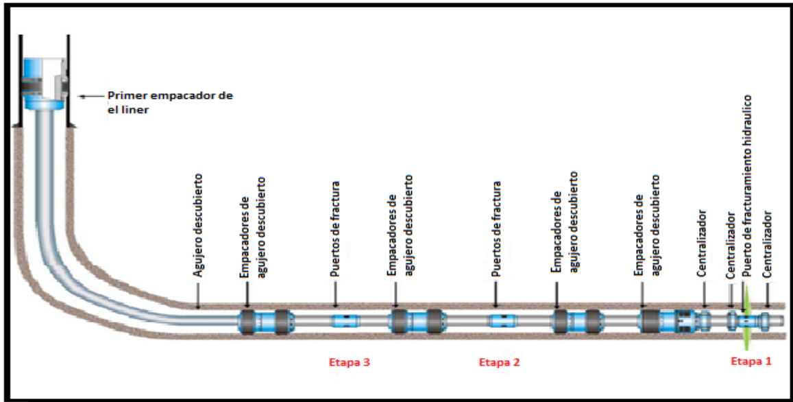
Figura 4.16. Estado mecánico de sistema permanente de fracturamiento. Recuperado de [ Effective open hole horizontal completion System for multistage fracturing and stimulation Athans J. & Packers plus energy Services. (2008).]
