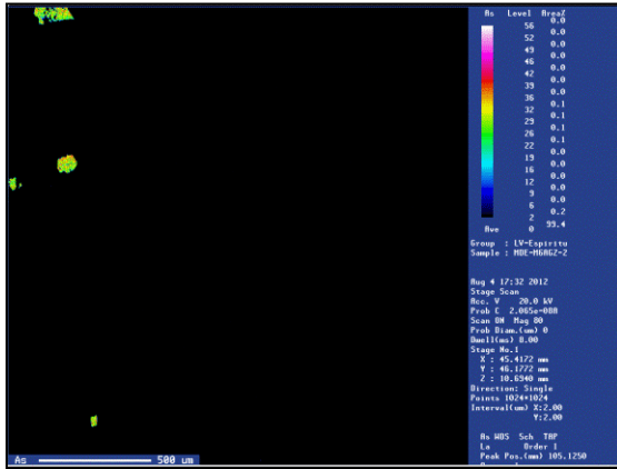
Figura 16. Mapeo de distribución elemental de Arsenico, aquí se puede distinguir fácilmente a la arsenopirita (Apy), ya que son cristales euhedrales y subhedrales de buen tamaño.
