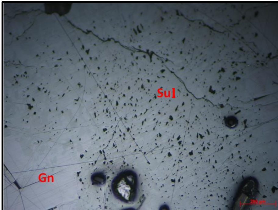
Foto-micrografía 1. Campo de la muestra esp-zim13.océano de galena (gn) con reemplazamiento de sulfosales (sul) en forma de islas. Tomada a microscopio mineralográfico con luz paralela.
