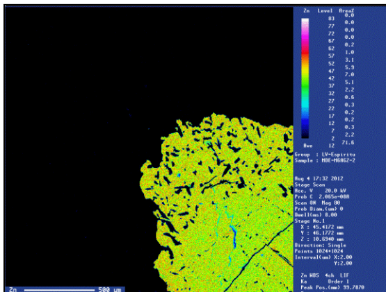
Figura 18. Mapeo de distribución elemental de Zinc, aquí es demasiado evidente que el Zn se encuentra solamente en un mineral, en este caso es esfalerita y se puede observar que la concentración de este elemento es alta.
