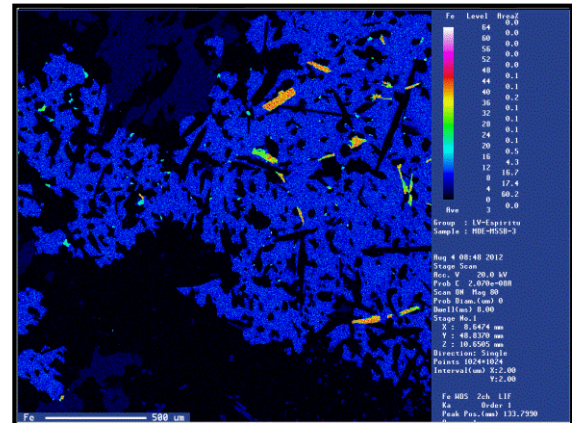
Figura 26. Mapeo de distribución elemental de hierro, nuevamente aquí se puede observar que la esfalerita puede ser catalogada como marmatita o esfalerita ferrifera. También se pueden observar algunos cristales de pirrotita, fácilmente identificables por ser las zonas con mayor concentración de este elemento.
