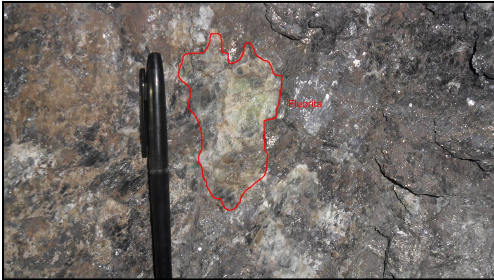
Figura 12. Parche de fluorita en el nivel -150
