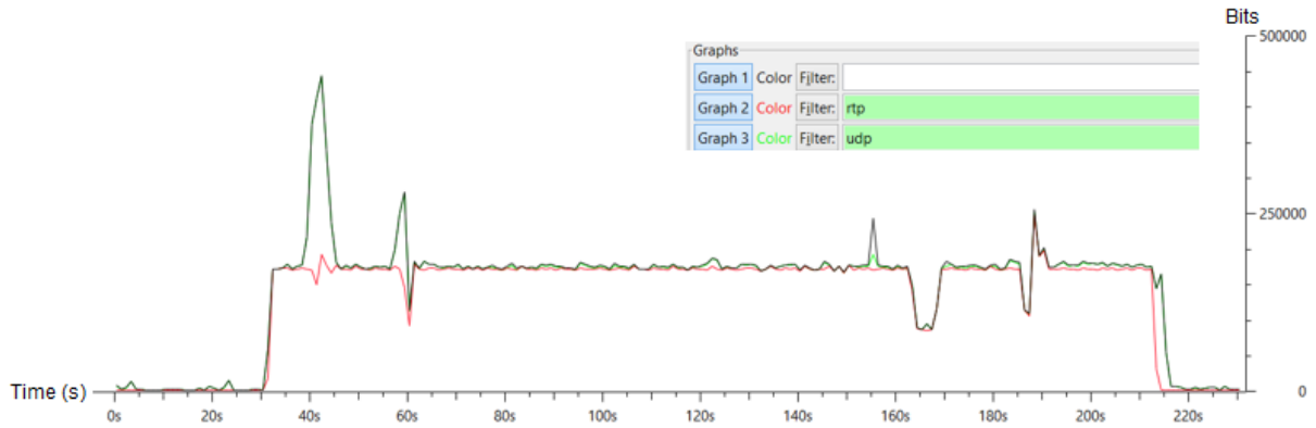
Figura 5.48. Utilización de llamada de VoIP en AP 1 en escenario 6.
