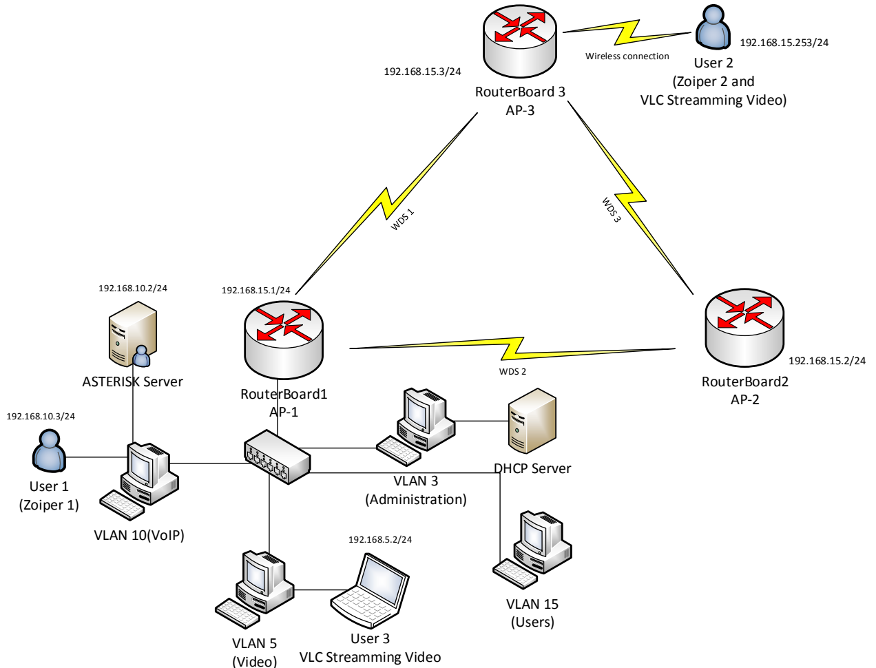
Figura 4.1. Diagrama general de implementación de red inalámbrica mesh parcial con VLAN's.
