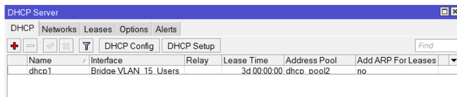
Figura 4.4. Servidor DHCP.
