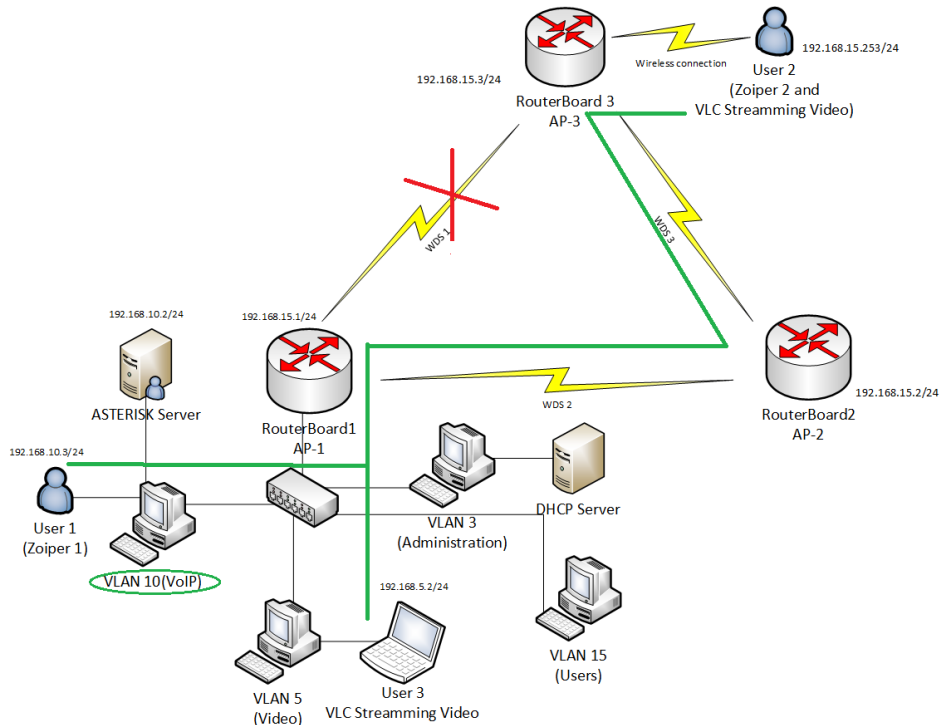
Figura 5.10. Diagrama de la ruta del tráfico en escenario 2 con VLAN's.
