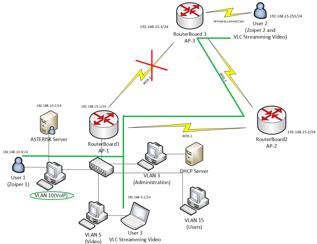
Figura 5.27. Diagrama de la ruta del tráfico en escenario 4 con VLAN's.
