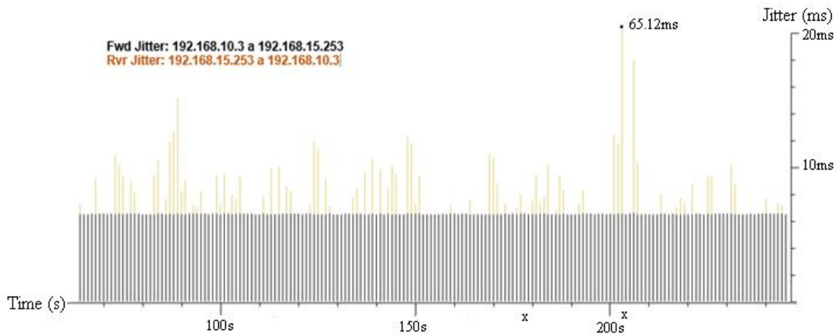
Figura 5.31. Jitter en escenario 4 con VLAN's.
