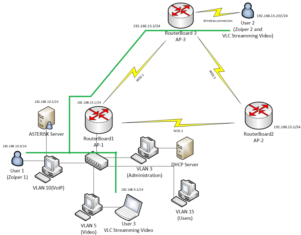
Figura 5.1. Diagrama de la ruta del tráfico en escenario 1 con VLAN's.
