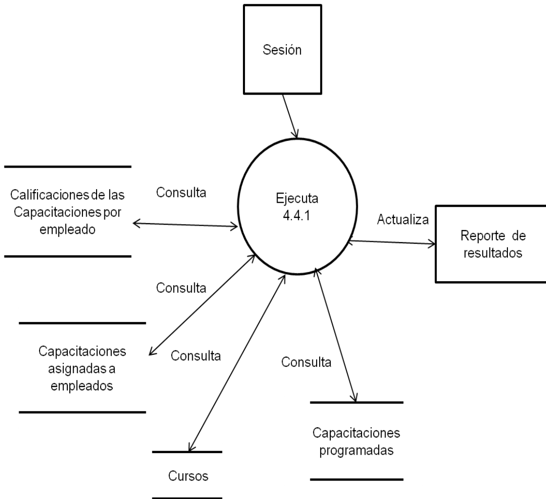
Figura 4.1.2.11 Diagrama del proceso Nivel 3, 4.4.1 Reportes de resultados de capacitación por cursos programados
