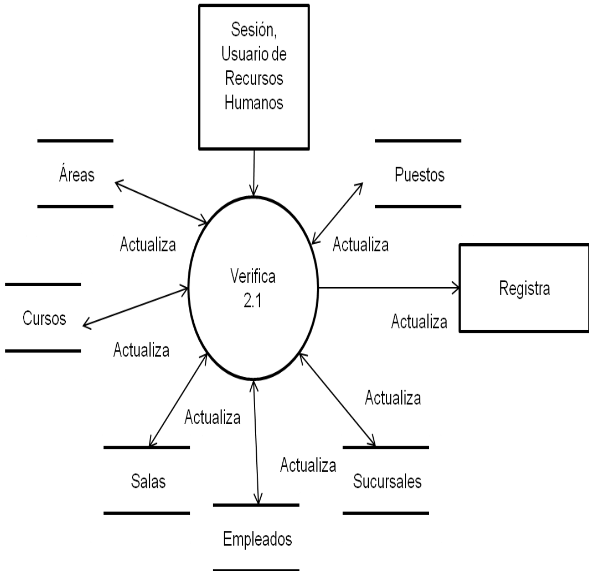
Figura 4.1.2.3 Diagrama del proceso Nivel 2, 2.1 Administración de recursos
