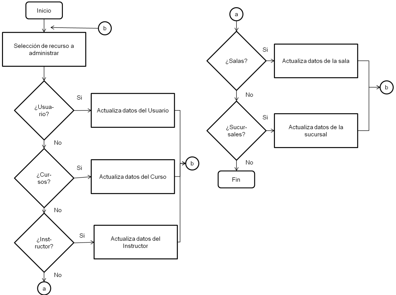
Figura 4.1.2.16 Diagrama de flujo de datos, 1.- Administración de recursos
