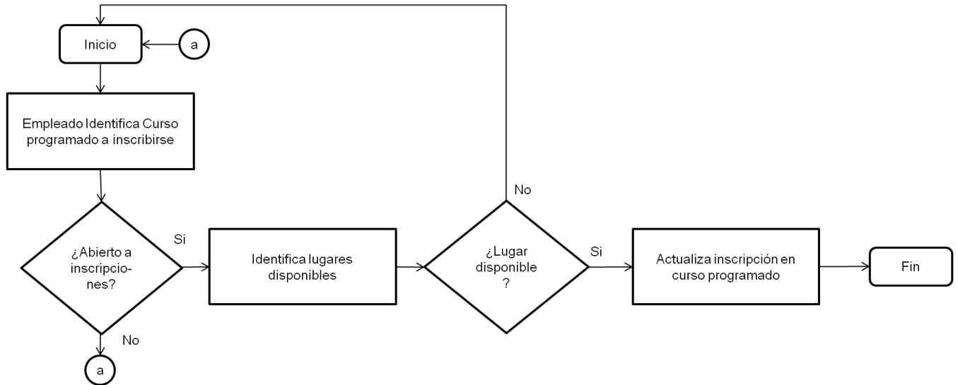
Figura 4.1.2.19 Diagrama de flujo de datos, 4.- Inscripciones
