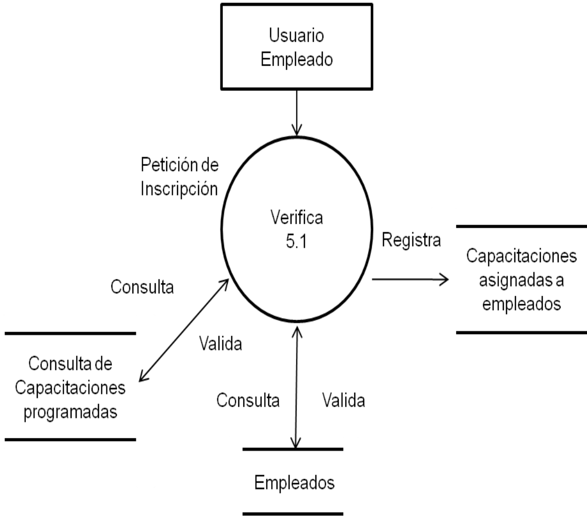
Figura 4.1.2.12 Diagrama del proceso Nivel 2, 5.1 Inscripciones
