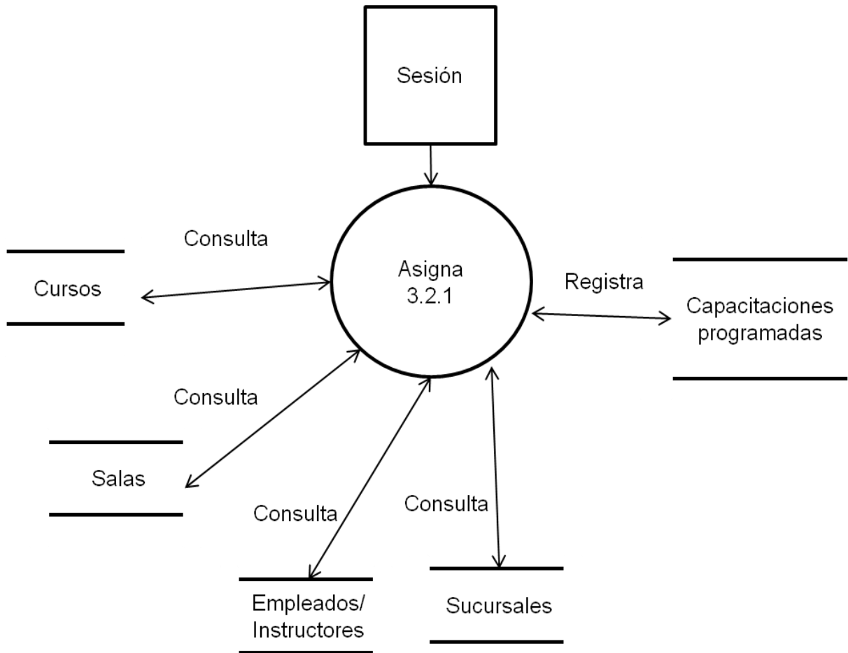
Figura 4.1.2.5 Diagrama del proceso Nivel 3, 3.2.1 Asignación de recursos
