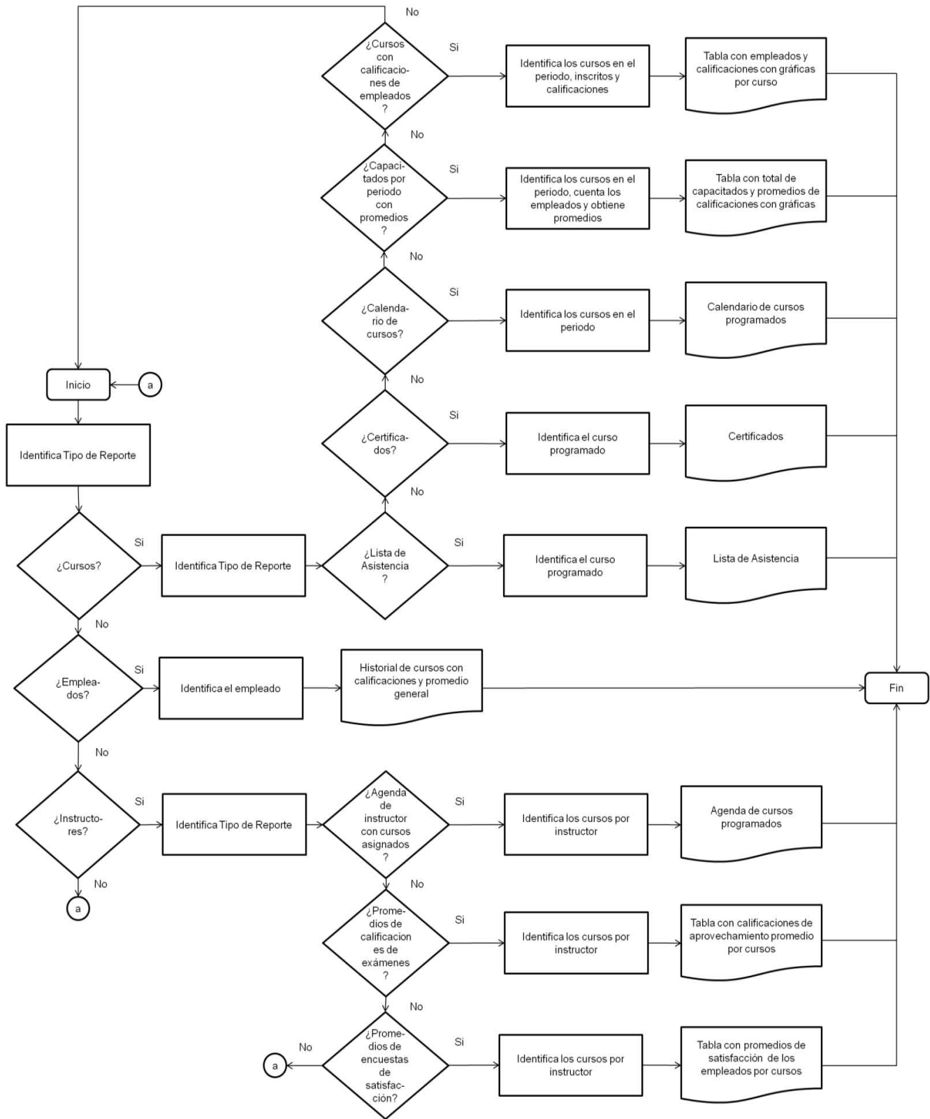
Figura 4.1.2.18 Diagrama de flujo de datos, 3.- Reportes supervisión
