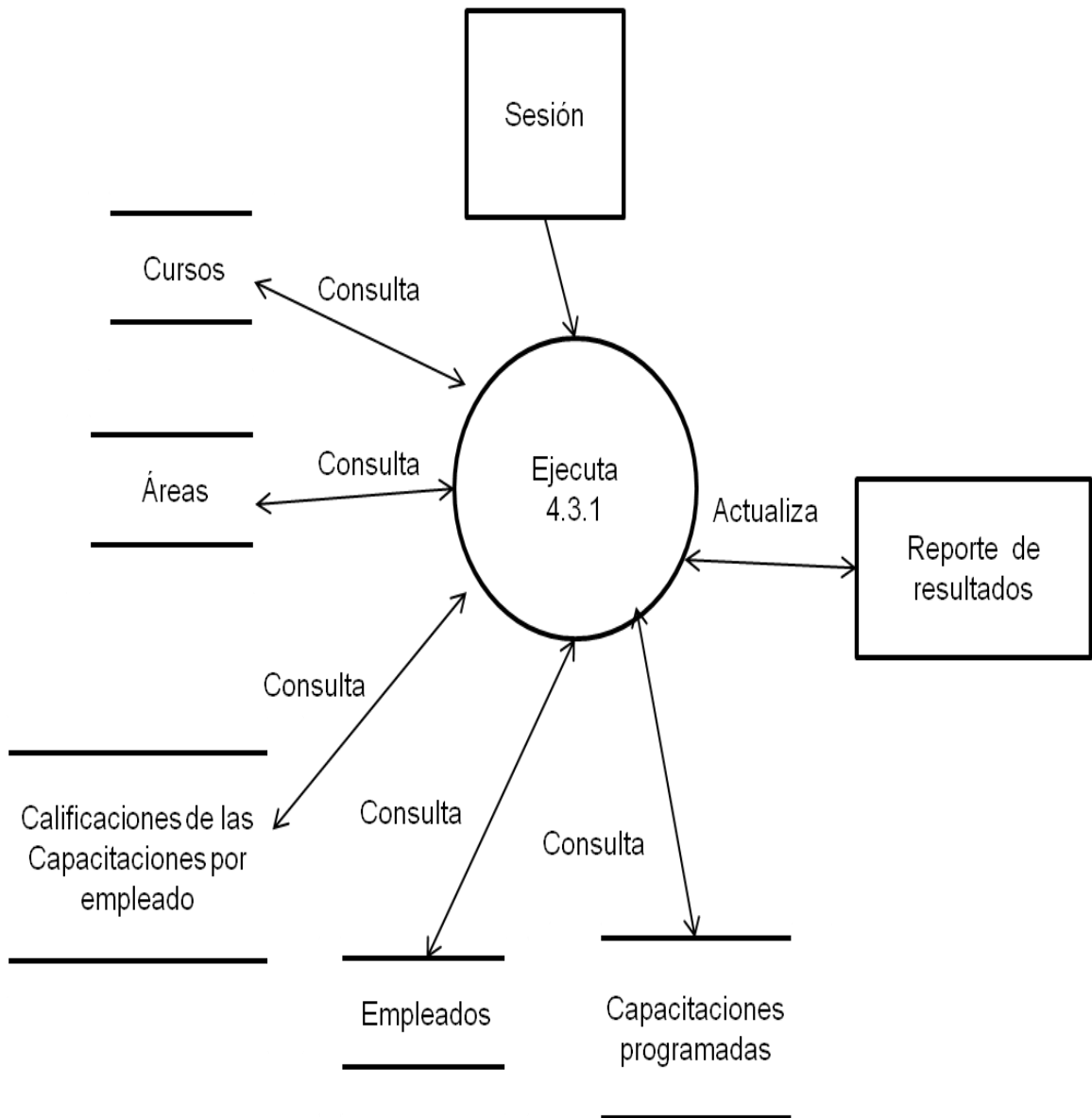
Figura 4.1.2.10 Diagrama del proceso Nivel 3, 4.3.1 Reportes de resultados de capacitación por área
