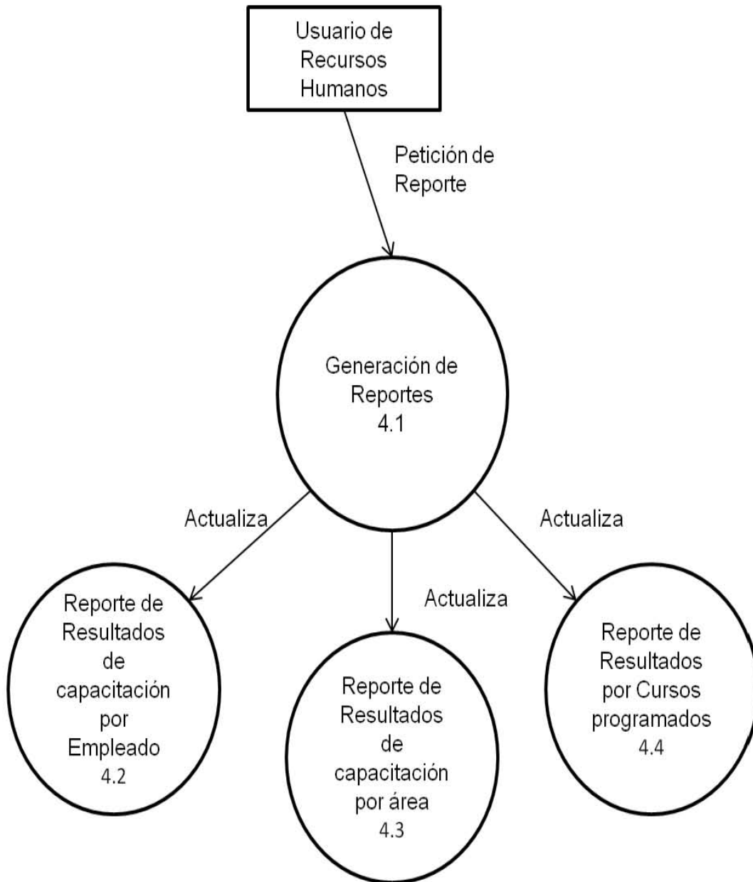
Figura 4.1.2.8 Diagrama del proceso Nivel 2, 4.1 Reportes supervisión
