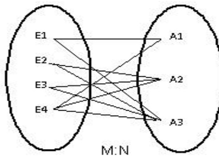
Figura 2.1.4 Relación muchos a muchos
