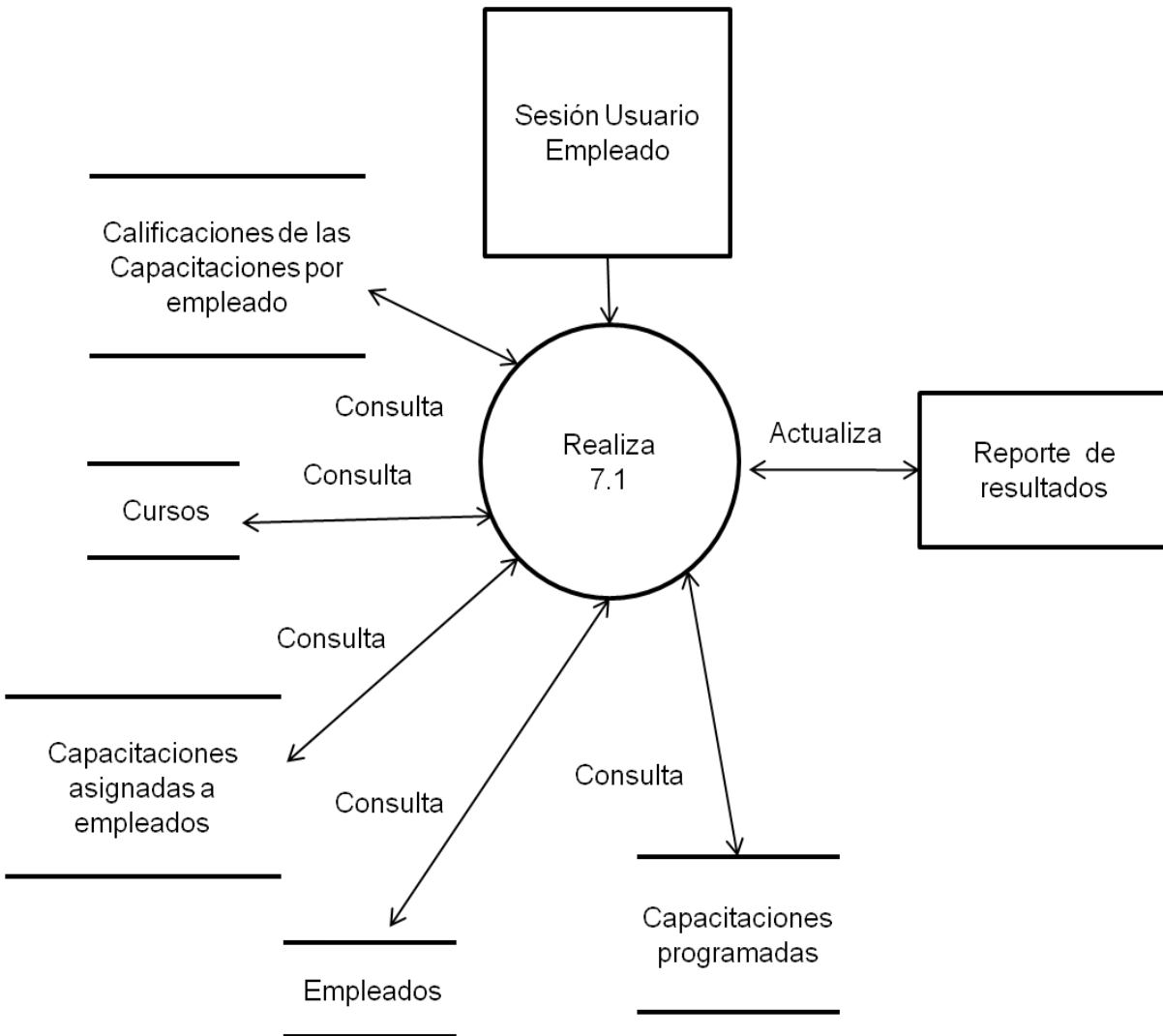
Figura 4.1.2.14 Diagrama del proceso Nivel 2, 7.1 Reportes de avances
