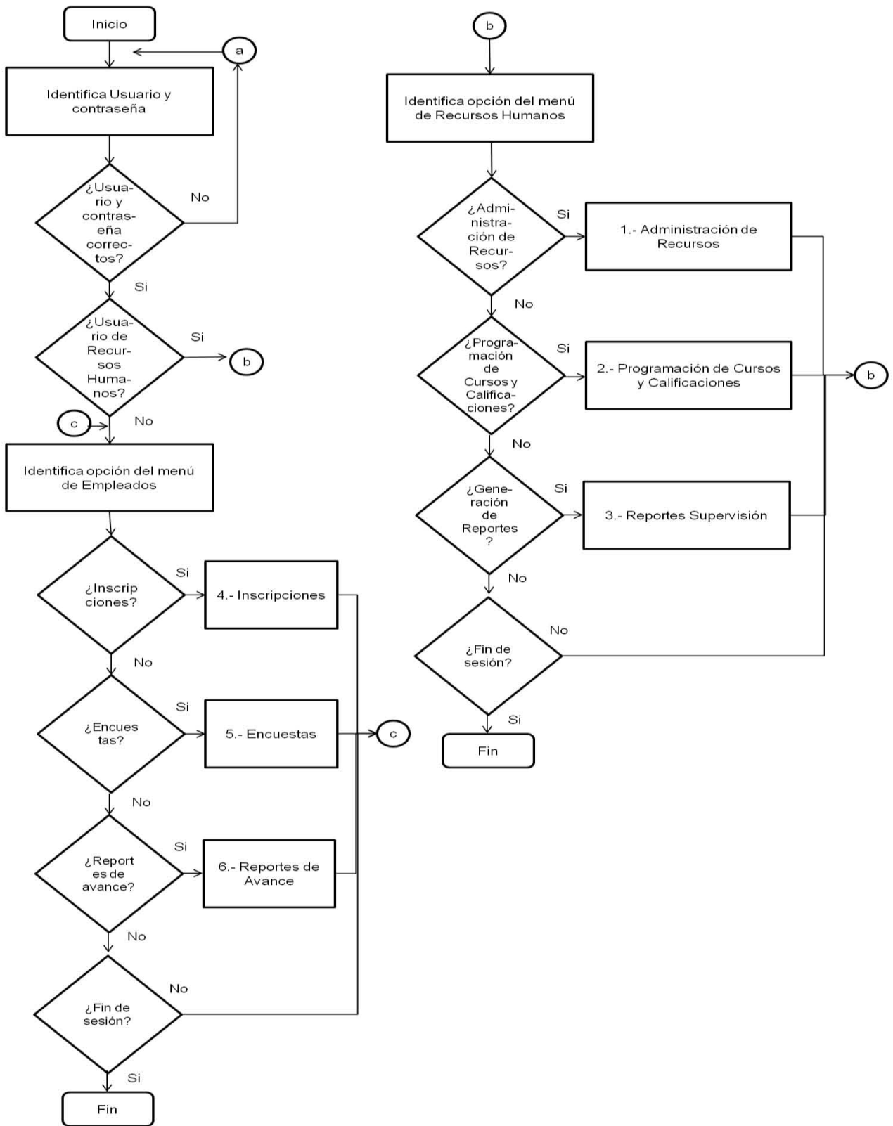
Figura 4.1.2.15 Diagrama de flujo de datos, Proceso general
