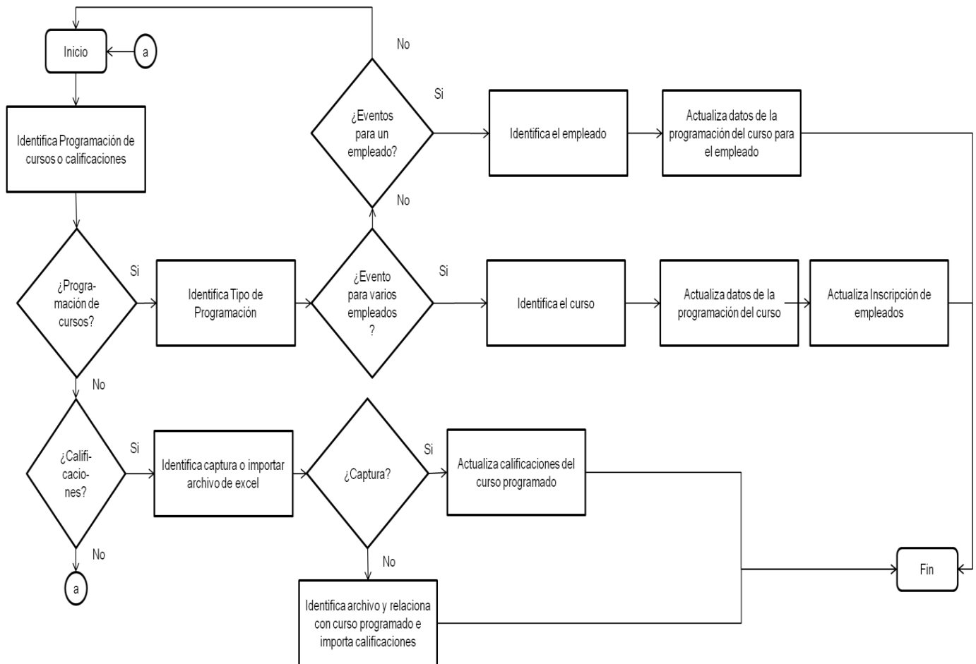
Figura 4.1.2.17 Diagrama de flujo de datos, 2.- Programación de cursos y calificaciones
