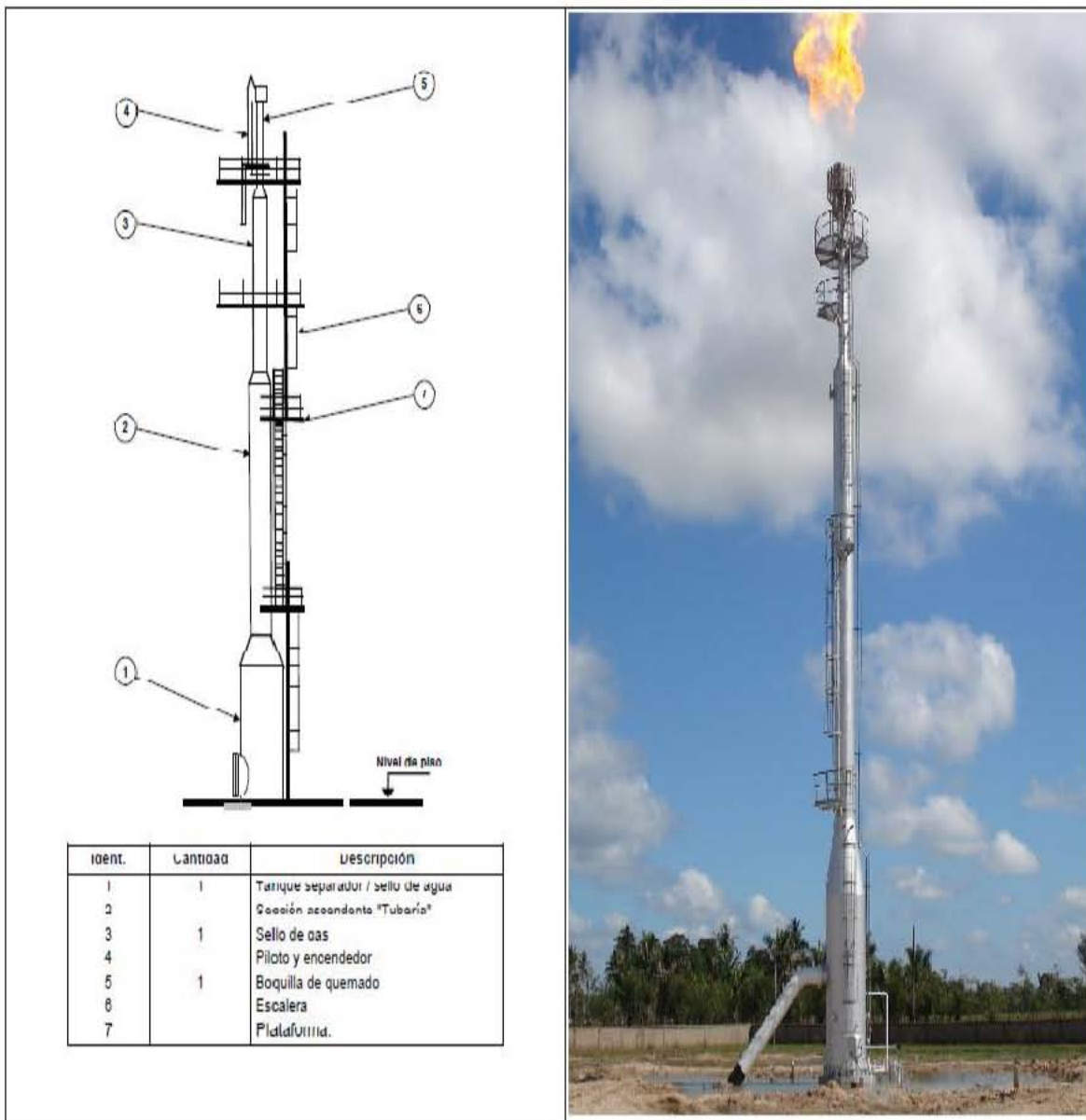
Figura 17. Quemador autosoportado
