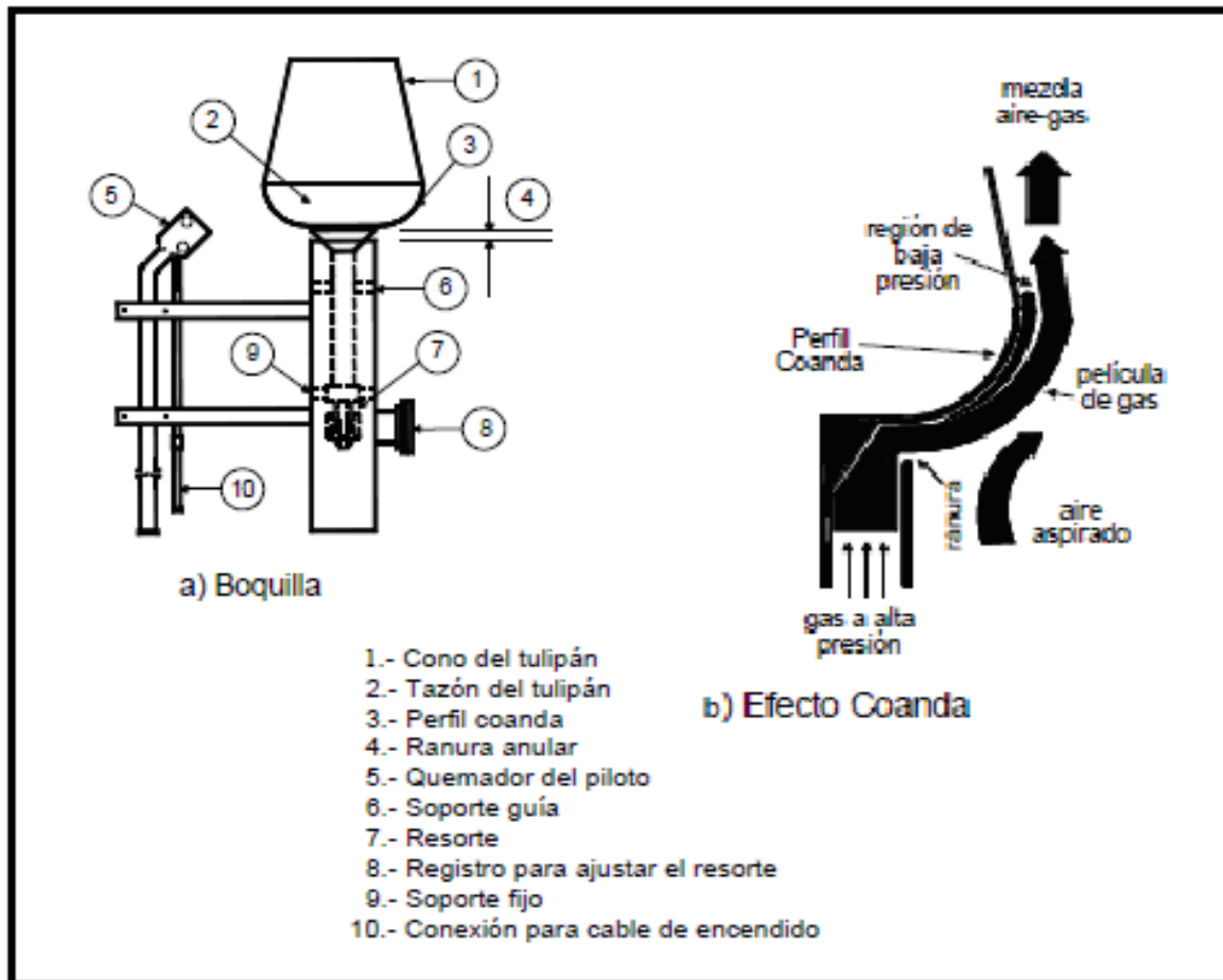
Figura 27. Boquilla de quemador tipo Coanda
