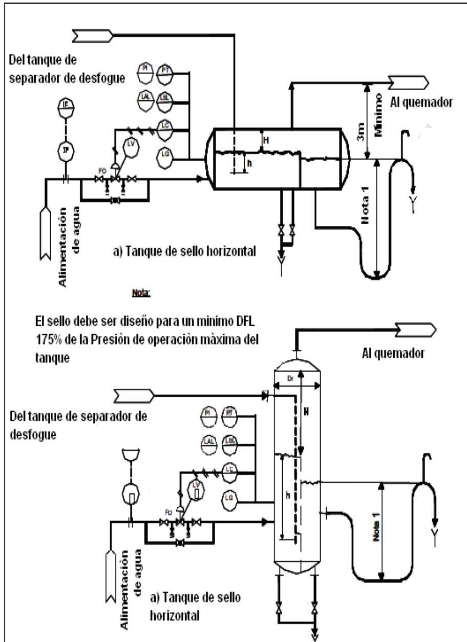
Figura 21. Sello líquido
