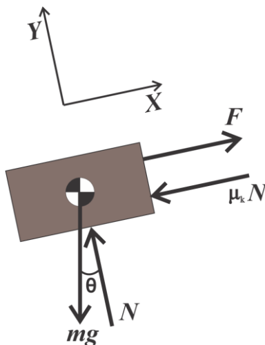
Figura 3.2 Diagrama de cuerpo libre.
