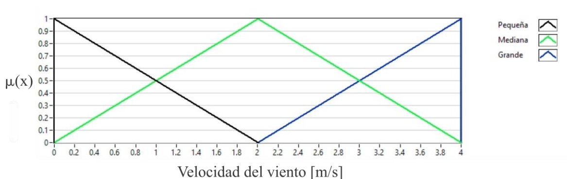
Figura 4.3 Variable difusa de velocidad del viento.
