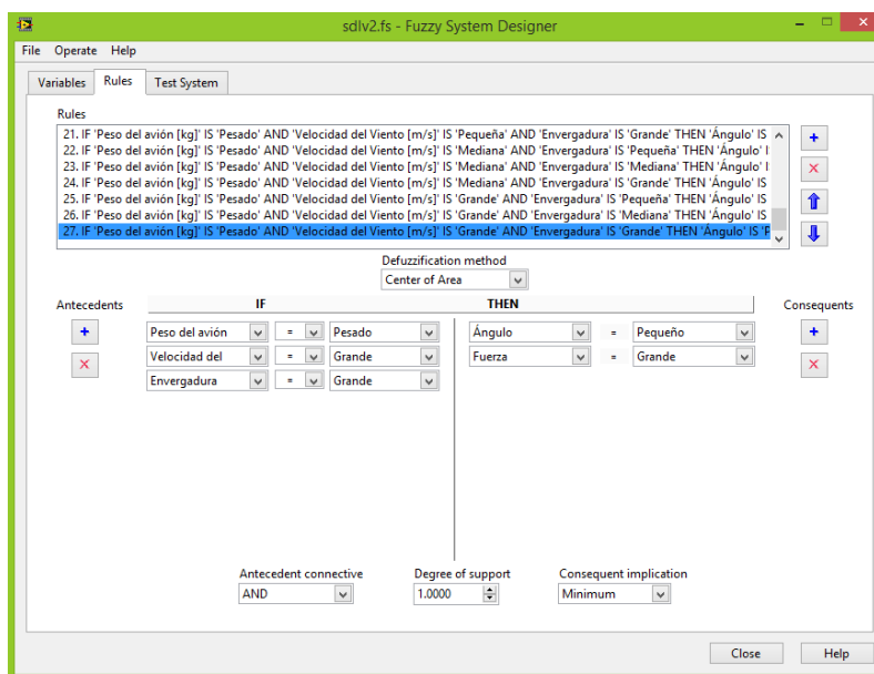
Figura IV.2 Reglas difusas
