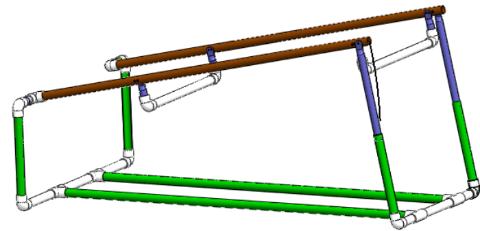
Figura 5.21 Lanzadera a 12°.
