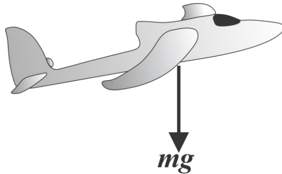
Figura 3.4 Diagrama de cuerpo libre del avión al momento de ser lanzado.
