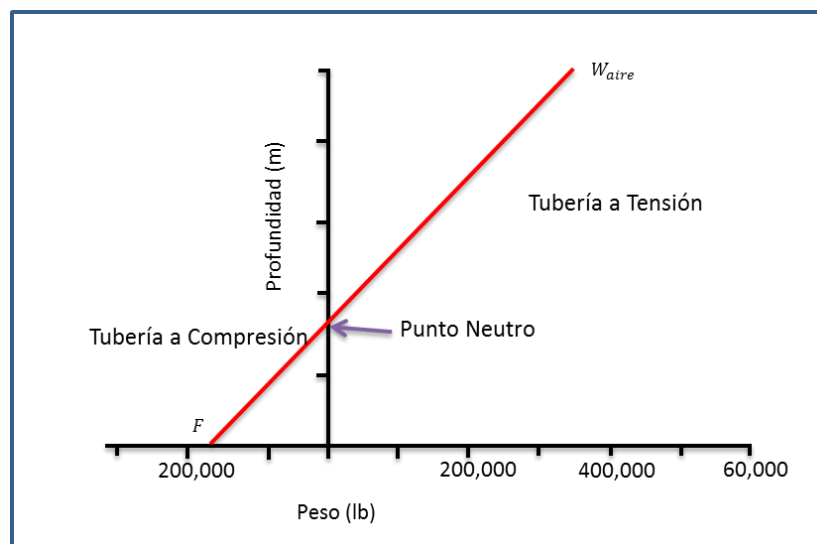
Figura 57. Grafica de diseño por tensión.
