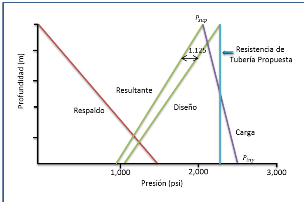
Figura 55. Gráfica de diseño por presión interna
