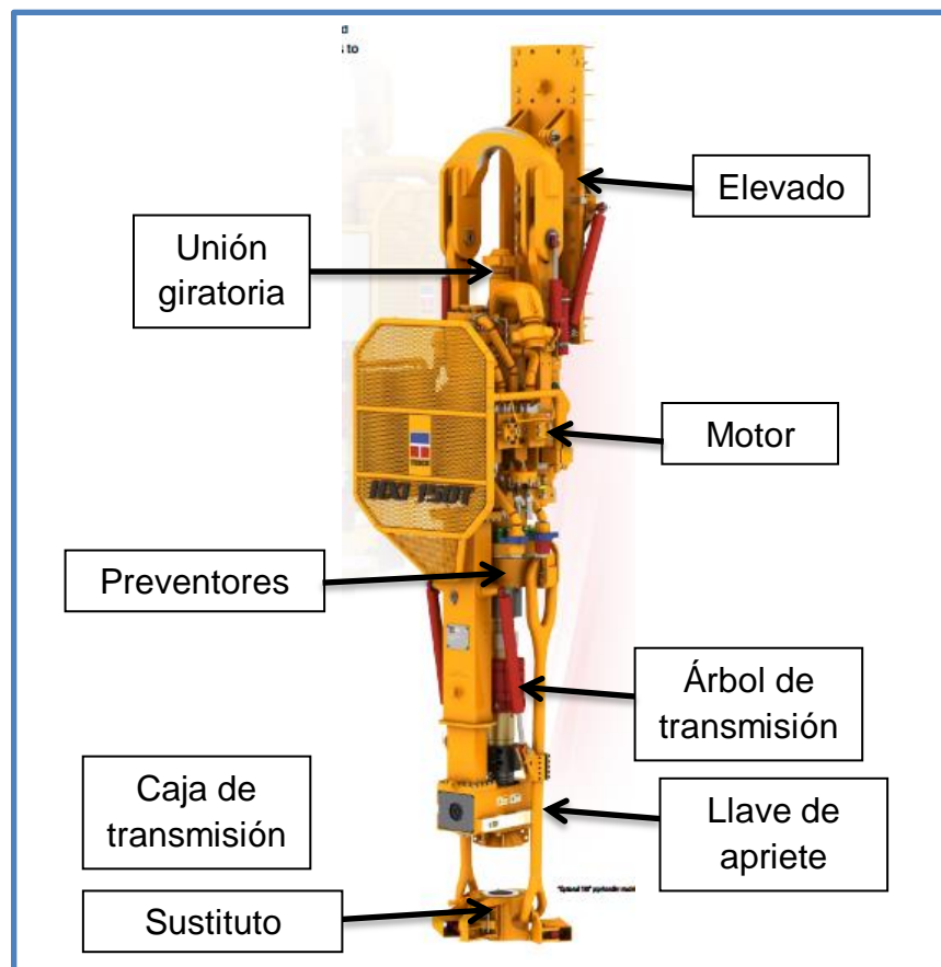
Figura 37. Componentes del Sistema Top Drive. Fuente: Página oficial Tesco Company
