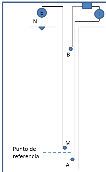
Figura 21. Configuración del registro de resistividad normal corta.
