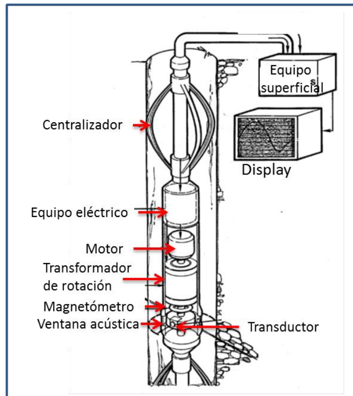
Figura 27. Herramienta de Registro de Imagen de pared de pozo. Fuente: B. Steingrímsson (2011) "Geothermal well logging"
