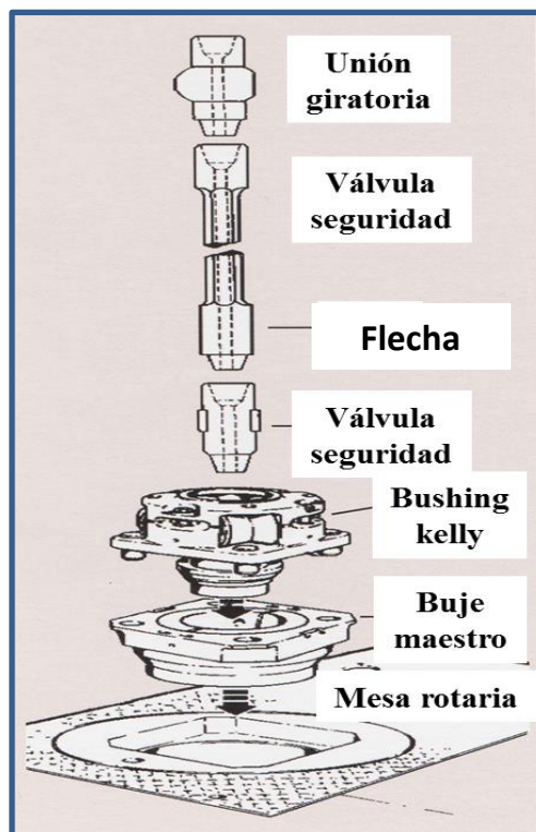
Figura 36. Sistema de rotación convencional.
