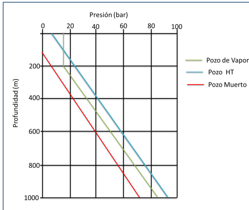
Figura 30. Perfiles de presión comunes en pozos geotérmicos. Fuente: B. Steingrímsson (2013) "Geothermal well logging: Temperature and pressure logs"
