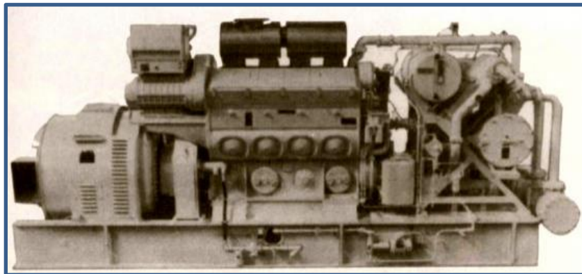
Figura 33. Motor de combustión interna. Fuente: J. Tester (2011) “Geothermal well drilling”
