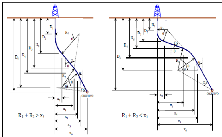
Figura 63. Trayectoria Tipo S modificada. Fuente: Guía práctica para el diseño de la perforación direccional, PEMEX.
