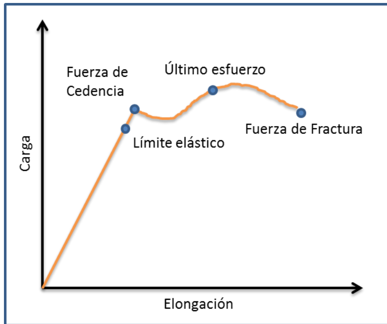
Figura 54. Comportamiento elástico de un tubo.
