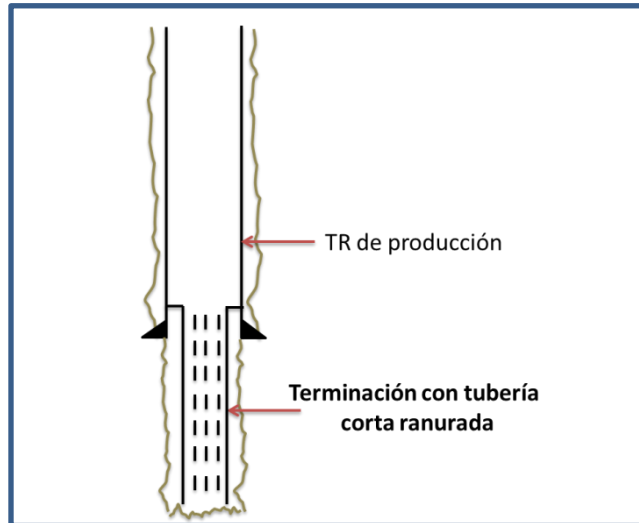
Figura 66. Terminación con tubería corta ranurada.
