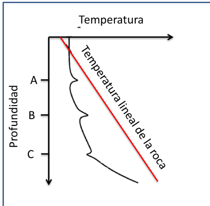
Figura 29. Perfil de temperatura en un pozo cerrado. Fuente: B. Steingrímsson (2013) "Geothermal well logging: Temperature and pressure logs"
