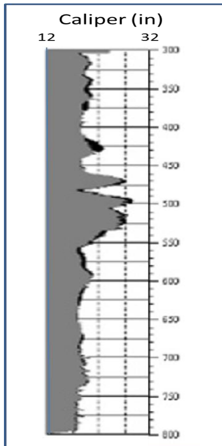
Figura 32. Ejemplo de registro de caliper en un pozo geotérmico. Fuente: Y. Gorbachev (1995) "Well logging: Fundamentals of method"
