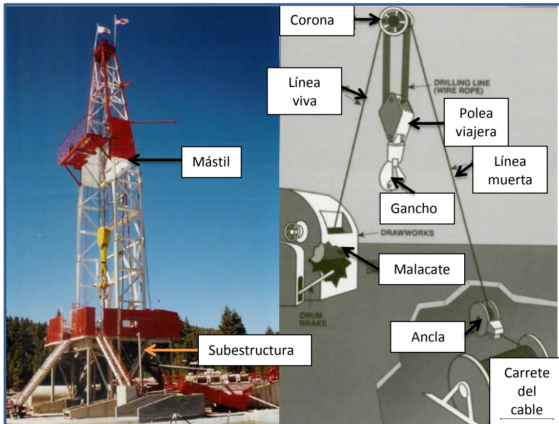
Figura 34. Componentes del sistema de izaje.
