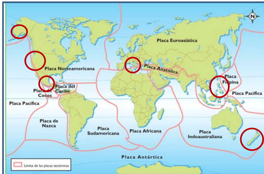
Figura 20. Mapa de las placas tectónicas y su relación con los campos geotérmicos de mayor importancia.
