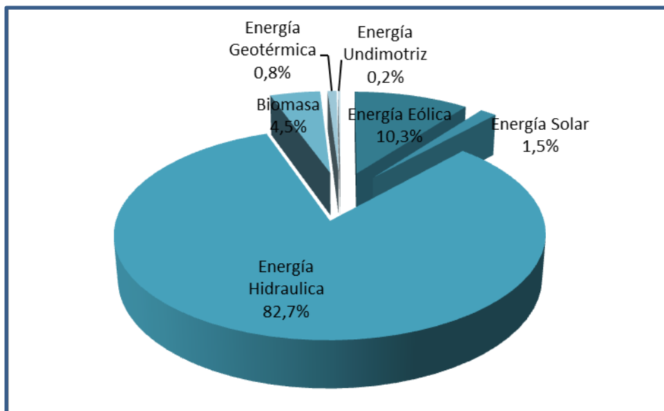
Figura 9. Energías renovables utilizadas en el mundo y su porcentaje de uso. Fuente: Renewables Global Status Report 2011
