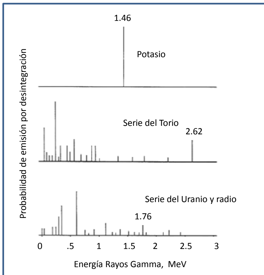
Figura 23. Distribución de la energía de los rayos gamma emitida por los tres isotopos naturales radioactivos. Fuente: B. Steingrímsson (2011) "Geothermal well logging"
