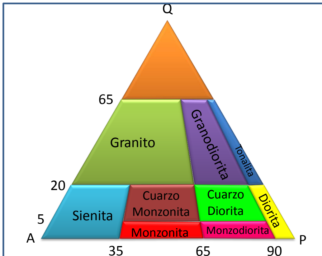
Figura 15. Diagrama ternario de la clasificación de las rocas ígneas faneríticas. Clasificación IUGS.
