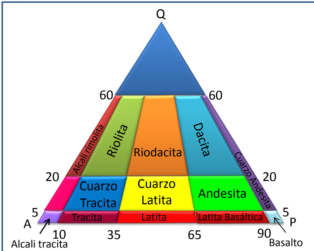
Figura 16. Diagrama ternario de la clasificación de las rocas afaníticas. Clasificación IUGS.
