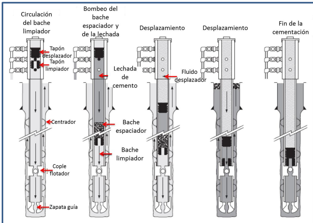
Figura 60. Proceso convencional de cementación primaria en pozos geotérmicos.
