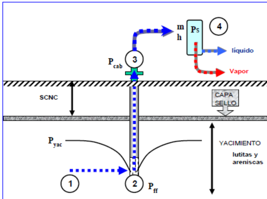
Figura 72. Proceso de producción de vapor en un pozo geotérmico.
