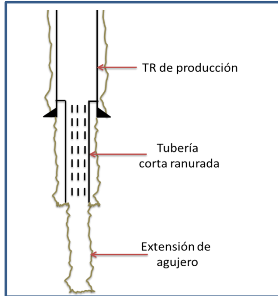
Figura 67. Terminación de un pozo exploratorio con tubería ranurada colgada y extensión de agujero.
