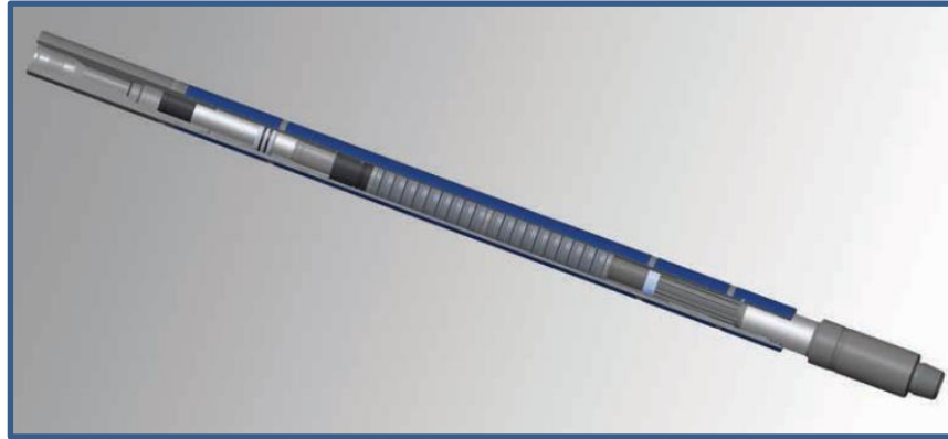
Figura 49. Amortiguadores. Fuente: Catalogo Schlumberger.
