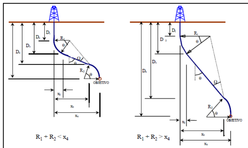
Figura 61. Trayectoria Tipo Slant. Fuente: Guía práctica para el diseño de la perforación direccional, PEMEX.
