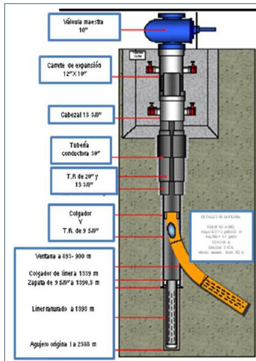
Figura 68. Estado mecánico (diseño) del pozo bilateral H-8D en el campo geotérmico de Los Humeros, Puebla. Fuente: Geotermia: Revista Mexicana de Geoenergía.
