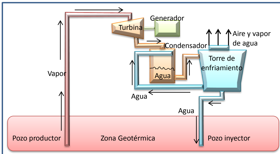
Figura 6. Diagrama de una planta de vapor seco.
