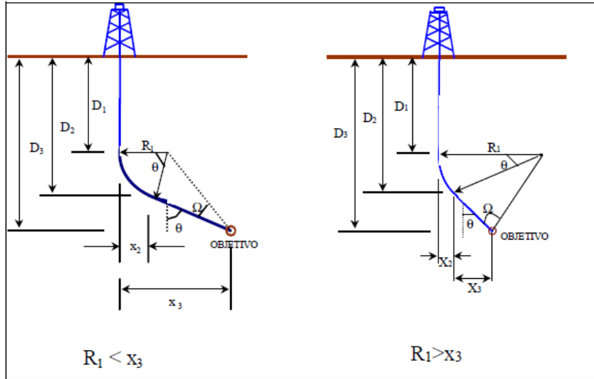
Figura 62. Trayectoria Tipo S. Fuente: Guía práctica para el diseño de la perforación direccional, PEMEX.
