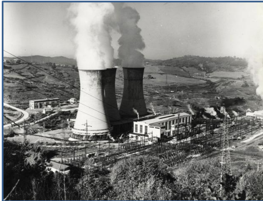
Figura 2. Primera central generadora de electricidad a partir de fluidos geotermiales. Fuente: Página oficial del Museo della geotermia.
