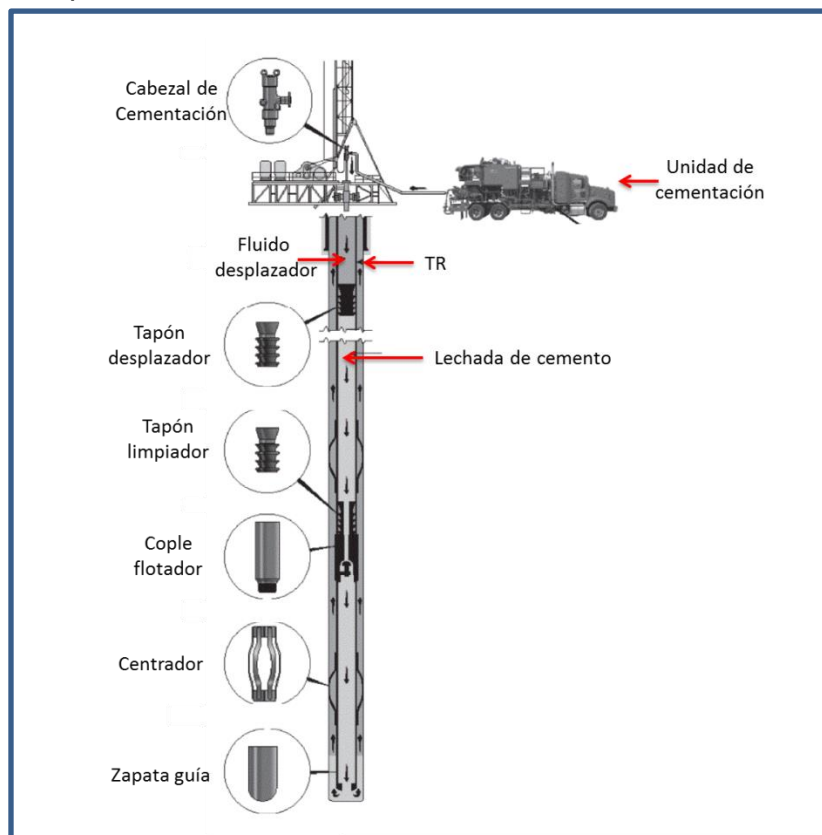
Figura 59. Equipo utilizado durante la cementación de pozos geotérmicos.
