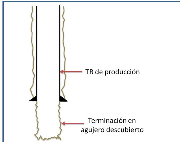
Figura 65. Terminación de un pozo geotérmico en agujero descubierto con una profundización del mismo.
