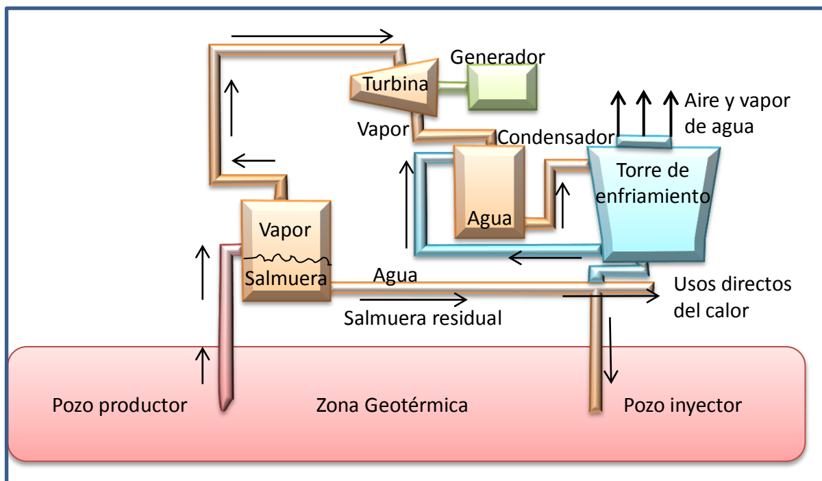
Figura 7. Diagrama de una planta de separación de vapor.
