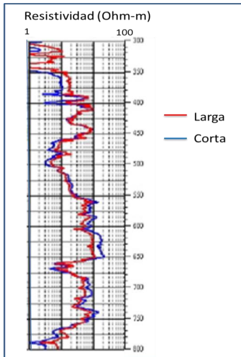
Figura 22. Ejemplo de registro de resistividad en un pozo geotérmico. Fuente: B. Steingrímsson (2011) "Geothermal well logging"
