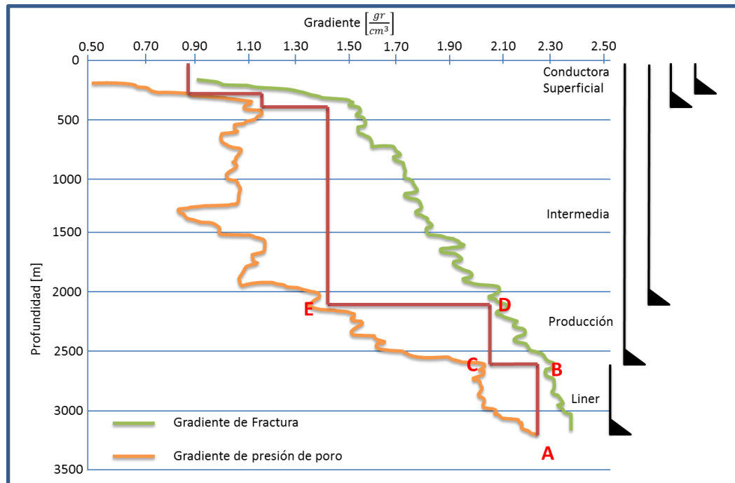
Figura 52. Método gráfico de asentamiento de tubería.
