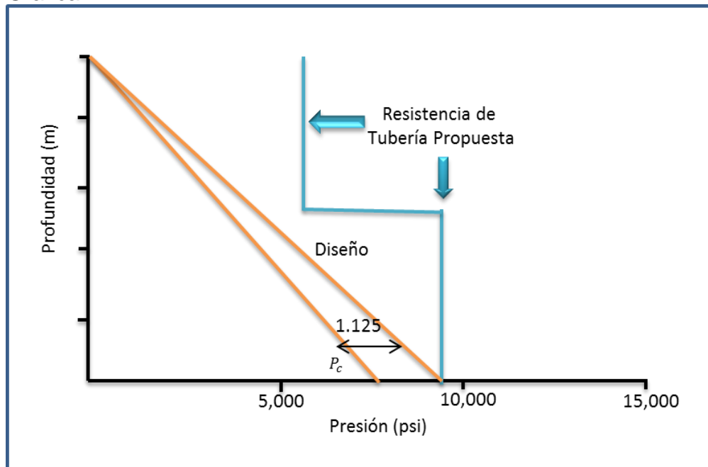
Figura 56. Grafica diseño por colapso.
