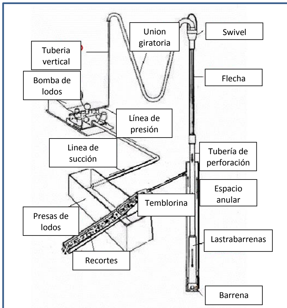
Figura 35. Sistema de circulación. Fuente: P. Ngugi, (2008), "Geothermal well drilling"
