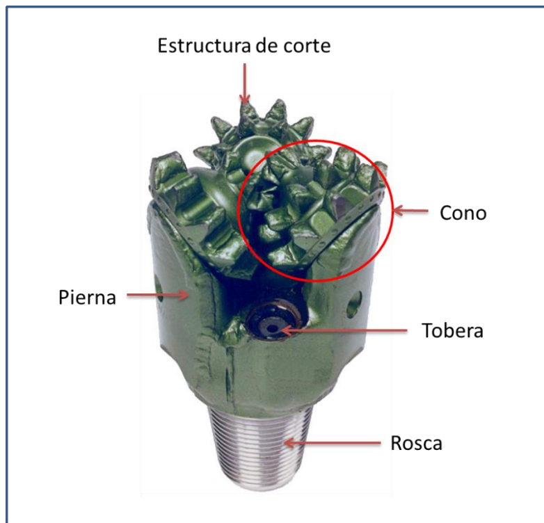
Figura 40. Barrena tricónica. Fuente: G. Culver (2000) “Drilling and well construction”
