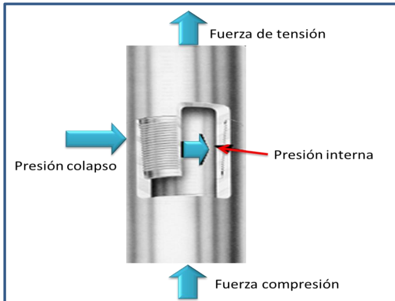
Imagen 53. Esfuerzos axiales que actúan en la tubería de revestimiento.
