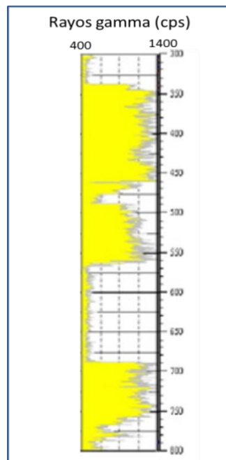
Figura 24. Ejemplo de registro de Rayos Gamma en un pozo geotérmico. Fuente: Y. Gorbachev (1995) "Well logging: Fundamentals of method"
