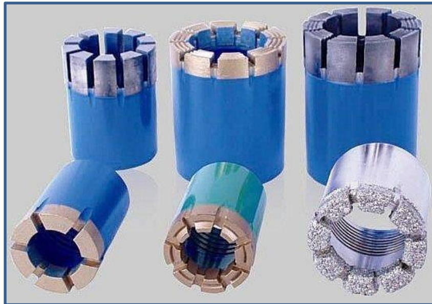
Figura 42. Barrenas nucleadoras. Fuente: Página oficial de “Huanyu bits”
