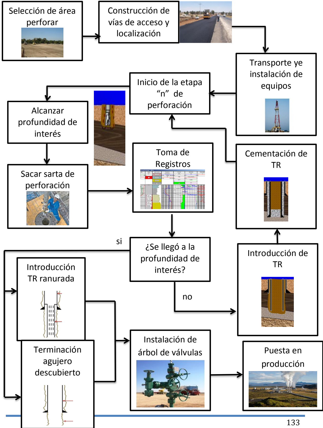
Anexo 2. Diagrama del proceso operativo de perforación de pozos geotérmicos
