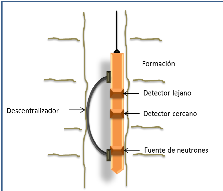
Figura 25. Herramienta de Registro Neutrón-Neutrón. Fuente: B. Steingrímsson (2011) "Geothermal well logging"
