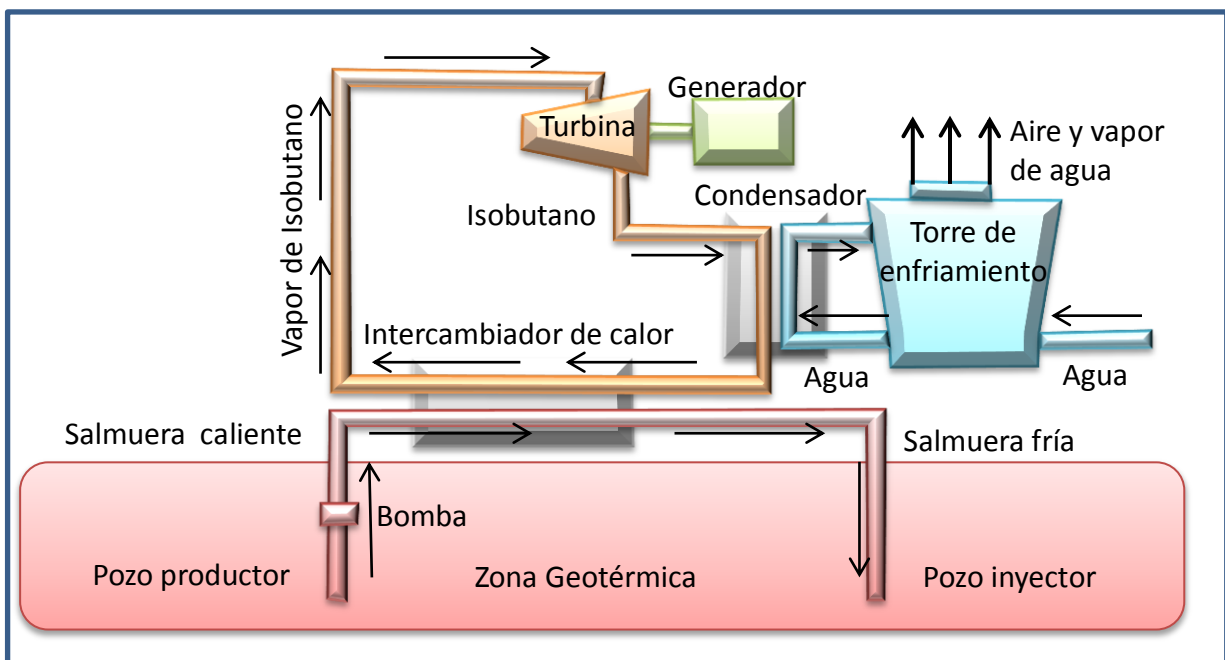
Figura 8. Diagrama de una planta de ciclo binario.
