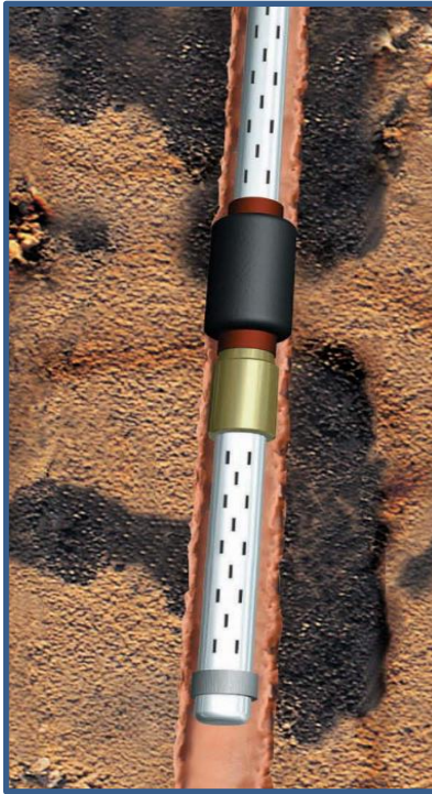
Figura 70. Esquema de un pozo terminado en TR corta ranurada, donde se muestra un empacador para agujero descubierto.
