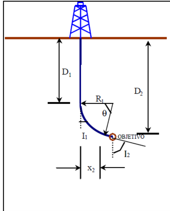
Figura 64. Trayectoria de incremento continuo. Fuente: Guía práctica para el diseño de la perforación direccional, PEMEX.
