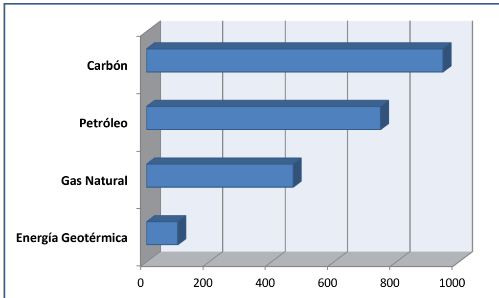
Figura 3. Grafica comparativa de emisiones de CO 2 , de las principales fuentes de generación de electricidad (Kg/MWh). Fuente: IAEA 2010
