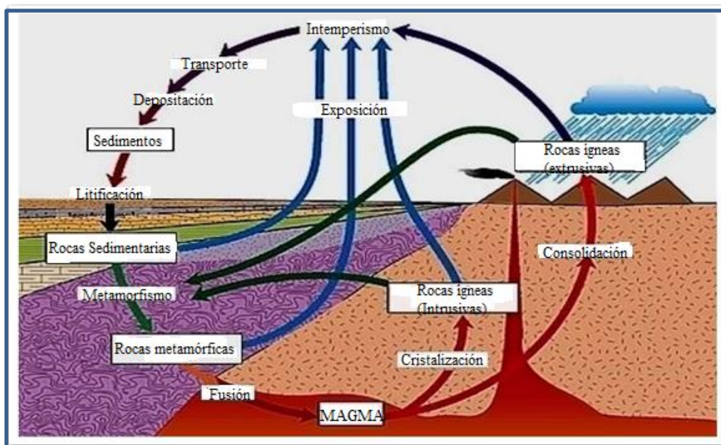
Figura 18. Ciclo de las rocas
