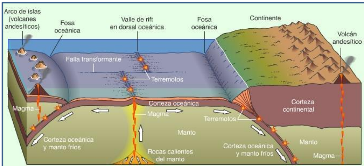
Figura 19. Límites de las placas tectónicas. Fuente: Página oficial de International Geothermal Association
