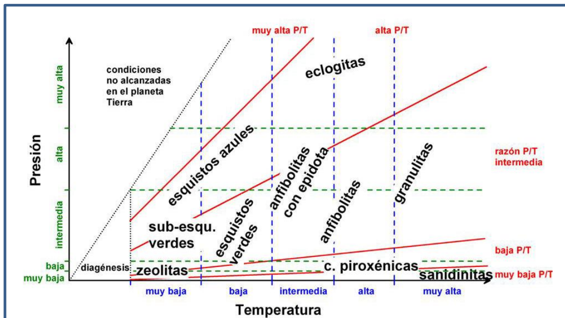
Figura 17. Clasificación de las rocas metamórficas según la presión y la temperatura a la que se encuentran. Fuente: Página oficial de la UGR.
