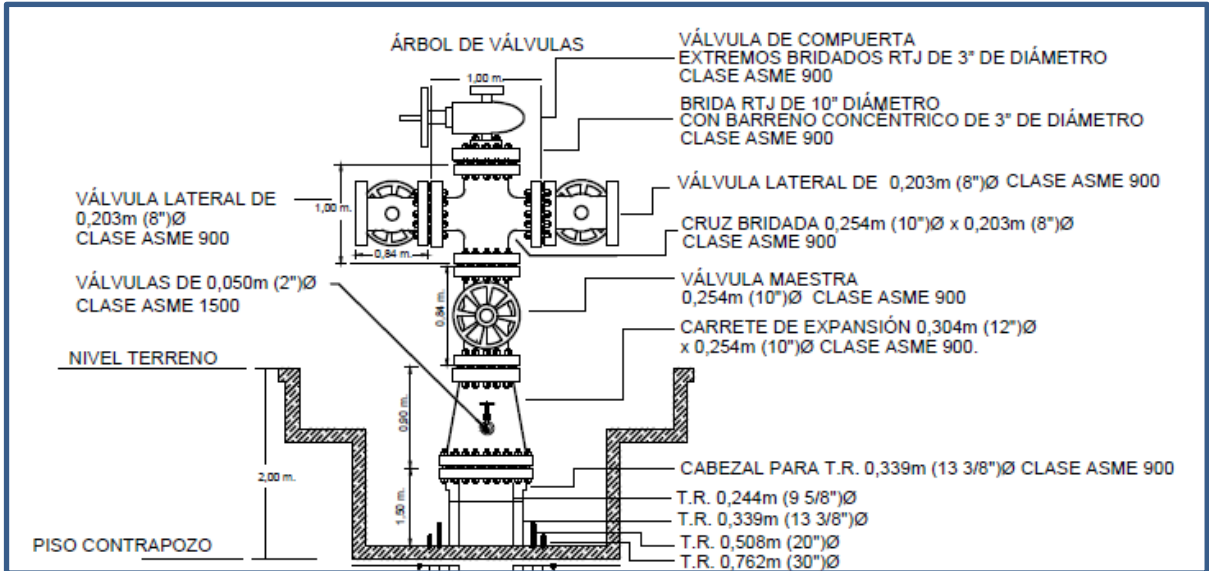
Figura 69. Cabezal de TR's y árbol de válvulas típico de un pozo geotérmico.
