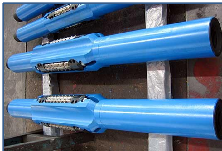
Figura 48. Rimadores. Fuente: Catalogo Schlumberger.
