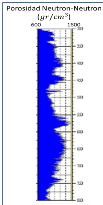
Figura 26. Ejemplo de registro Neutron-Neutron en un pozo geotérmico. Fuente: Y. Gorbachev (1995) "Well logging: Fundamentals of method"
