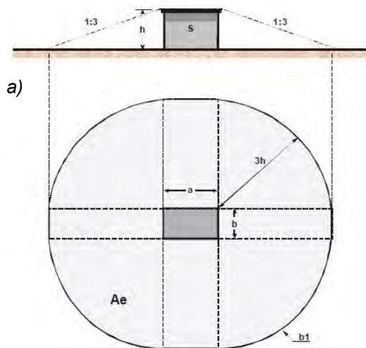
Figura 4.2; Área de captura equivalente para una estructura de terreno plano y (a) con techo plano, (b) con techo a dos aguas.
