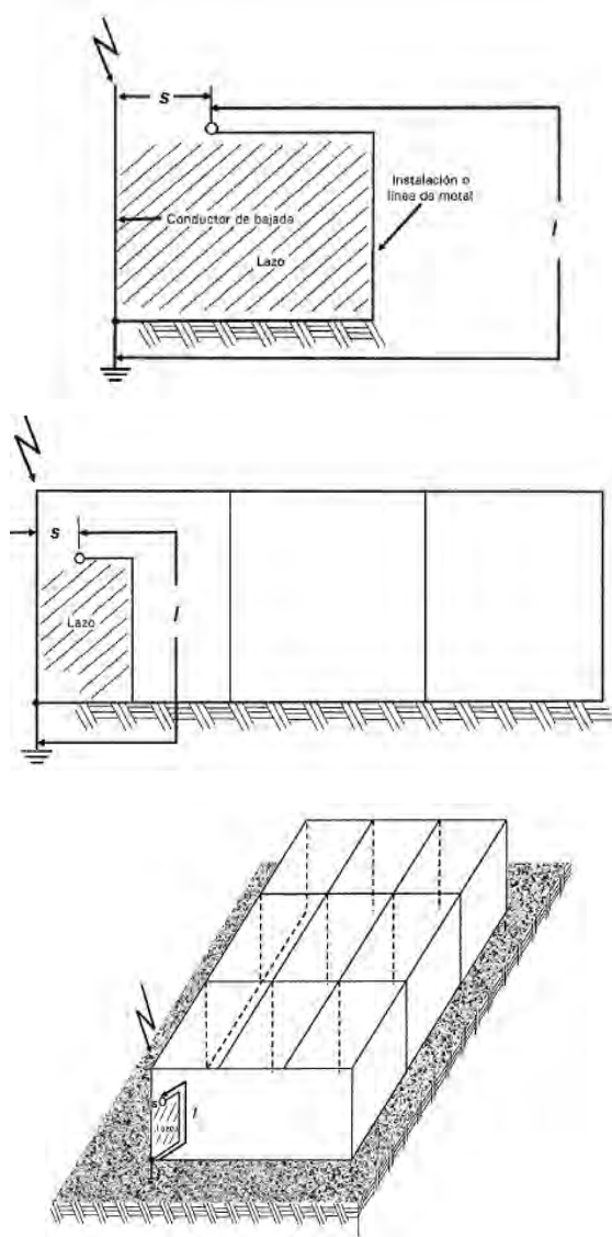
Figura 4.13; Valor del coeficiente k_c , para (a) uno o dos, (b) tres o cuatro, (c) más de cuatro conductores de bajada.
