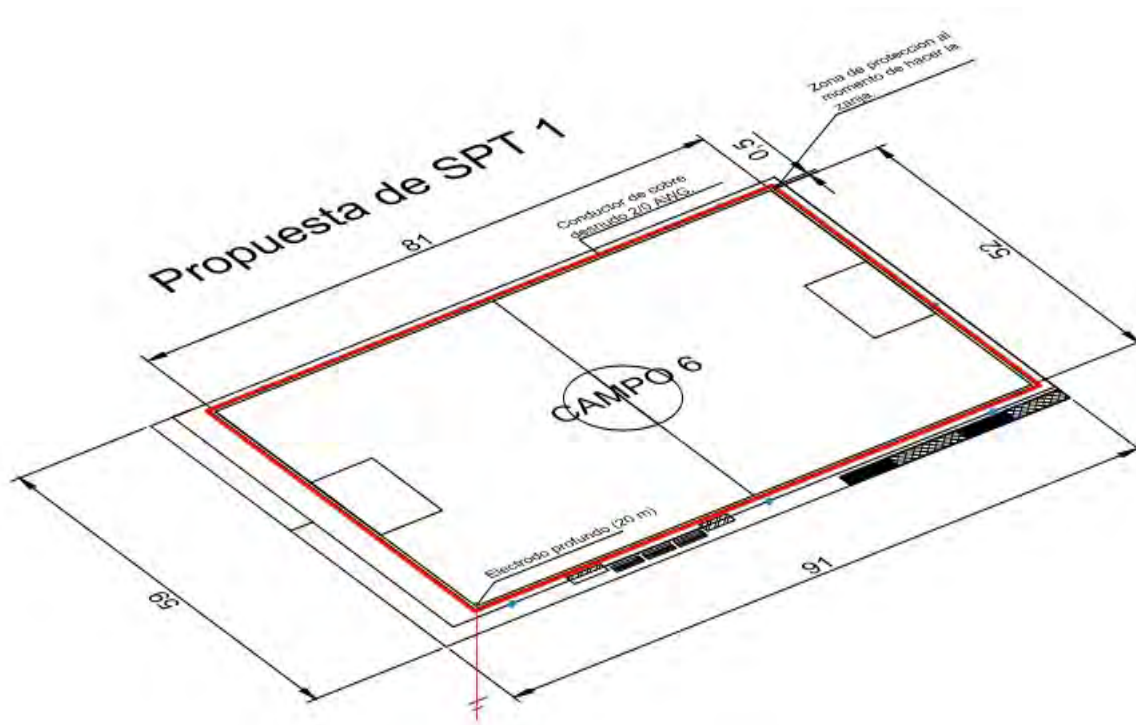
Figura 5.11; Primera propuesta SPT.
