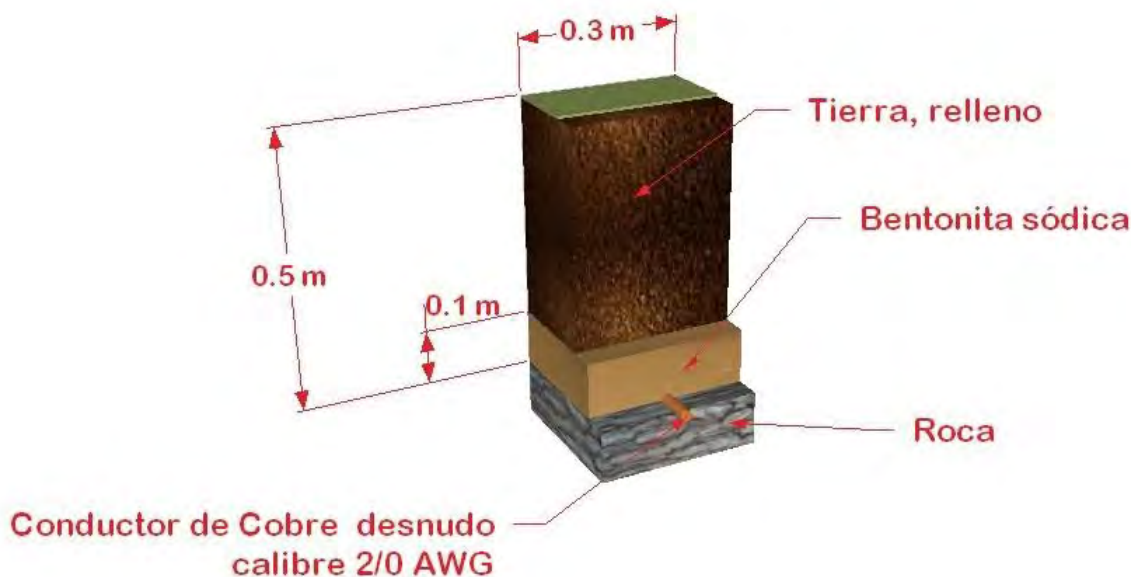
Figura 5.13; Perfil de suelo de la primera propuesta de SPT.
