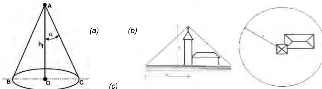
Figura 4.7; Protección cónica.
