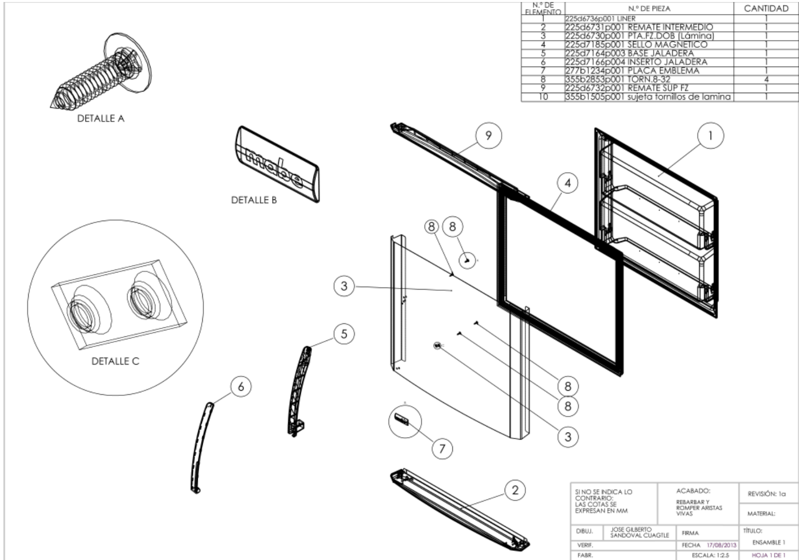
Ilustración 2.1 Vista explosionada del ensamble de la puerta superior del refrigerador (vista exterior).
