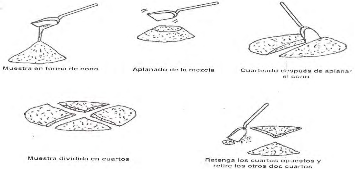
Figura 3.4. Cuarteo manual.
