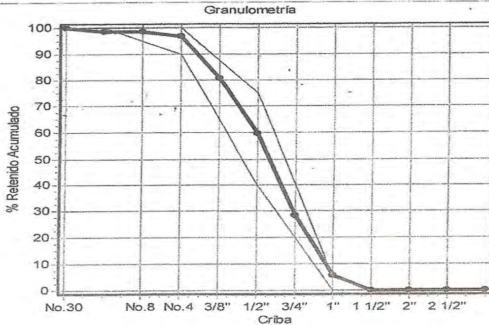
Figura 4.3. Curva granulométrica.
