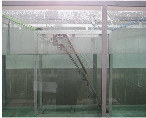
Fig. 5.32 Cámara OWC prototipo
