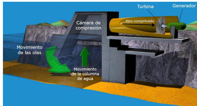
Figura 3.7 Columna de agua Oscilante [Rodríguez, 2010]
