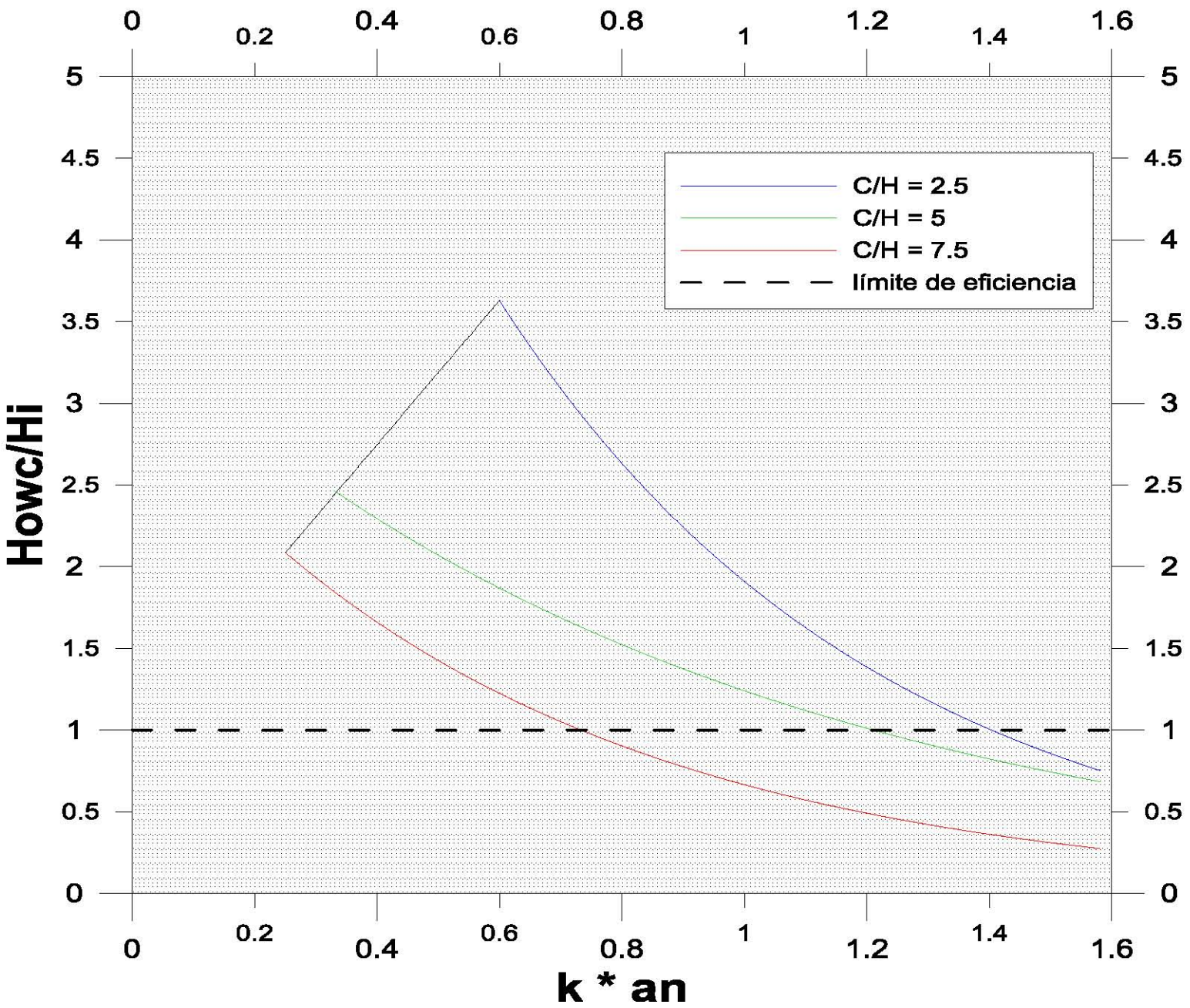
Fig. 5.26 Nomograma OWC
