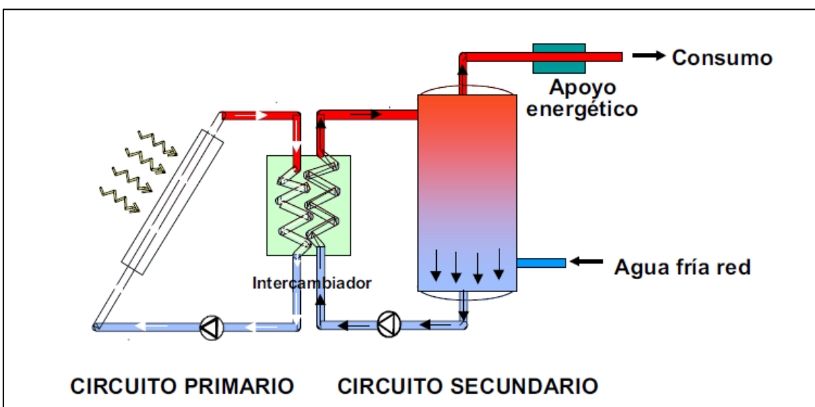
FIG. 18- CIRCUITO CERRADO
