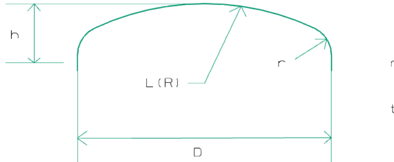
Figura 2.3 Diseño de la tapa para el biodigestor. (Megyesy, 1992)
