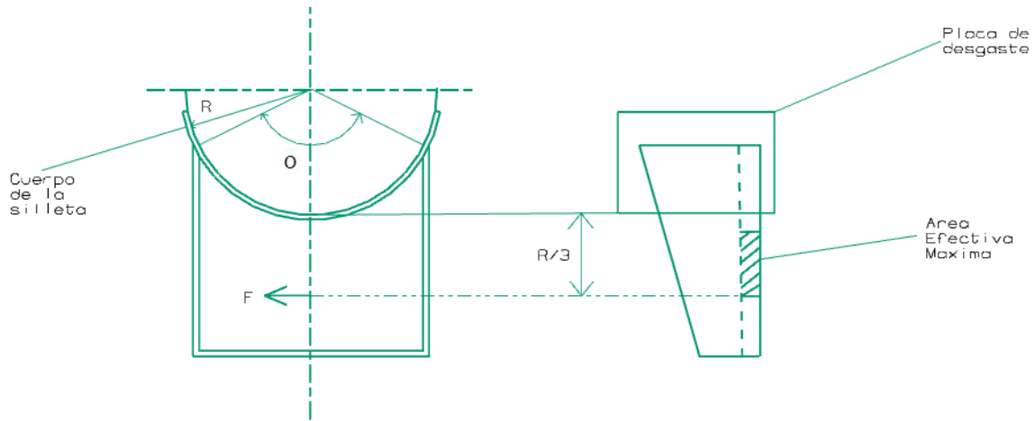
Figura 2.5 Diseño de la silleta. (Megyesy, 1992)
