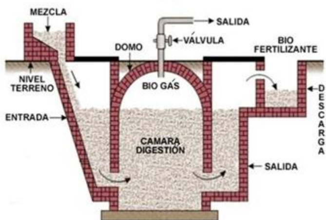
Figura 1.4 Biodigestor Chino. (Torre Guillén D., 2009)
