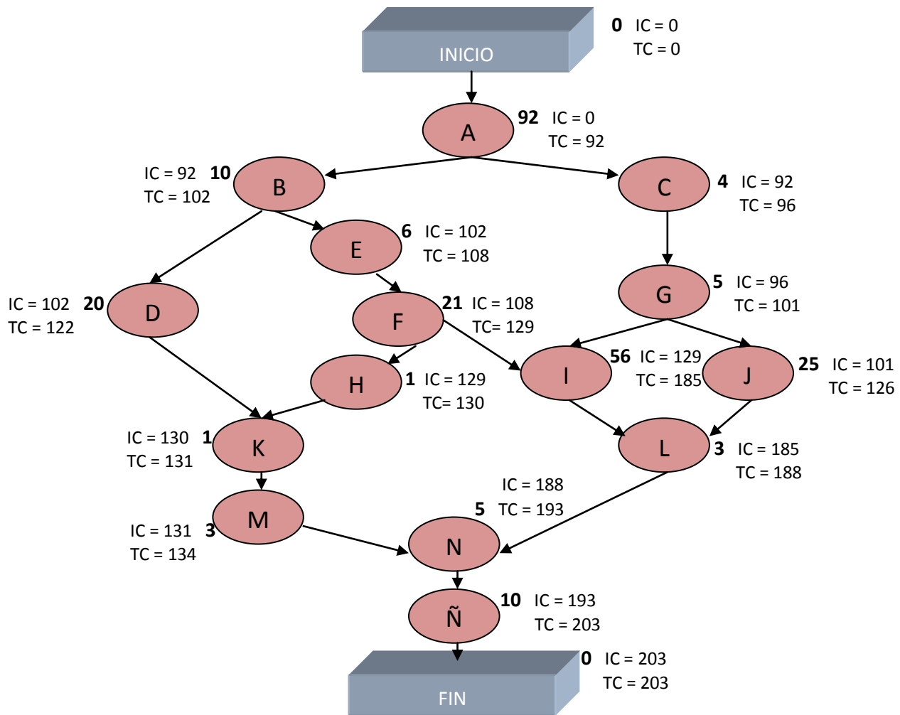
Figura 14. Red del proyecto con tiempos de inicio cercano (IC) y tiempos de terminación cercano (TC). Elaboración propia
