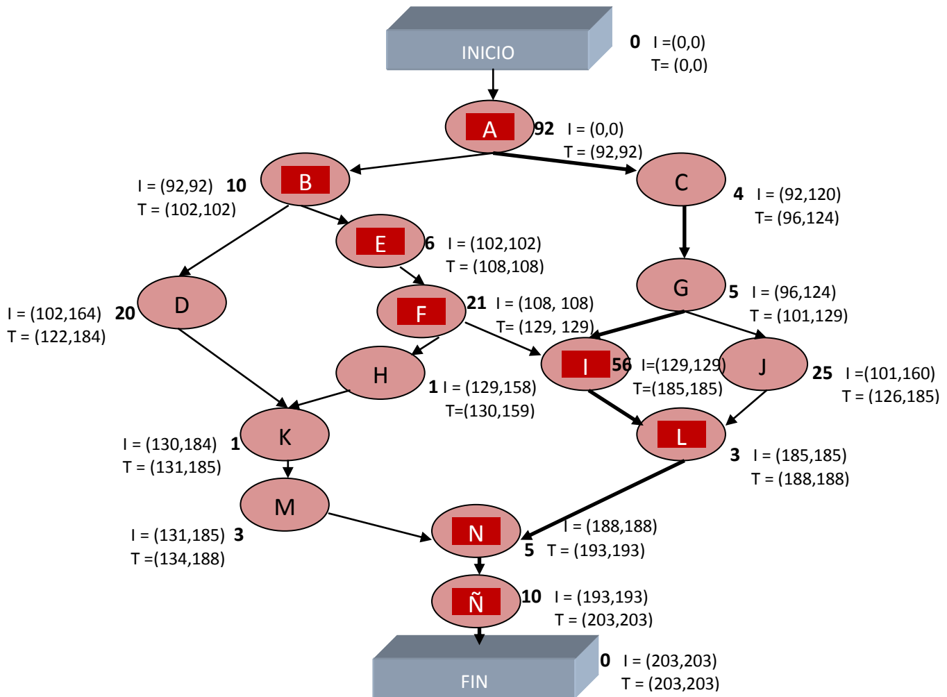
Figura 16. Red completa del proyecto con IC e IL (paréntesis superiores) y TC y TL (paréntesis inferiores). Elaboración propia
