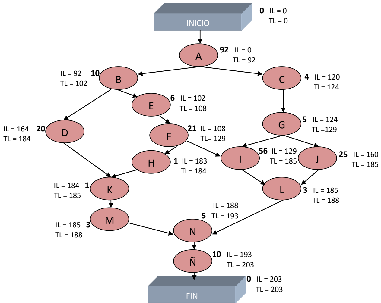
Figura 15. Red del proyecto con tiempos de inicio más lejano (IL) y tiempos de terminación más lejano (TL). Ruta crítica. Elaboración propia
