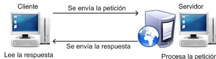
Figura 1.6: Modelo Cliente/Servidor
