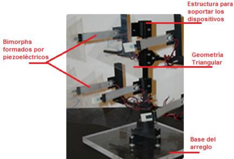
Fig. 2.2.2.2.2 Componentes del arreglo Piezo-Leaf [19].
