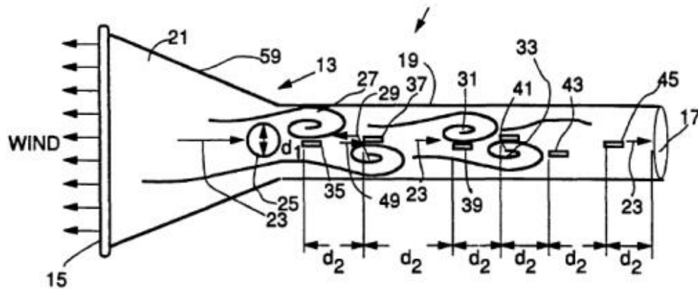
Fig. 2.2.1.8.1 Figura esquemática del "Wind Power Generator and Velocimeter", en donde se puede apreciar la colocación de los piezoeléctricos y los vórtices que los deforman. [27]
