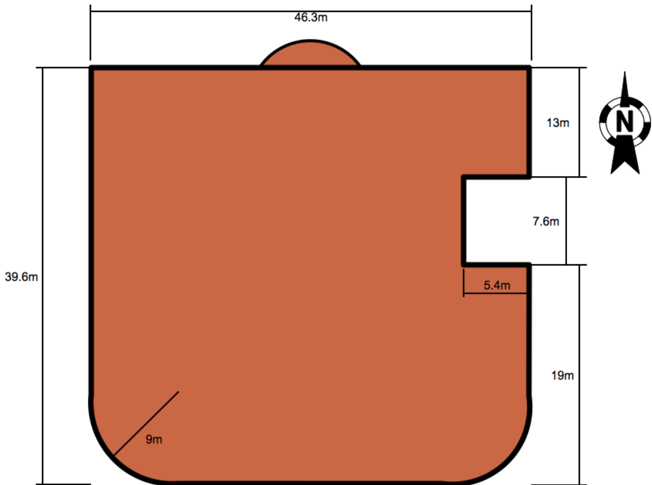
Figura 28. Superficie de captación Biblioteca Enrique Rivero Borrell
