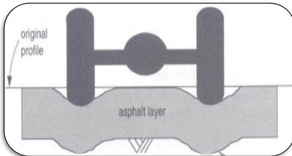
Figura 3.1 Deformación permanente debido a una capa subyacente débil
