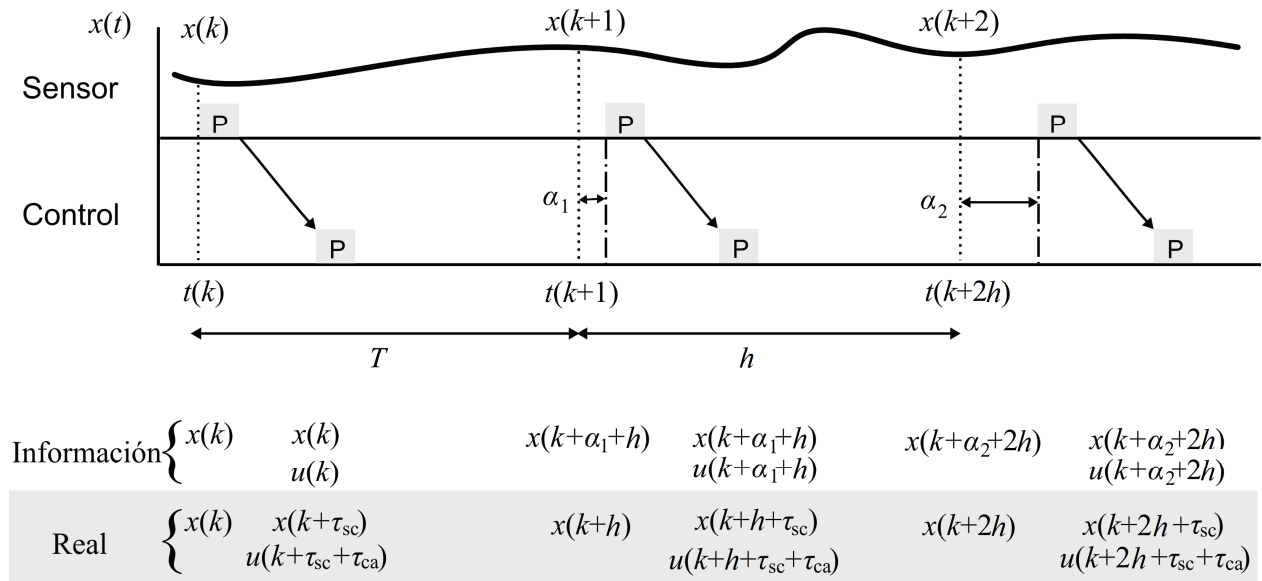
Figura 2.4. Representación del efecto del muestreo variante en el tiempo en un NCS.
