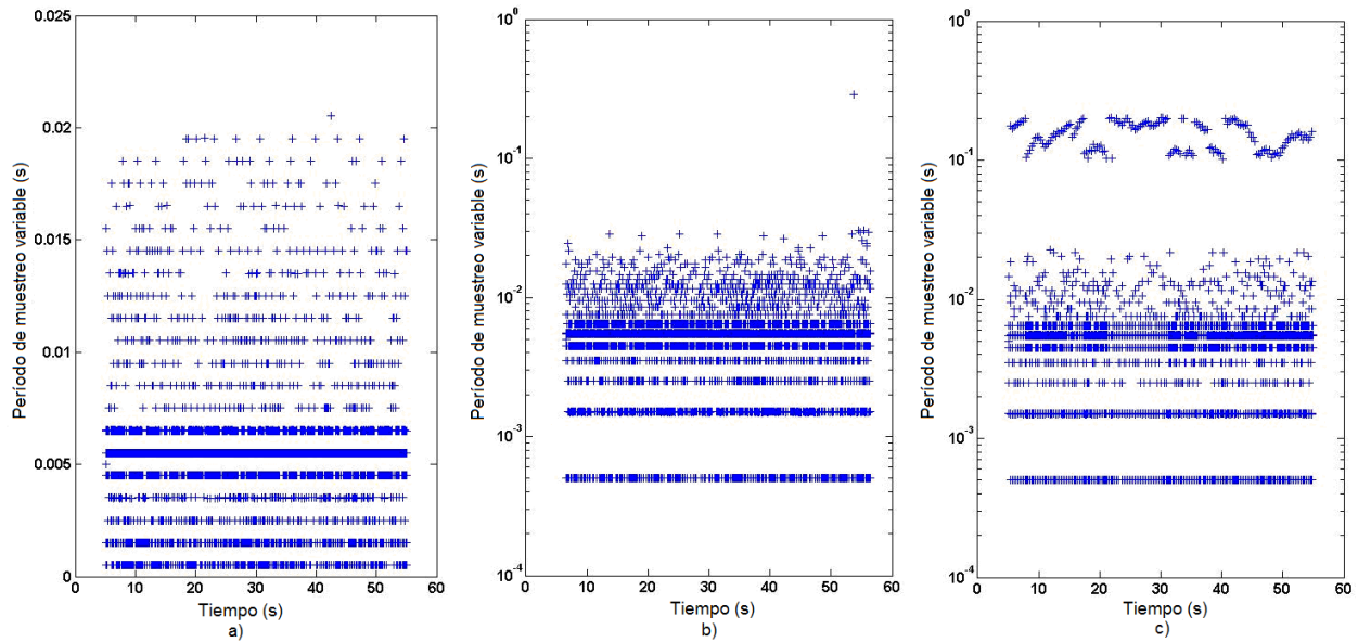
Figura 7.21. Periodos de muestreo variable para tráfico a) ligero, b) medio y c) severo
