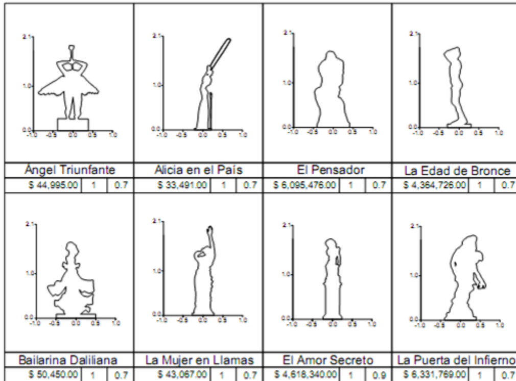
Figura 3.5 Parte del inventario de contenidos susceptibles a fallar por volteo o deslizamiento del Museo Soumaya, las dimensiones están en metros y la moneda en $US
