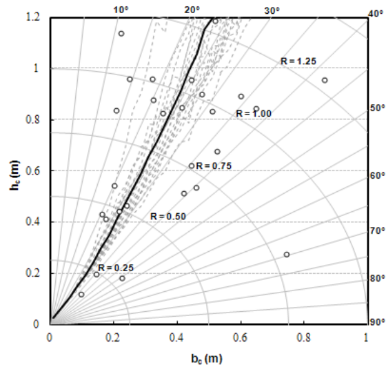
Figura 4.19 Gráfico con línea de limite falla media (línea continua) y contenidos (círculos), los círculos que están por encima de la línea son muy propensos al vuelco, mientras que los que están debajo no son propensos al vuelco bajo una aceleración dada.
