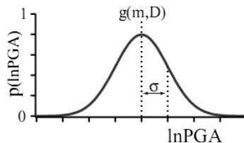
Figura 4.2 Curva que ilustra los parámetros de la ecuación (4.2)
