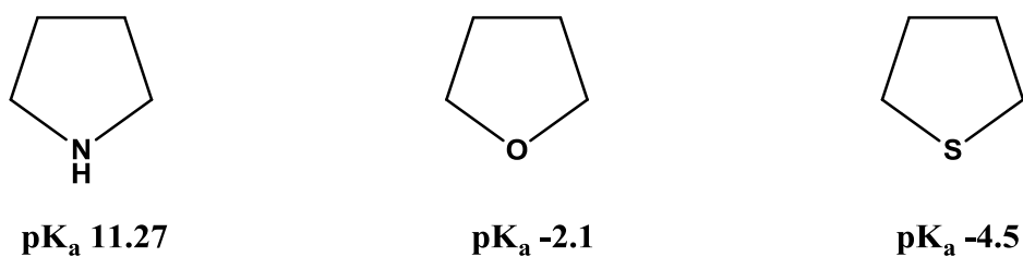
Figura 5. Valores de \text{pK}_a para análogos de heterociclos aromáticos
