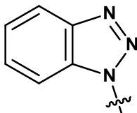
Figura 13. Estructura del benzotriazol
