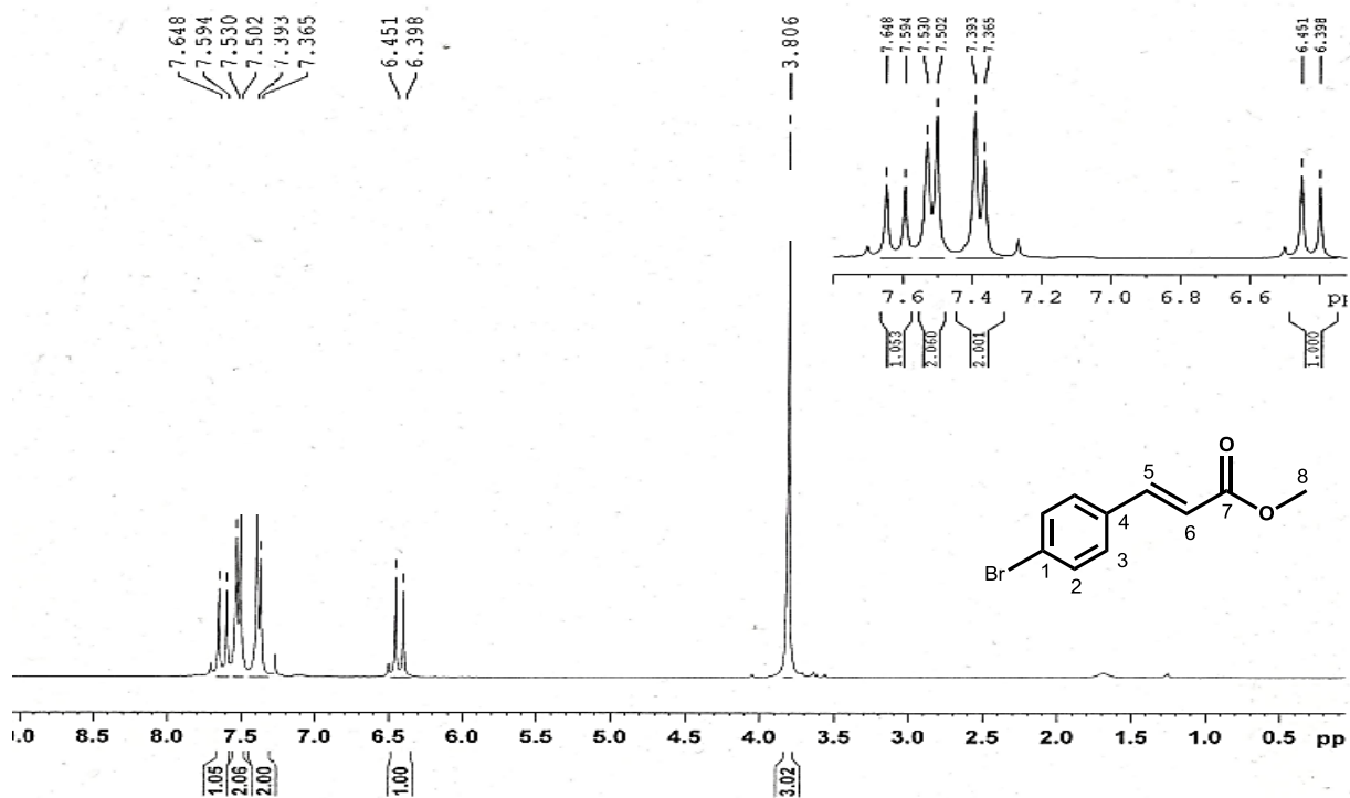
Espectro 19. RMN ^1\text{H} del producto de acoplamiento C-C 17
