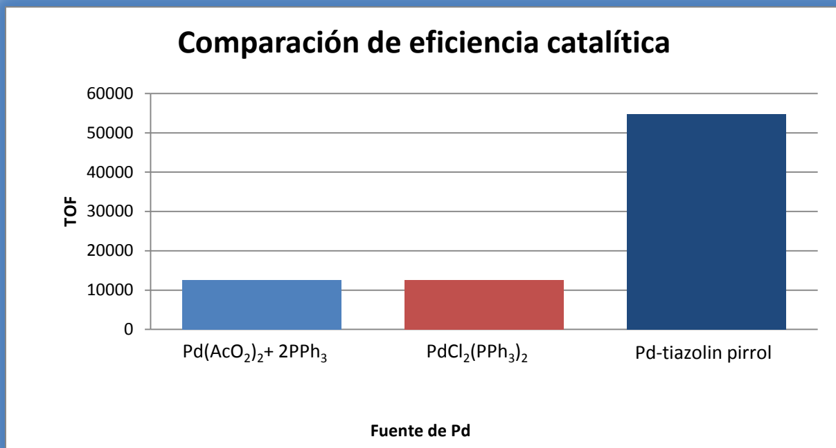
Grafica 8. Comparación de la eficiencia catalítica de los sistemas utilizados en la reacción de Heck
