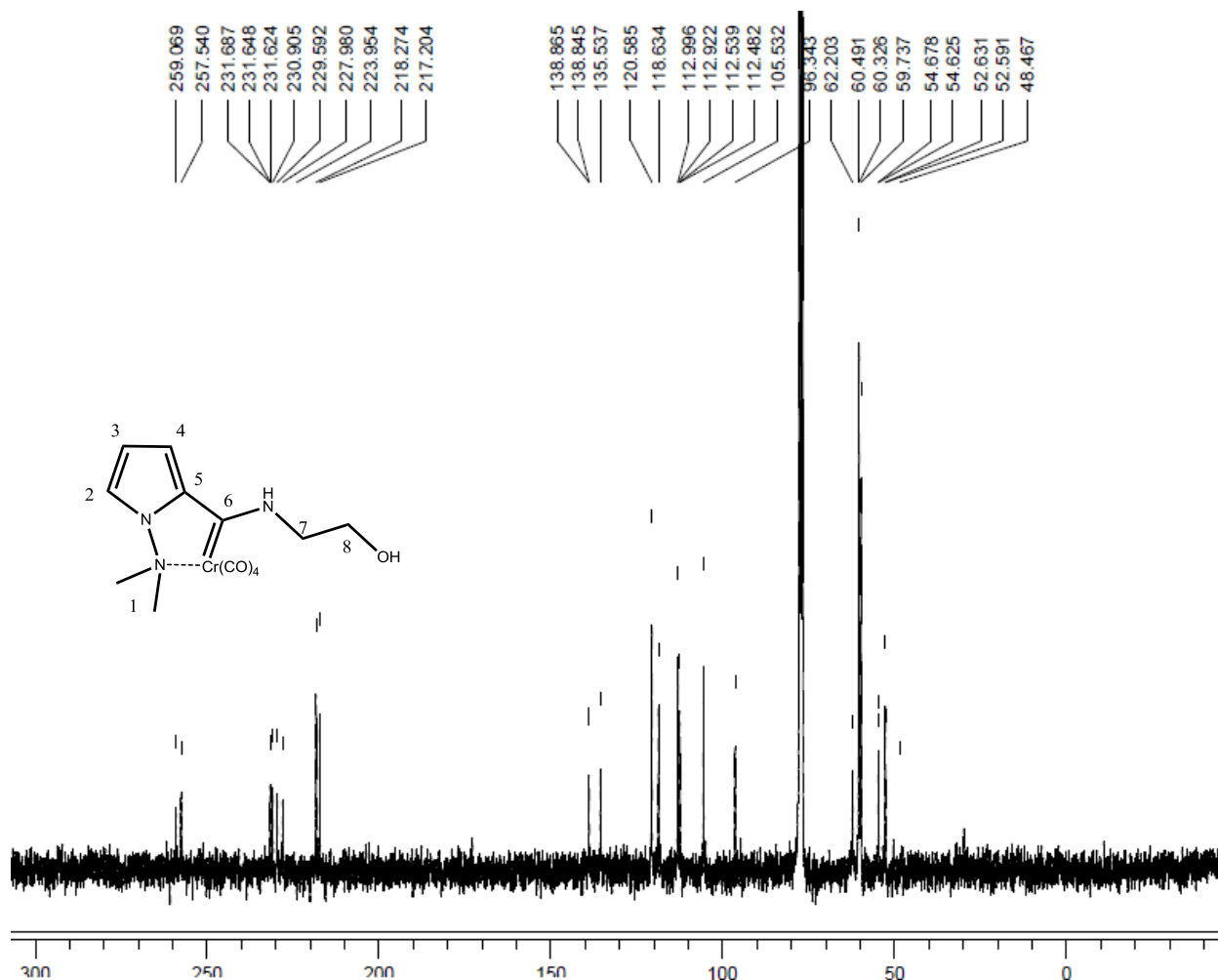
Espectro 7. Espectro de RMN 13 C para el compuesto 3
