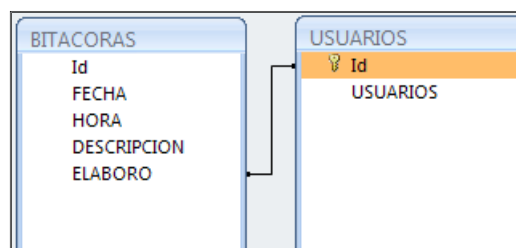
Figura 3. 8. Diagrama físico.
