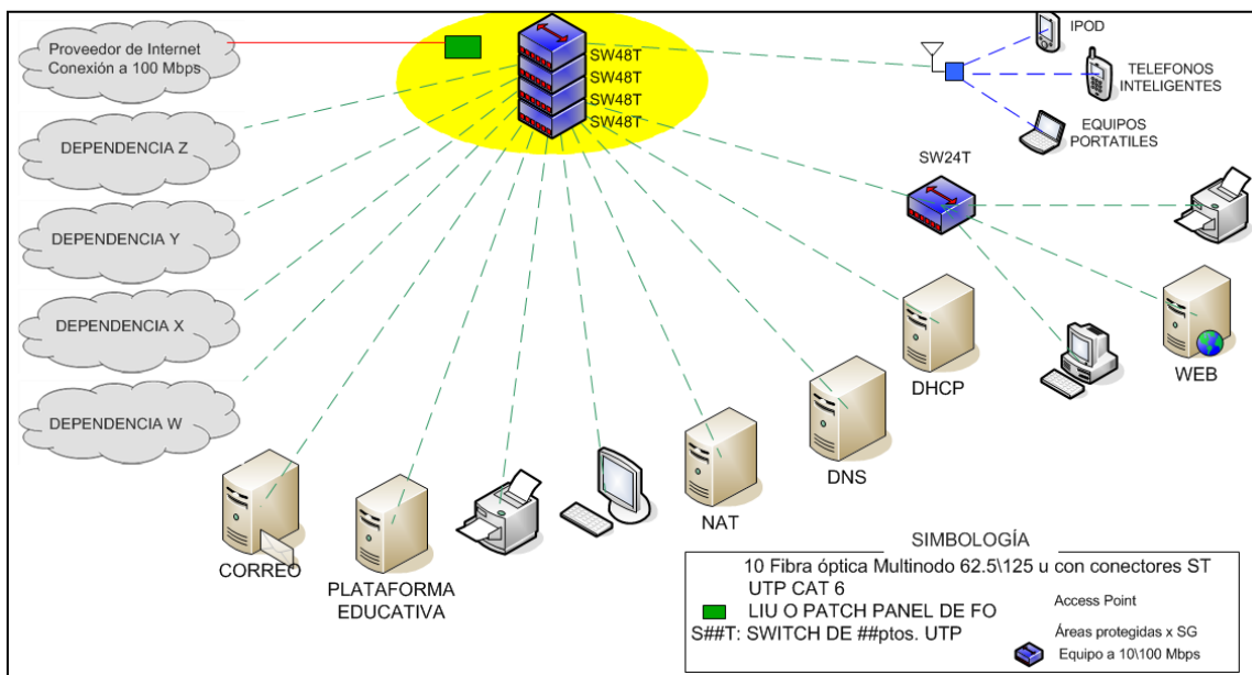
Figura 2. 1. Detalle topológico de la dependencia
