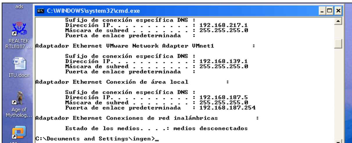
Figura 3. 46. Configuración de IP.
