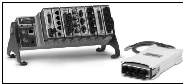
Fig.IV.6. cDAQ 9188 y Ethernet Dispositivos de Adquisición de Datos NI
