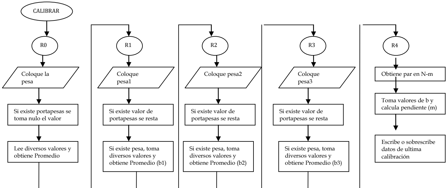
Fig. VI.1. Diagrama de flujo de los módulos de programas
