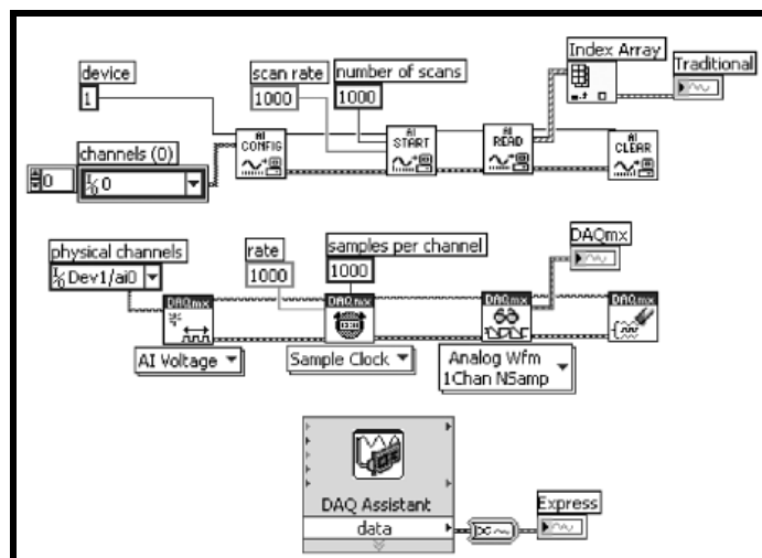
Fig.V.26. Comparativa de código (Traditional DAQ, DAQmx y Express)
