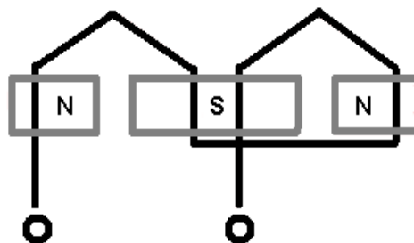
Figura No. 5.2 Bobinado por polos.
