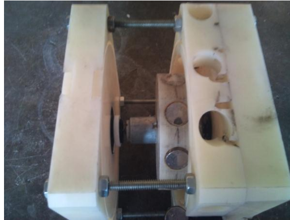
Fotografía No. 7.12 Motor armado.
