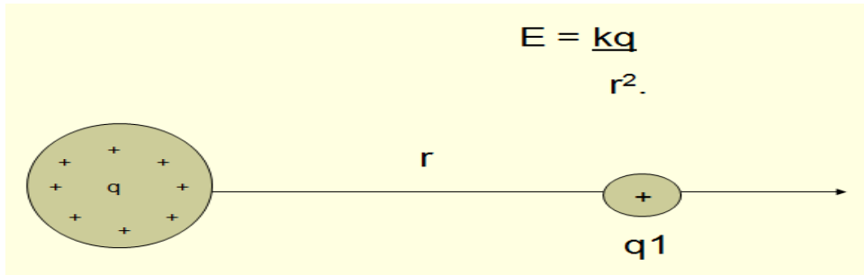
Figura No.1.6 Intensidad del campo eléctrico E, producido por una carga q a una distancia r del centro de dicha carga.
