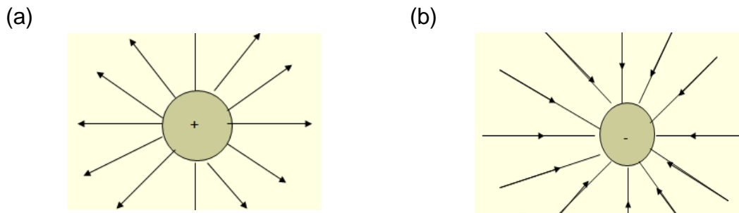
Figura No.1.5 La dirección y el sentido de la intensidad del campo eléctrico a) están dirigidos hacia fuera de la carga. b) Si la carga es negativa, E está dirigido hacia el centro.
