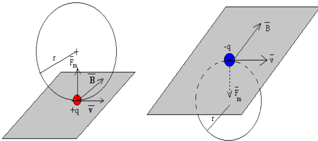
Figura No.2.4 Trayectoria circular de la partícula.
