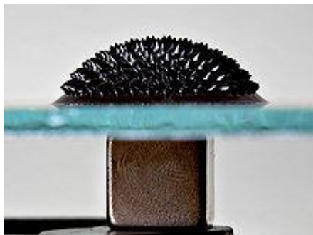
Figura No.3.1 Ferrofluido en vidrio, con un imán de tierras raras debajo de él.
