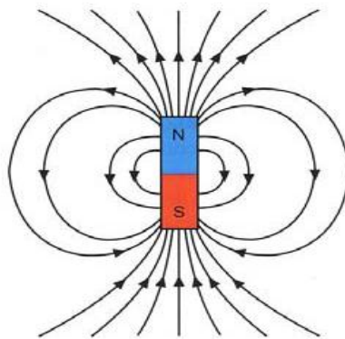
Figura No. 2.7 Líneas de fuerza de un imán.
