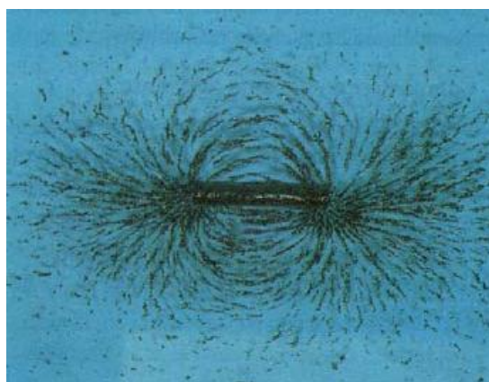
Figura No.2.6 El espectro magnético de un imán.
