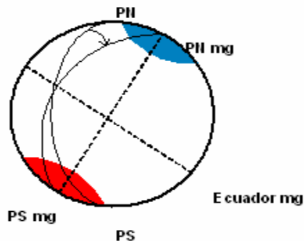
Figura No.2.1 Los polos magnéticos terrestres.
