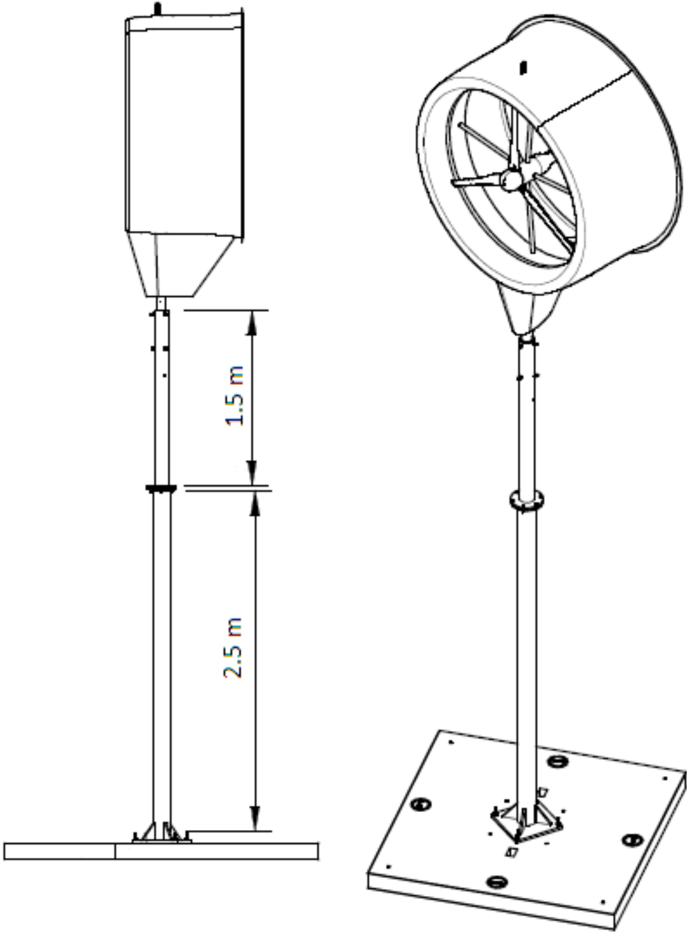
Capítulo 4 Imagen 9 Estructura del aerogenerador
