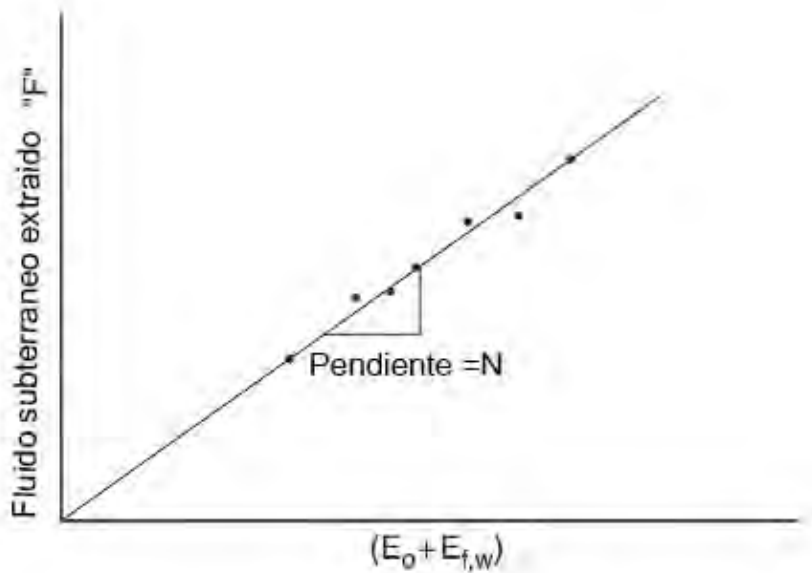
Figura 4.16 Fluidos extraídos vs. E_o + E_{f,w}
