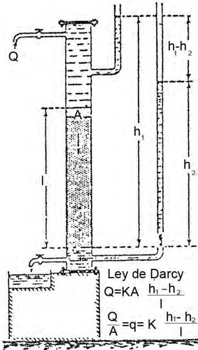
Figura 2.7 Experimento de Darcy
