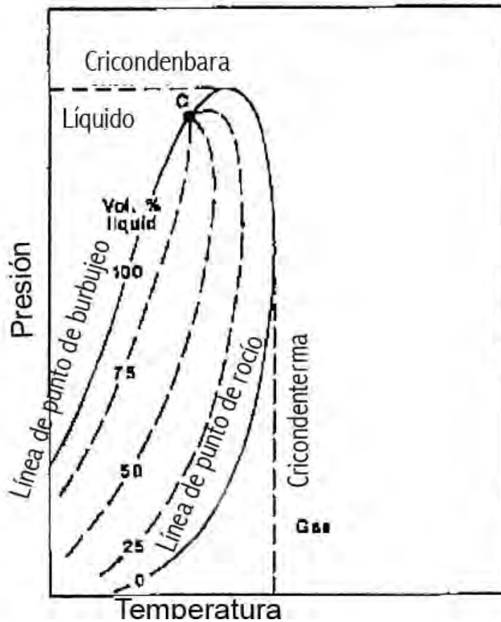
Figura 1.2 Diagrama típico de dos componentes, con las definiciones de cricondenbara y cricondenterma (William W. Mc Cain Jr. "The Properties Of Petroleum Fluids" Tulsa Oklahoma 1990. Edit. Penwell Publishing)
