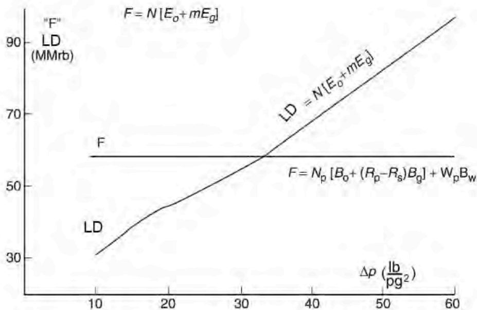
Figura 4.22 Solución del balance de materia para la presión
