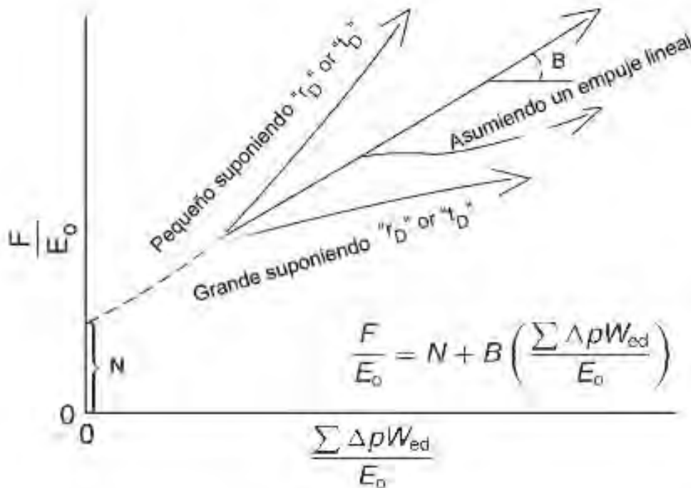
Figura 4.21 Gráfica de la forma lineal de Havlena y Odeh
