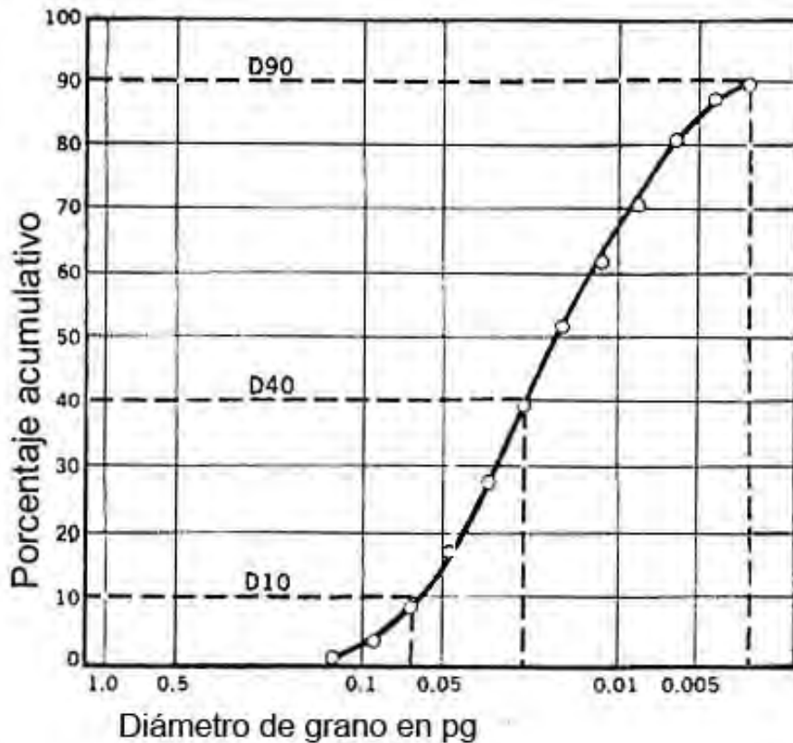
Figura 5.1 Análisis típico de Tamiz
