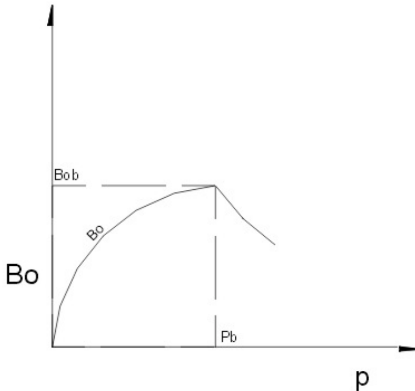
Figura 1.6 Factor de volumen del aceite vs. Presión
