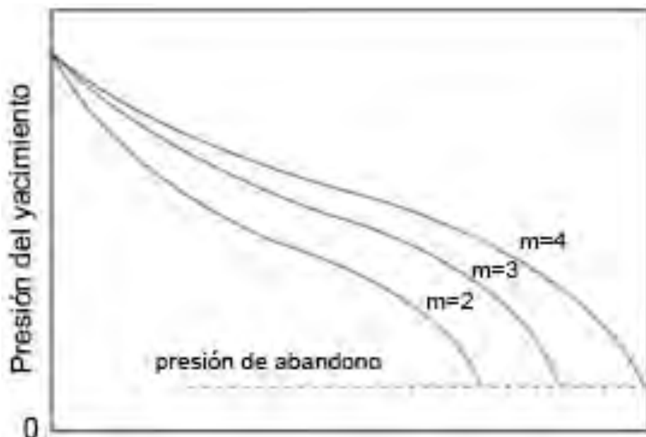
Figura 4.7 Muestra El efecto de la capa gas en la recuperación final
