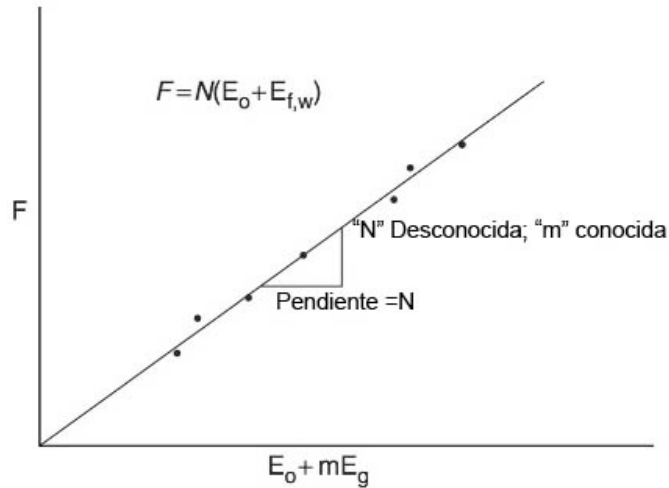
Figura 4.17 F vs. E_o + mE_g
