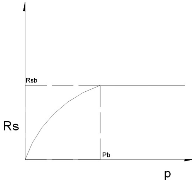
Figura 1.5 Relación de solubilidad Vs Presión
