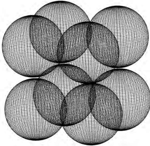
Figura 2.1 Empacamiento cúbico de esferas, tiene una porosidad de 47.64%
