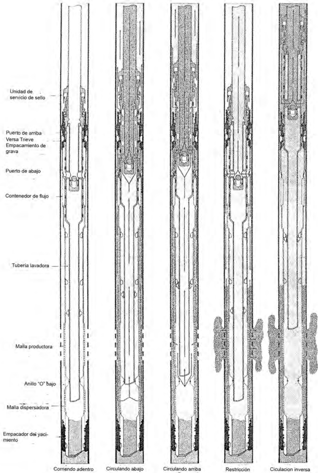
Figura 5.10 Técnica de empacamiento interno en tubería
