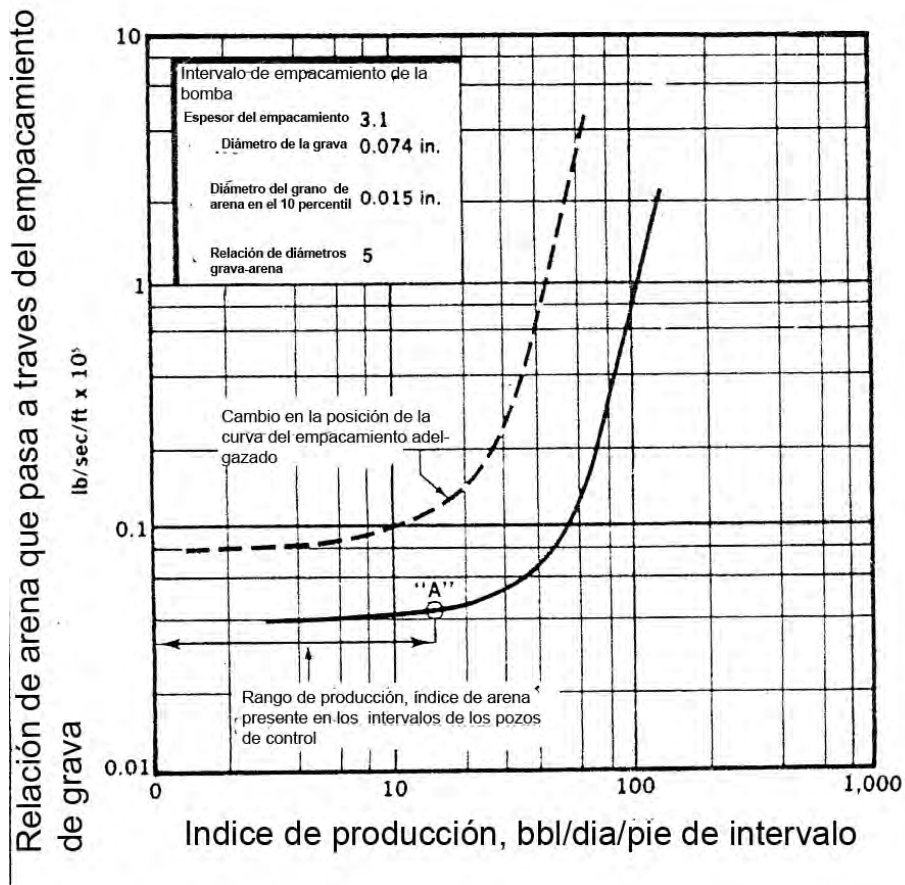
Figura 5.4 Muestra el índice de producción Vs en índice de arena que pasa a través del empacamiento de grava.
