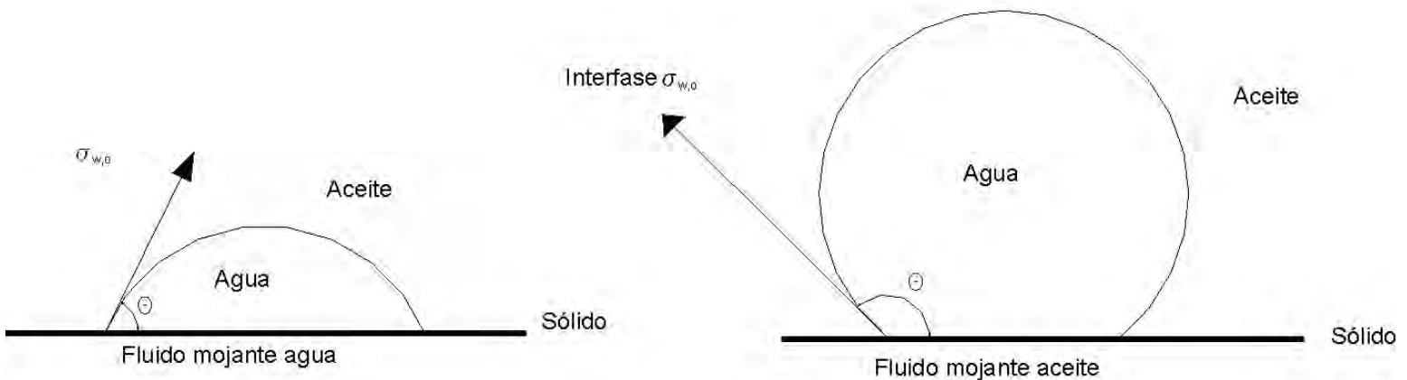
Figura 2.6 Diagrama de mojabilidad en un sistema sólido-fluido
