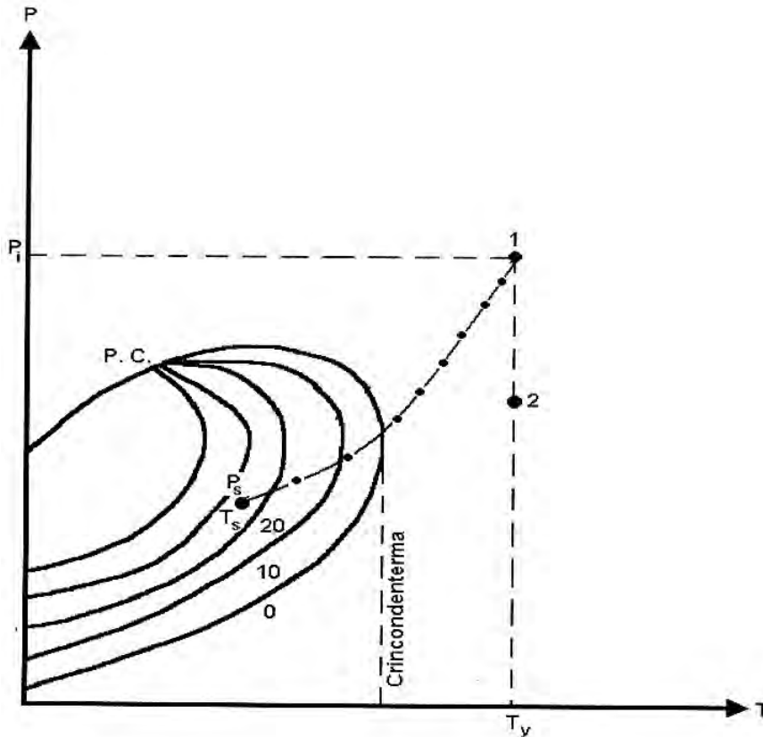
Figura 4.5 Muestra el diagrama de fases de un yacimiento de gas húmedo
