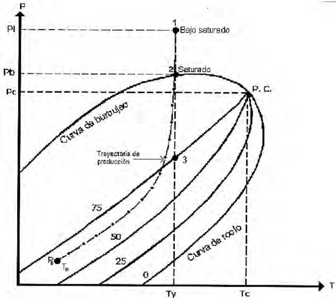
Figura 4.2 Muestra el diagrama de fases de un yacimiento de aceite y gas de bajo encogimiento
