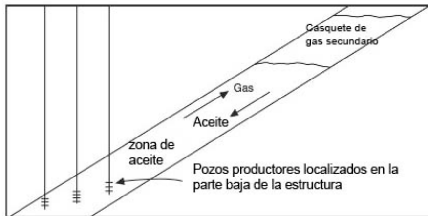
Figura 4.12 Yacimiento con segregación gravitacional
