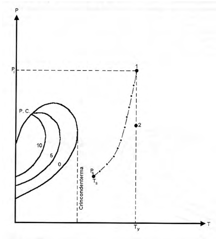
Figura 4.6 Muestra el diagrama de fases de un yacimiento de gas seco
