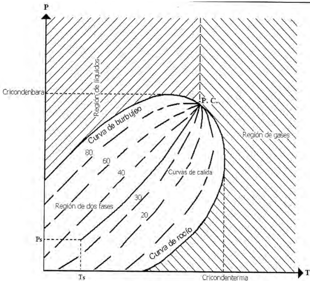
Figura 4.1 Muestra el diagrama de fases temperatura-presión.
