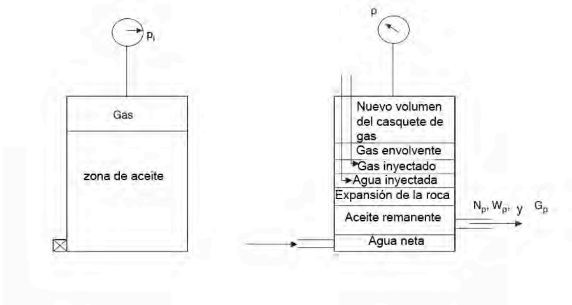
Figura 4.14 Concepto del modelo de tanque
