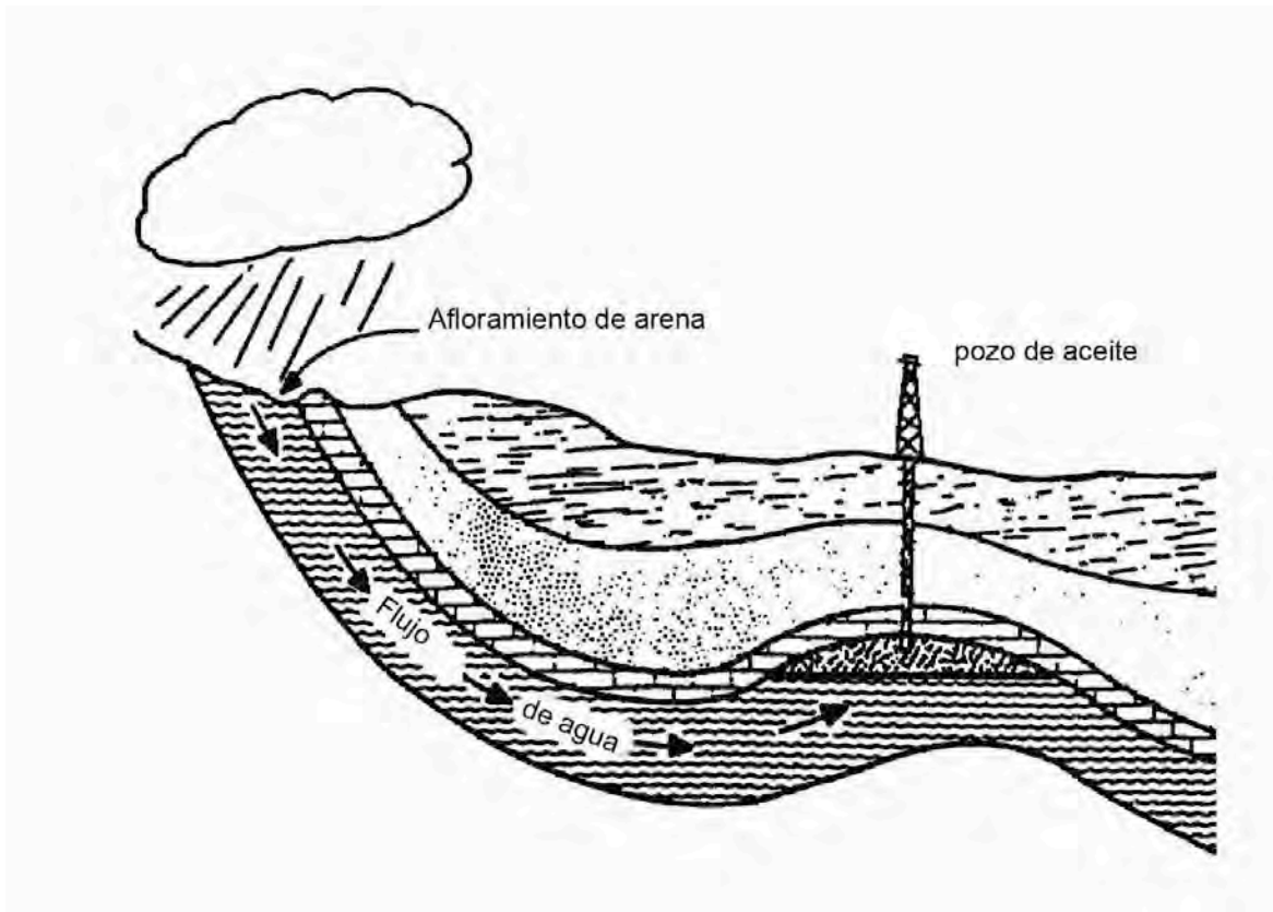
Figura 4.8 Yacimiento con empuje de agua artesiana
