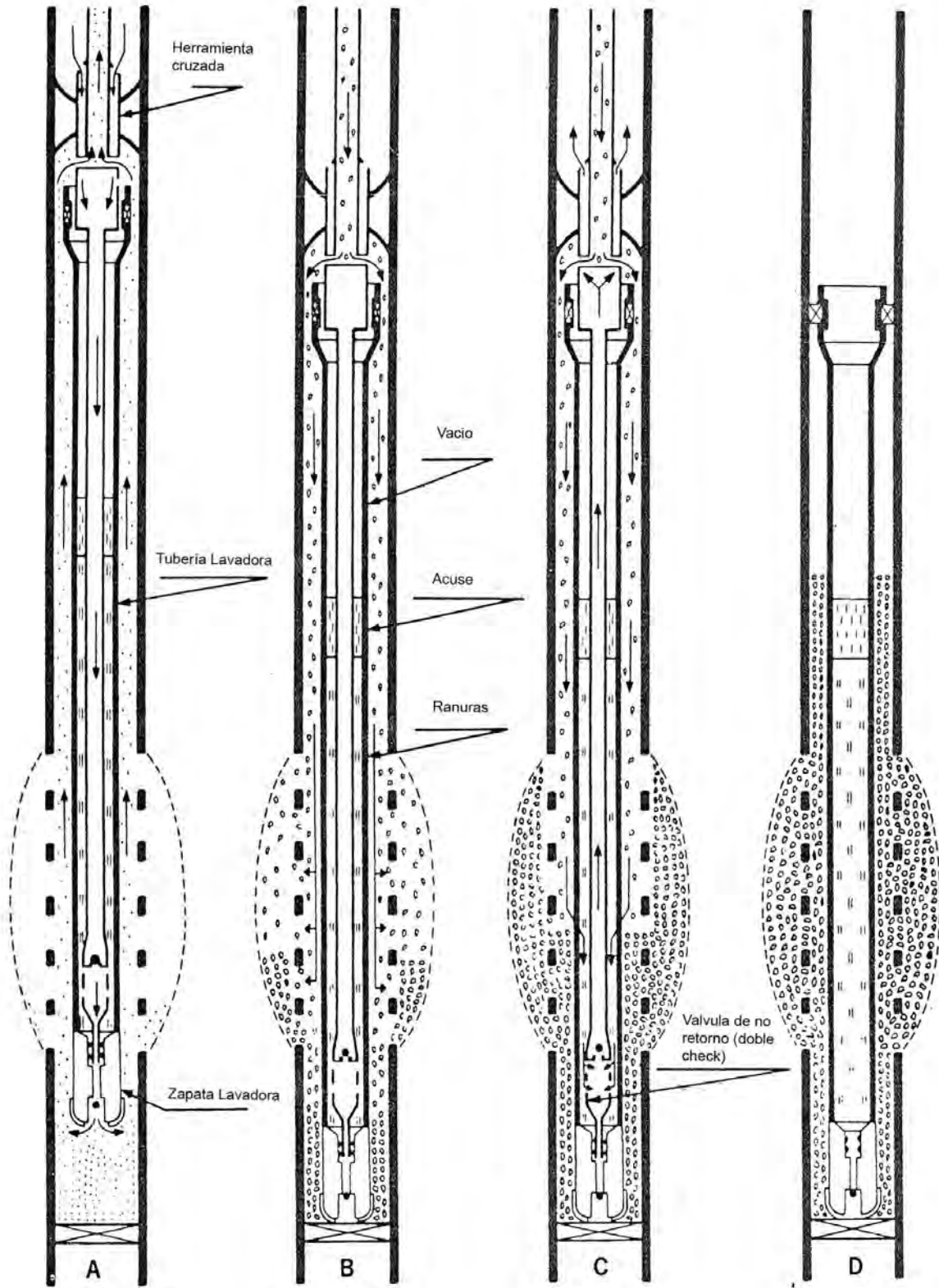
Figura 5.8 Segunda etapa de apriete del empacamiento en dos etapas
