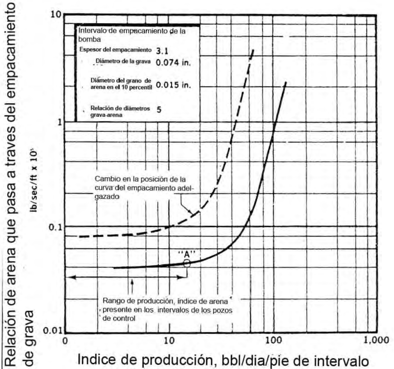
Figura 5.5 Movimiento dentro del empacamiento Vs La dinámica del flujo
