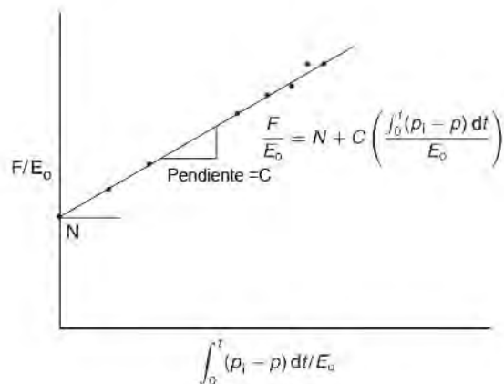
Figura 4.20 Muestra la determinación gráfica de N y C
