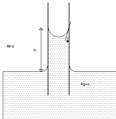
Figura 2.5 Líquido mojante
