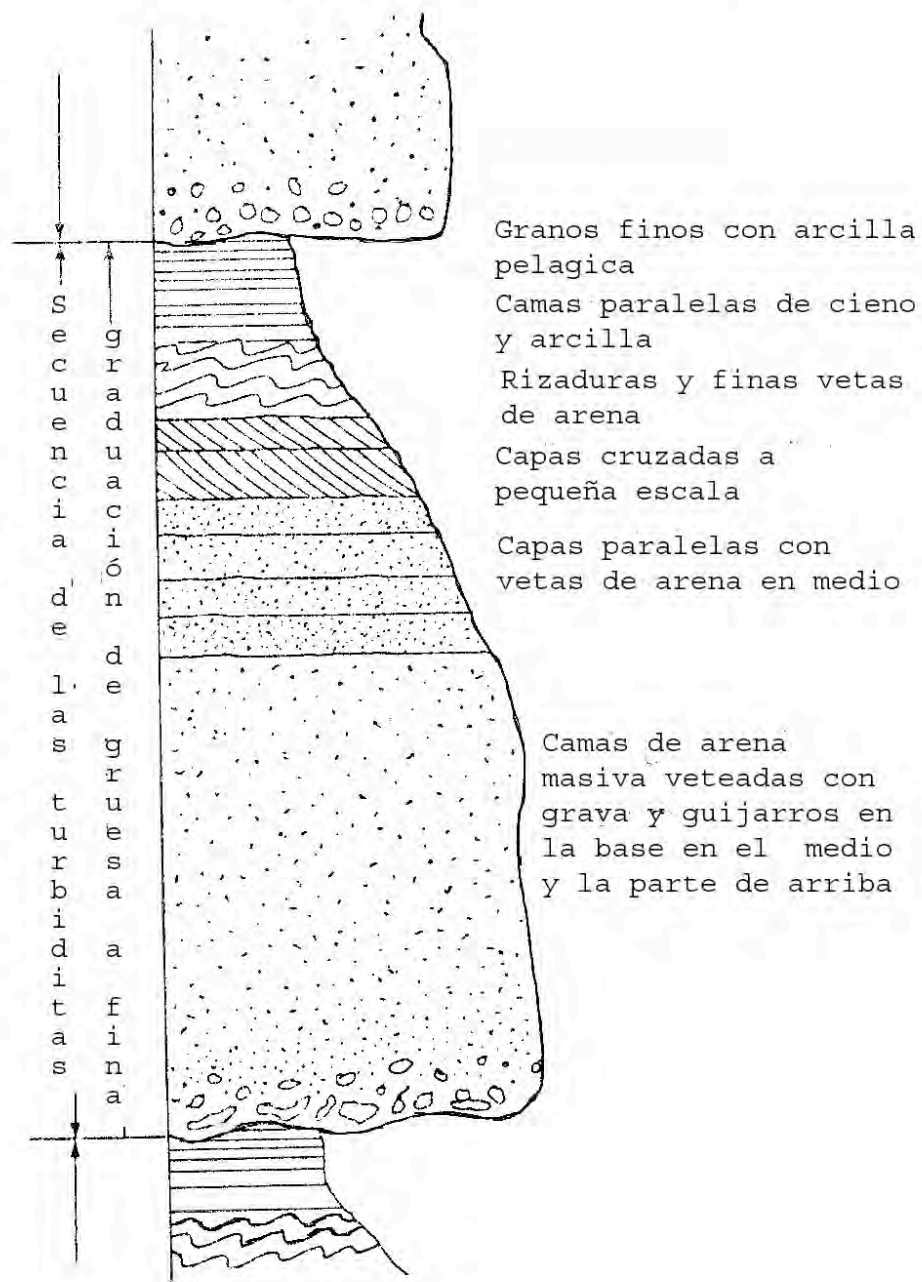
Figura 3.3 Diagrama de una típica corriente de depósito de turbiditas. El rango de las secuencias en los espesores es de menos de un metro a 3 ó 4 metros. No todas las subunidades se presentan en cada secuencia y el patrón exacto de secuencias varía con la pendiente y hay un abanico de ambiente hasta el plano abisal. Las secuencias individuales pueden ser localizadas a muchos kilómetros.
