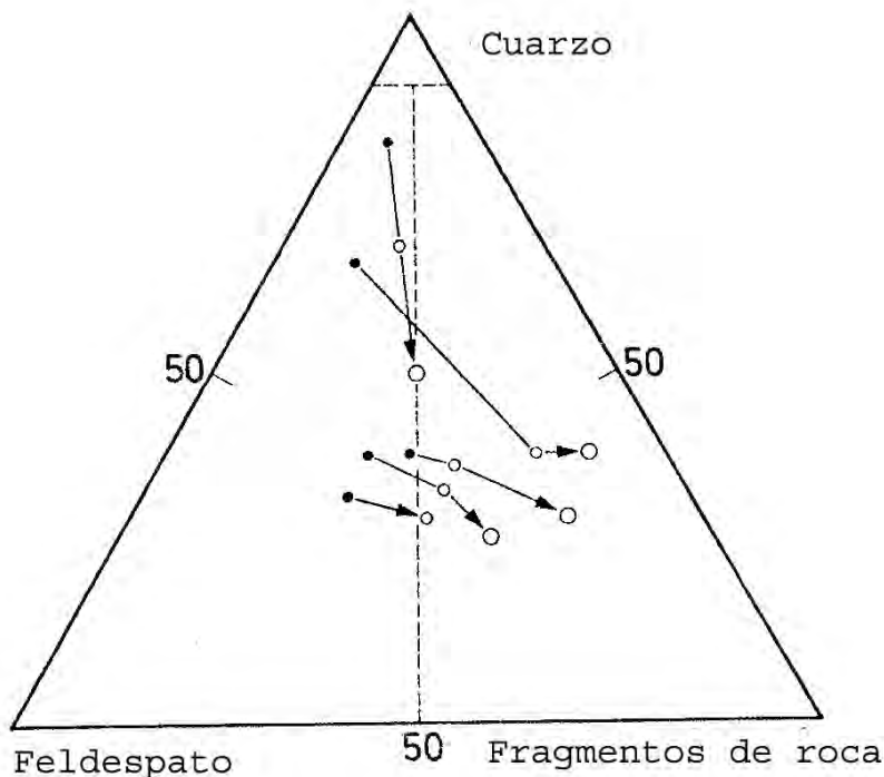
Figura 3.5 La grafica muestra la clasificación de las arenas, cada flecha conecta muestras de la misma secuencia, las dirección de la flecha va de lo más fino a lo más grueso.
