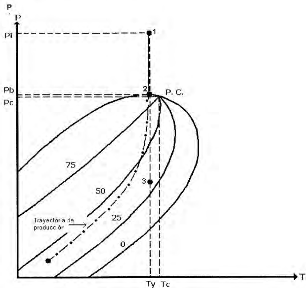
Figura 4.3 Muestra el diagrama de fases de un yacimiento de aceite y gas de alto encogimiento
