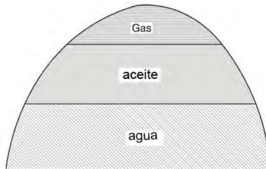
Figura 4.10 Muestra la distribución inicial de fluidos en el yacimiento.
