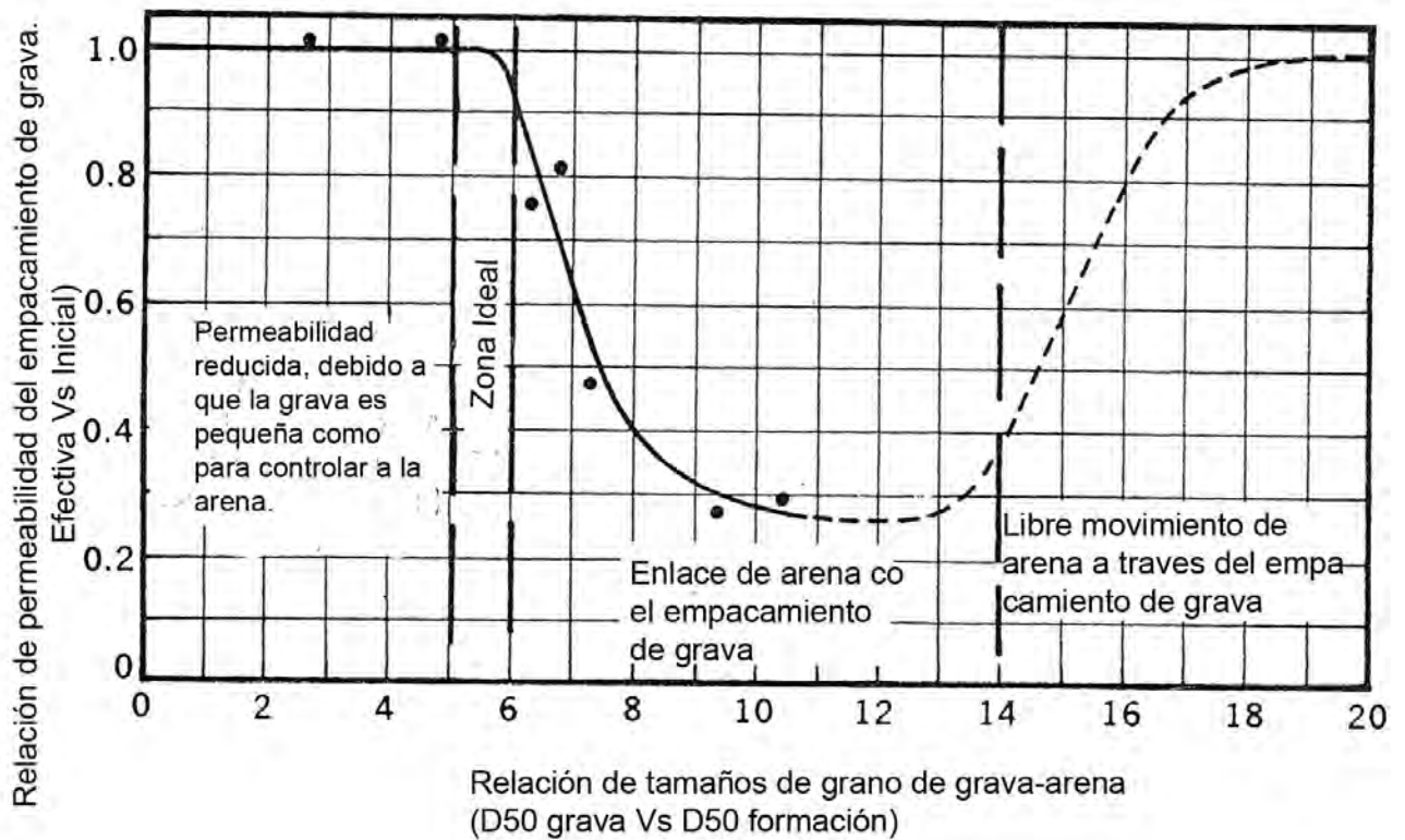
Figura 5.2 Efecto de la relación grava-arena en la permeabilidad del empacamiento de grava.
