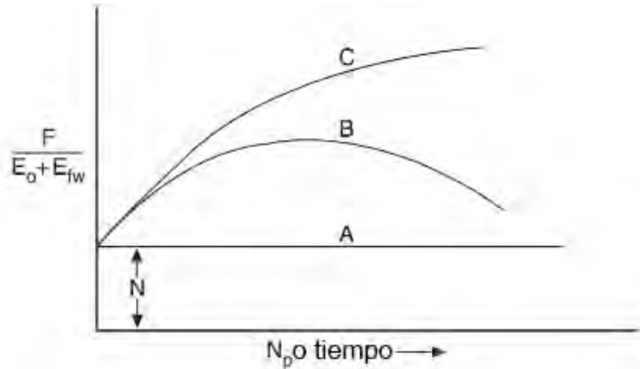
Figura 4.15 Clasificación del yacimiento
