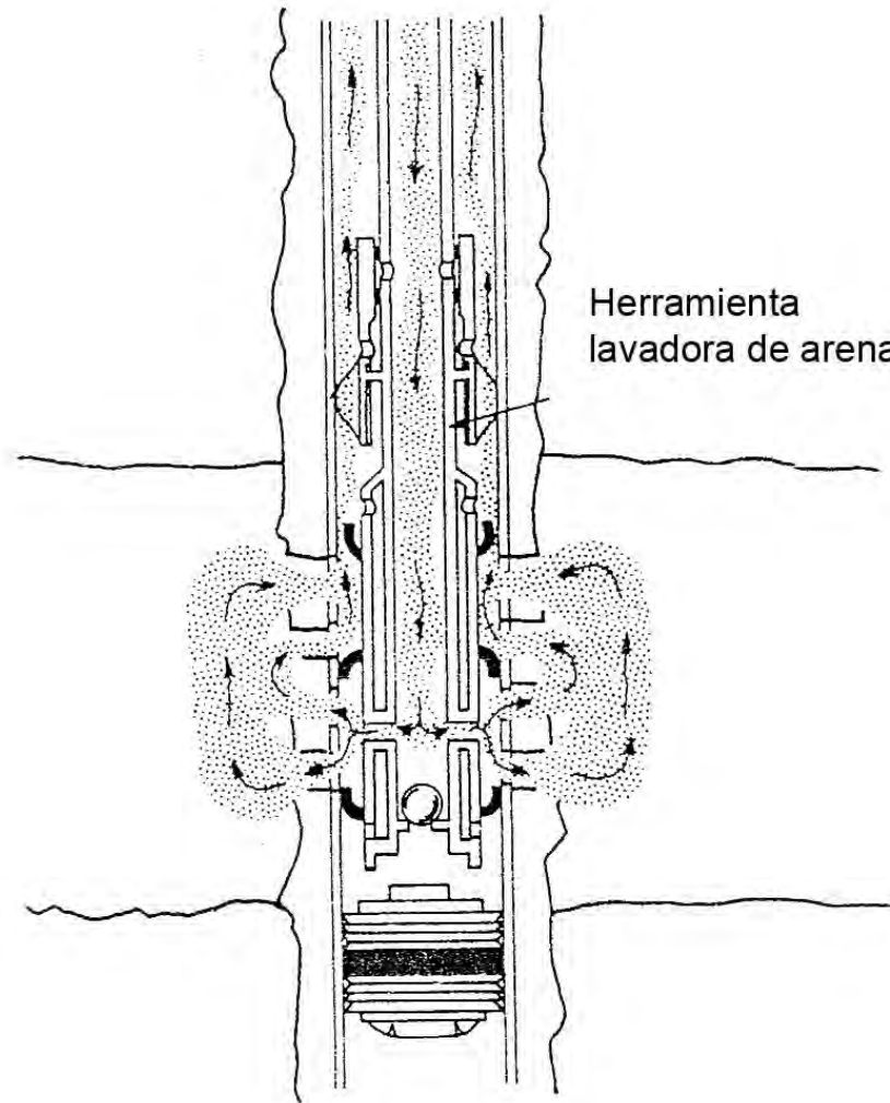
Figura 5.7 Herramienta lavadora tipo taza
