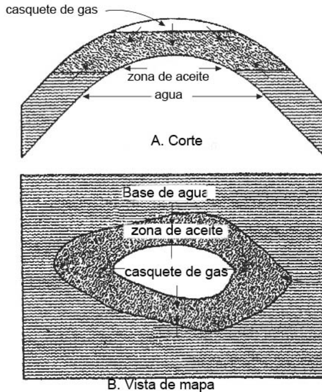
Figura 4.13 Muestra una combinación de mecanismos de empuje
