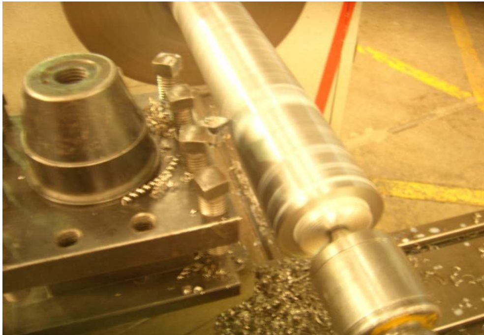
Figura 4.10 Barra hueca de acero.
