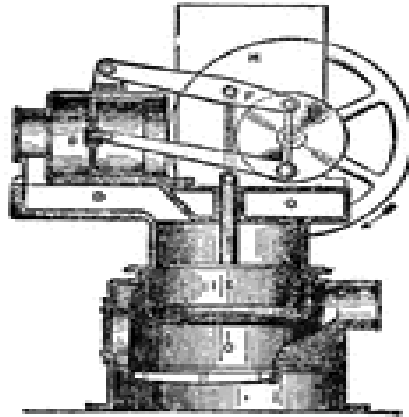
Figura 1.5 Motor Robinson
