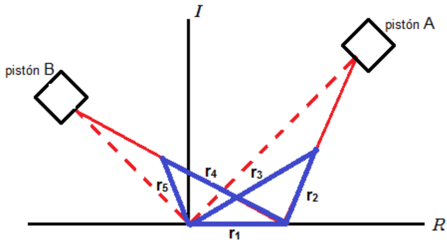
Figura 3.8 Cadena cinemática con el centro de masa de las bielas.
