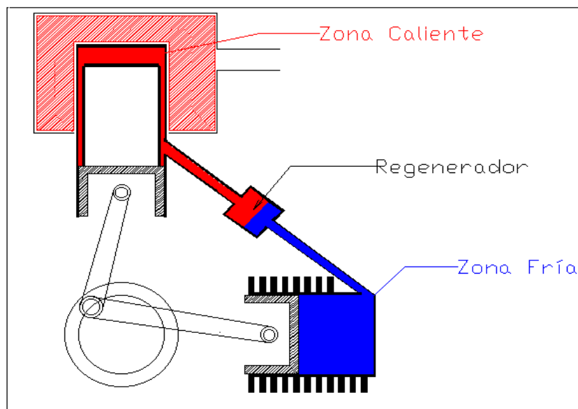
Figura 1.14 Motor Stirling tipo alfa. Fuente: http://personales.able.es/jgros/alfa.htm .
