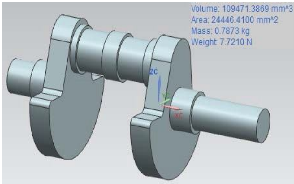
Figura 4.27 Cigüeñal de acero.
