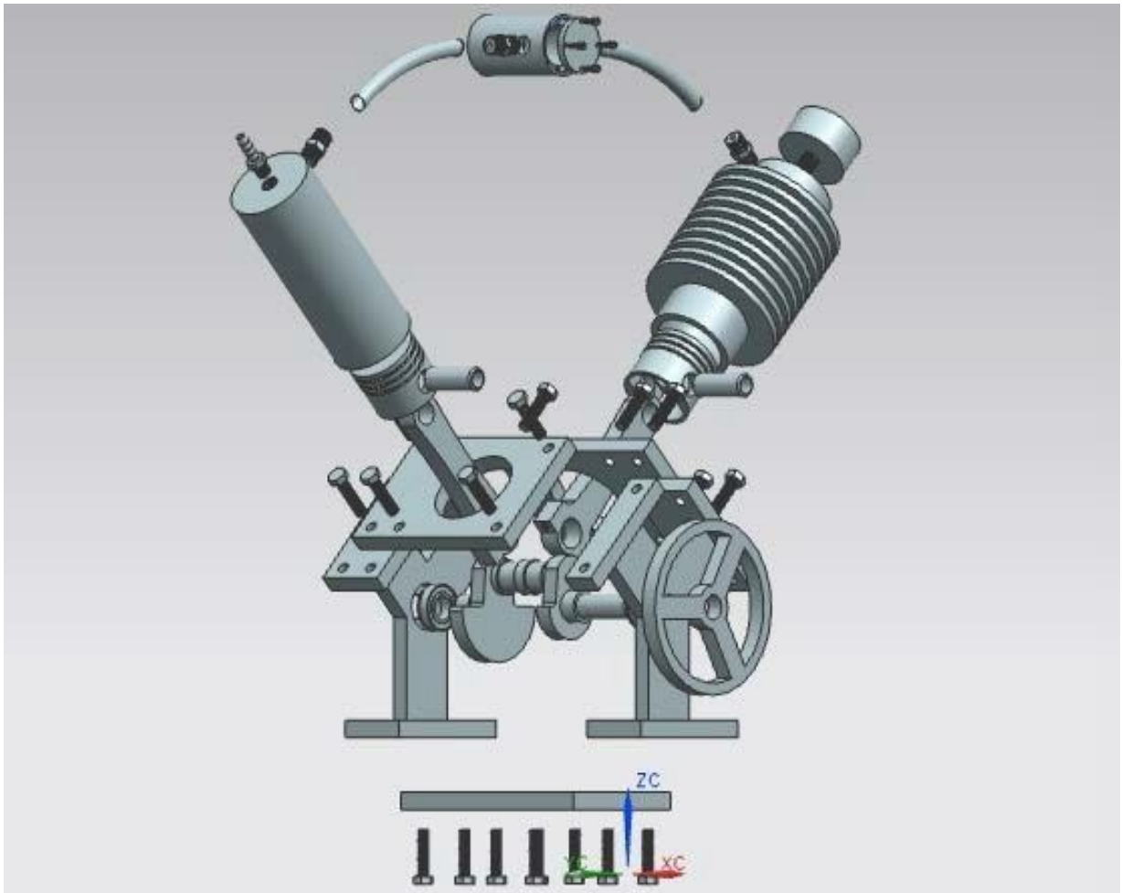
Figura 4.2 Componentes del motor Stirling diseñado.
