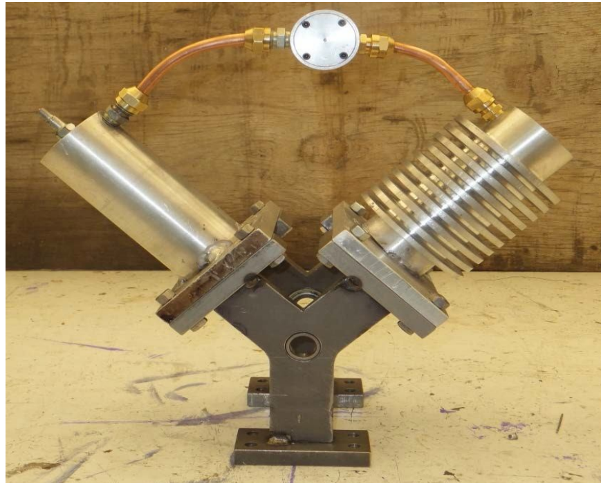
Figura 4.46. Ensamble de tubería de conexión.
