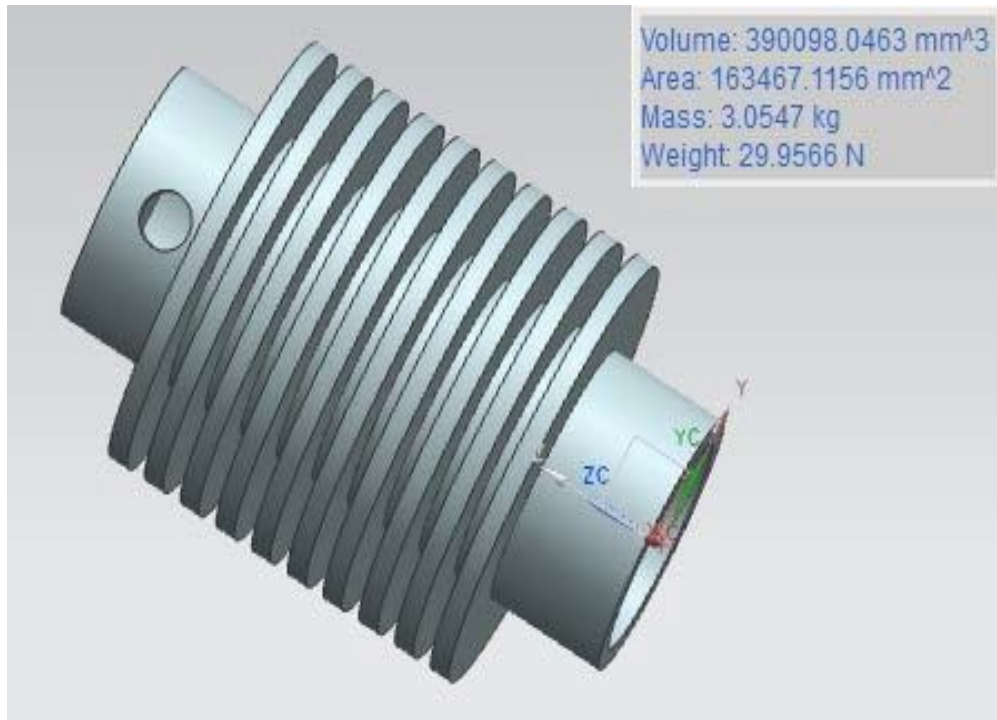
Figura 4.3 Cilindro de enfriamiento.
