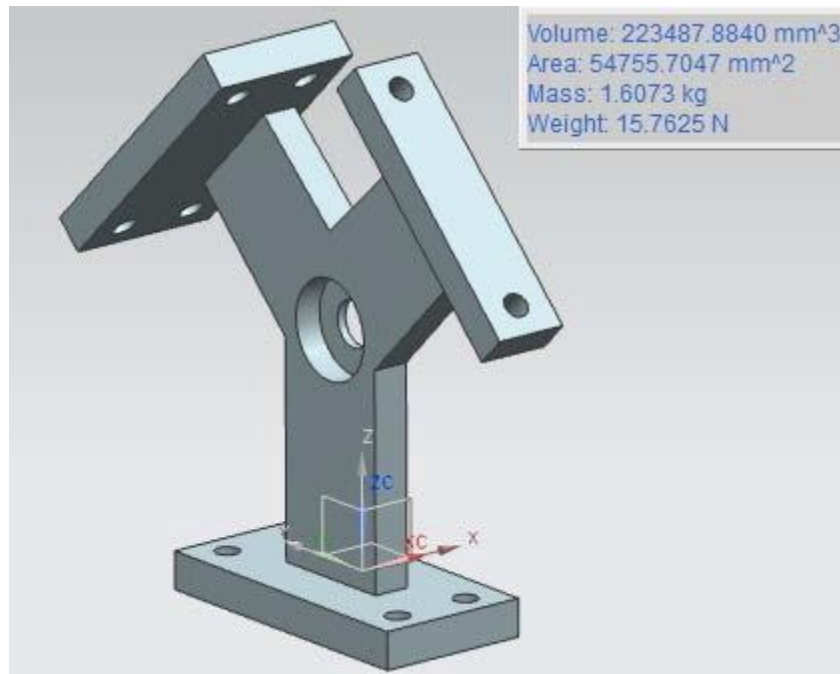
Figura 4.39. Base del motor en V.
