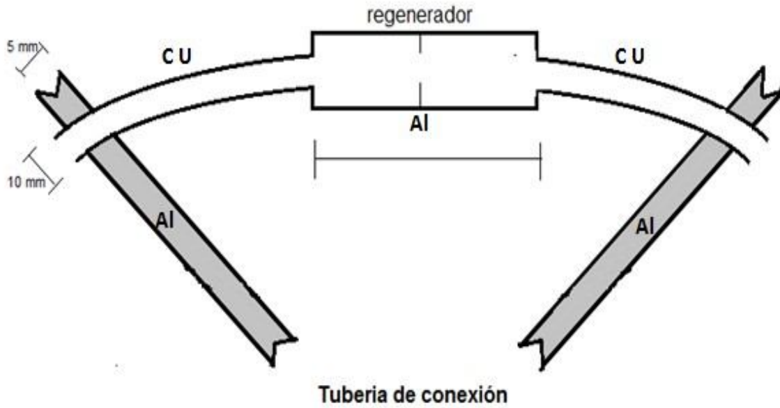
Figura 3.4 Tubería de conexión.
