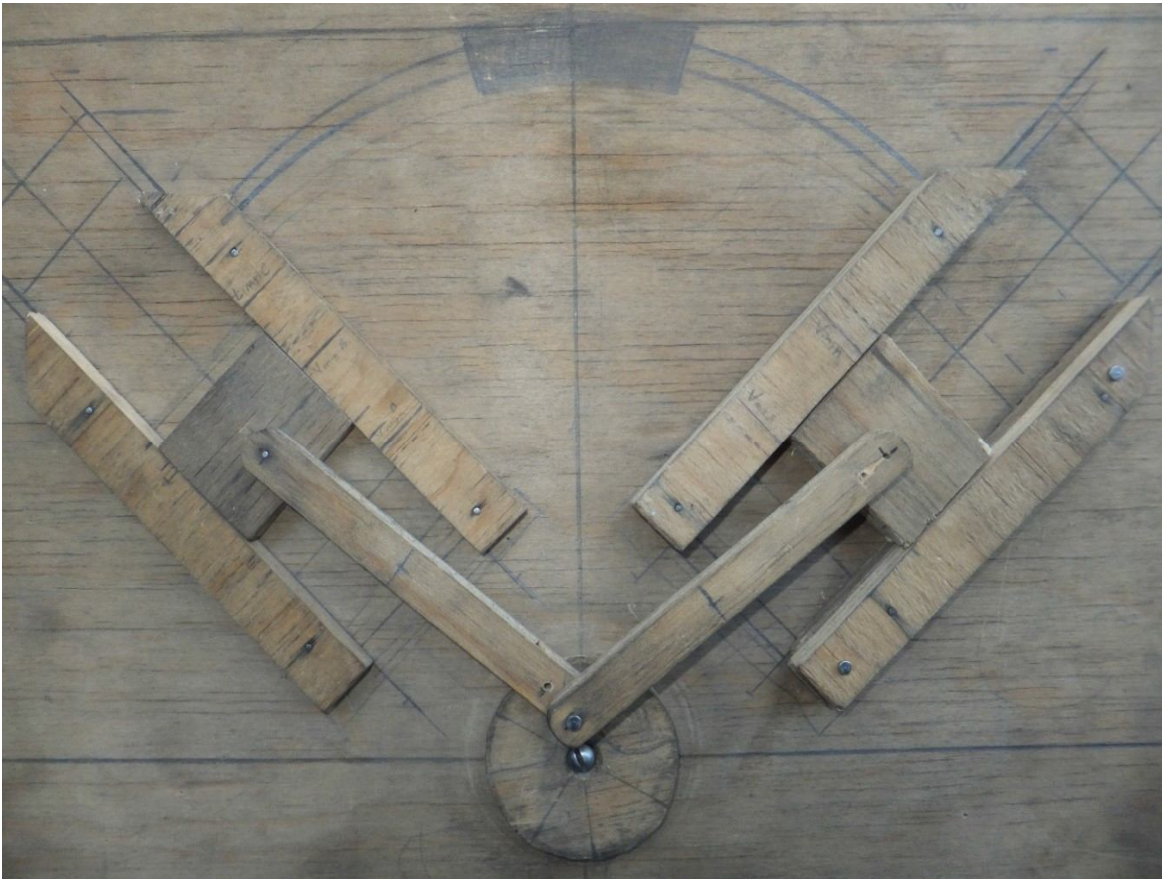
Figura 3.1 Motor Stirling tipo alfa en modelo en madera.
