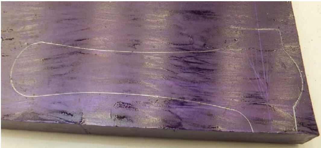
Figura 4.24 Plano de la biela marcado sobre placa de aluminio.
