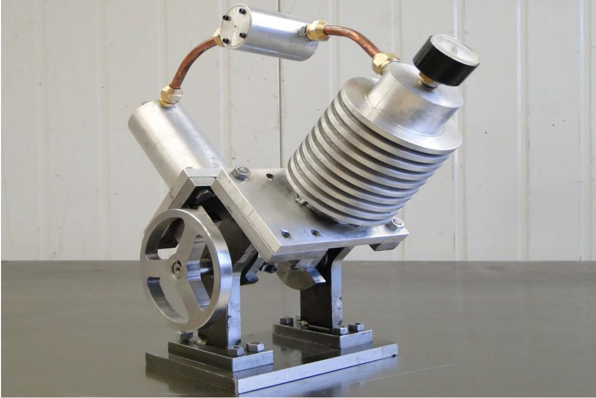
Figura 4.53. Motor ensamblado vista lateral izquierda.
