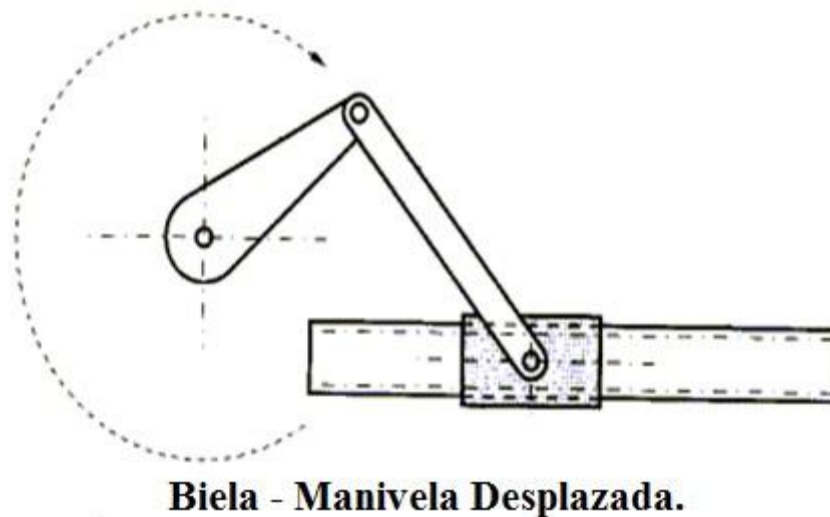
Figura 2.13 Mecanismo biela-manivela desplazada.
