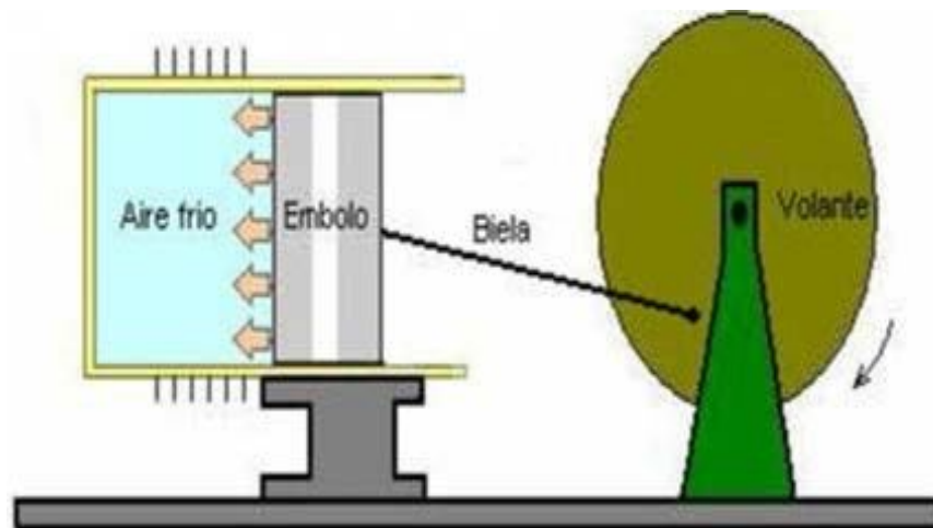
Fig.1.13 Conversión de la compresión del gas en movimiento. (1)
