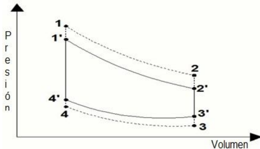
Figura 2.14 Efectos de la transferencia imperfecta de calor.
