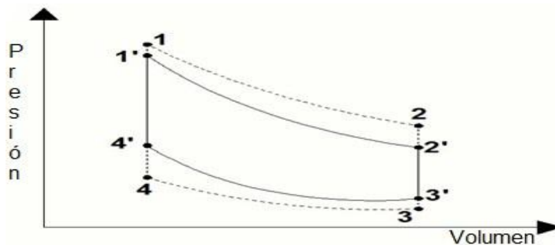
Figura 2.16 Efectos de fugas del fluido de trabajo.
