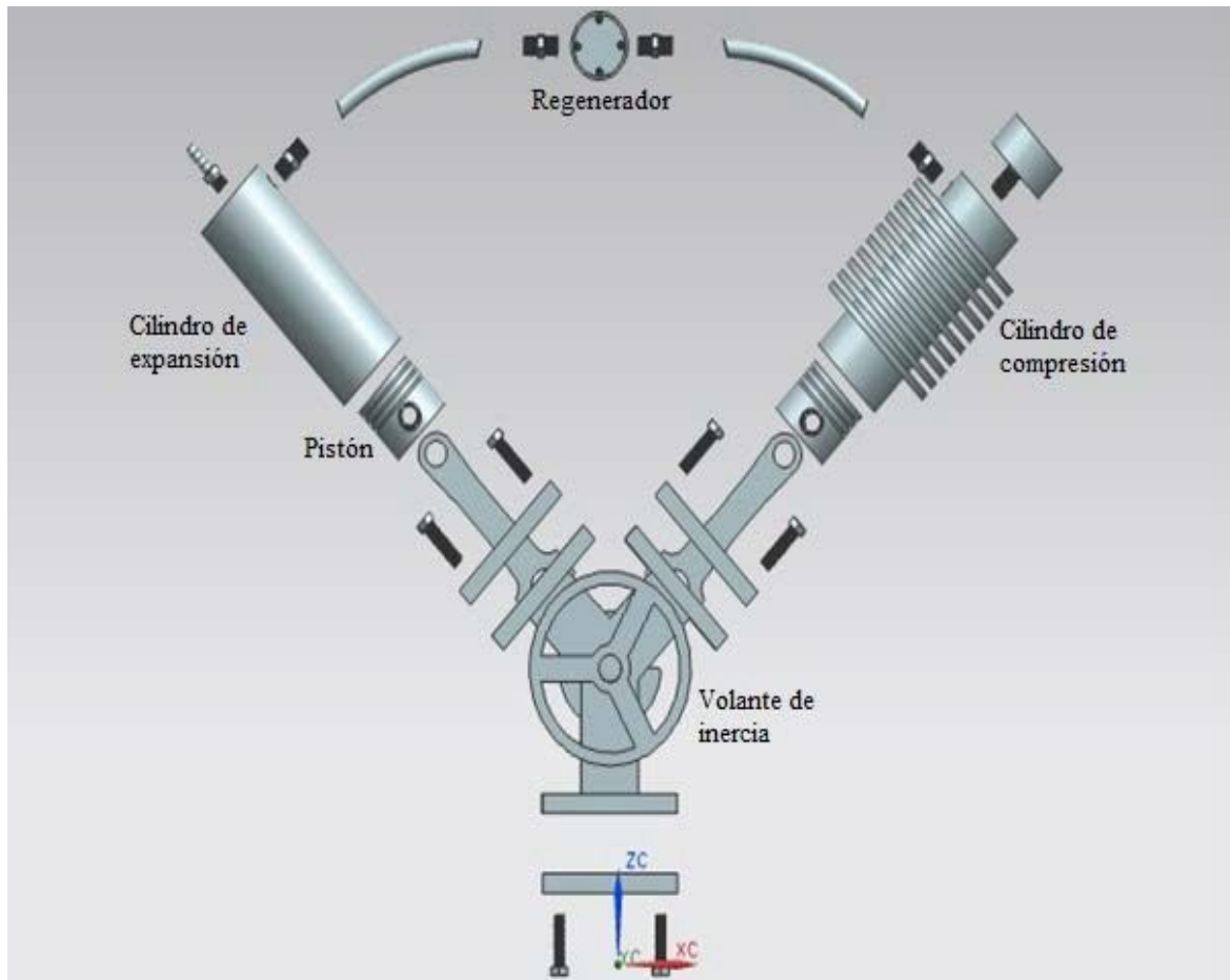
Figura 4.1 Componentes del motor Stirling propuesto.
