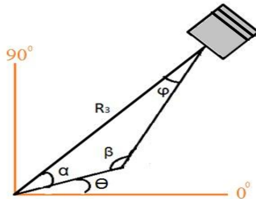
Figura 3.10 Ángulos del mecanismo.
