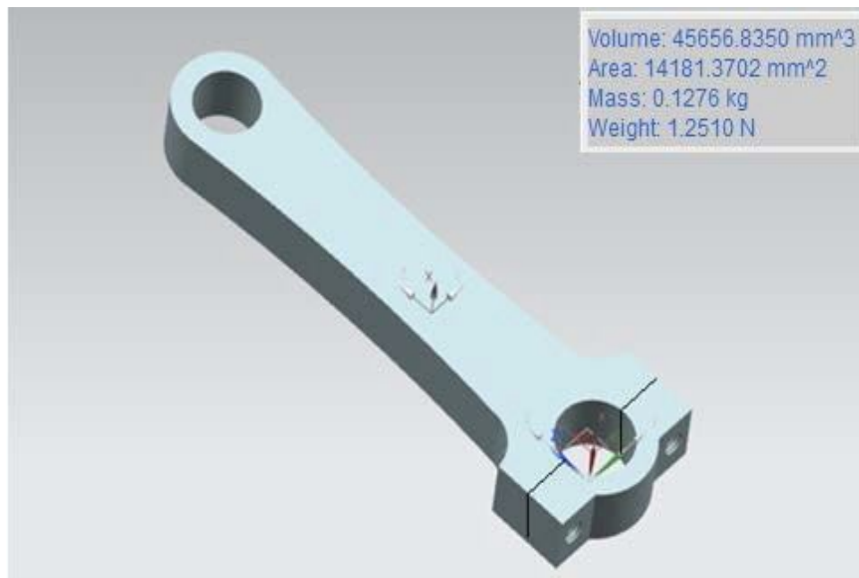
Figura 4.23 Biela de aluminio.
