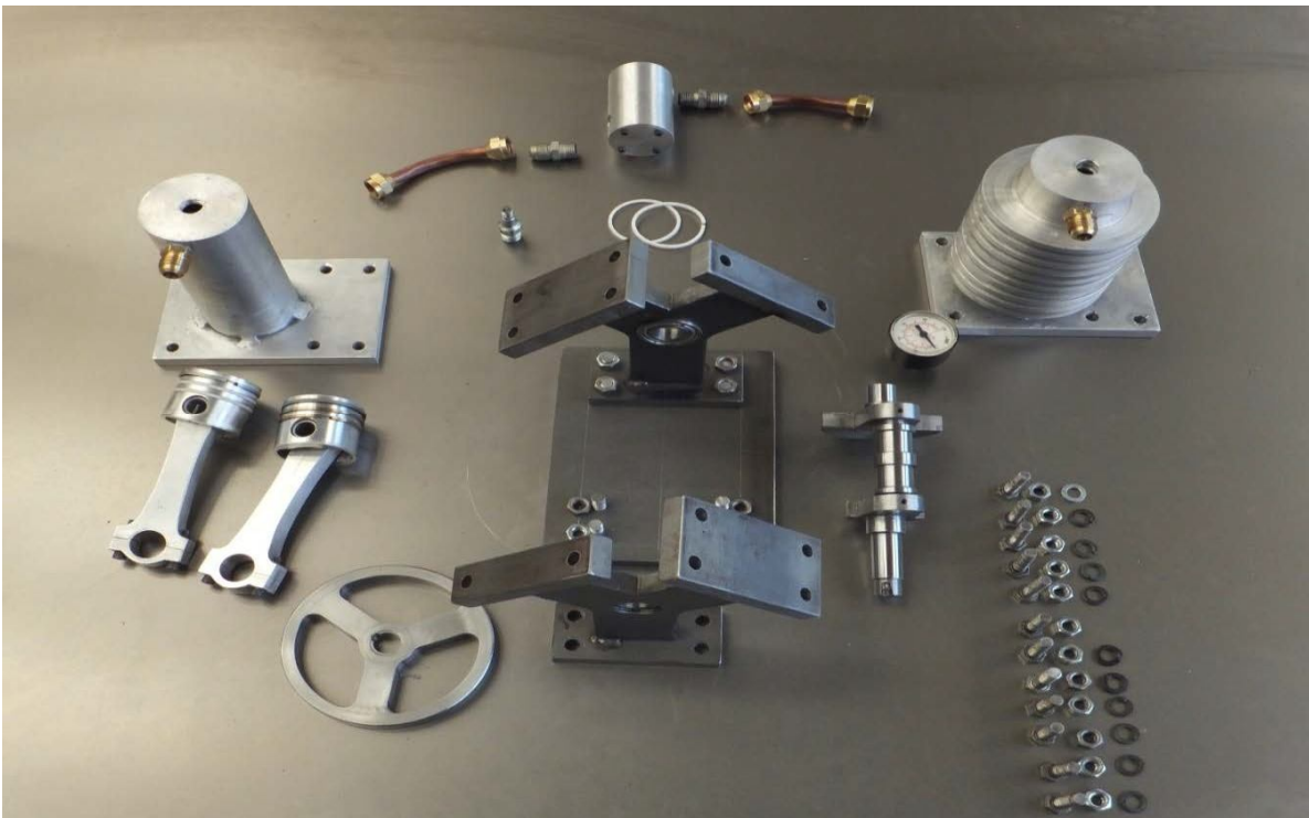
Figura 4.50. Despiece del motor Strling tipo alfa.
