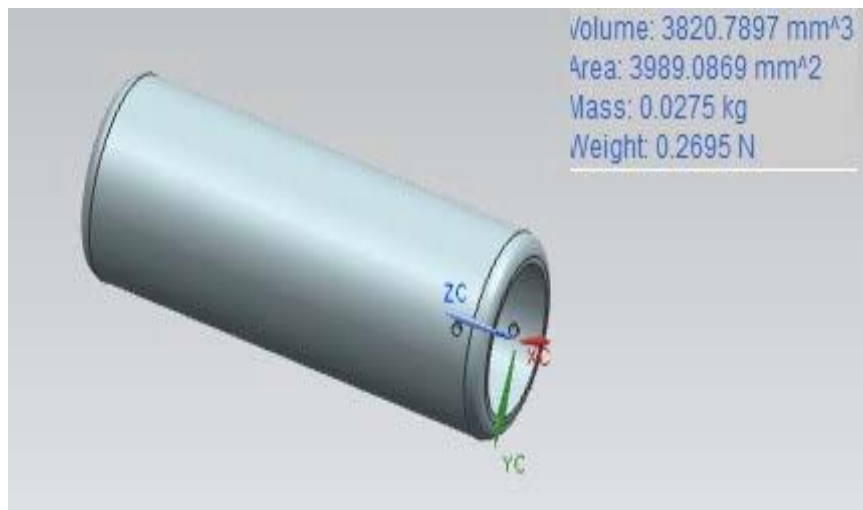
Figura 4.34. Bulón.
