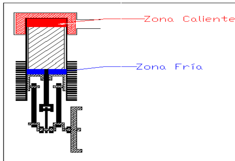
Figura 1.15 Motor Stirling tipo beta. Fuente: http://personales.able.es/jgros/beta.htm .
