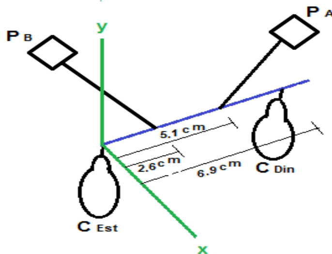
Figura 3.9 Diagrama de cuerpo libre.
