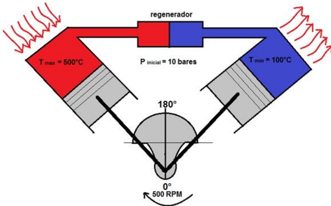
Figura 3.2. Diagrama del sistema.
