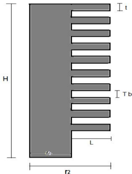
Figura 3.5 Cilindro aletado.
