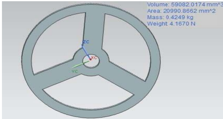
Figura 4.31. Volante de inercia.
