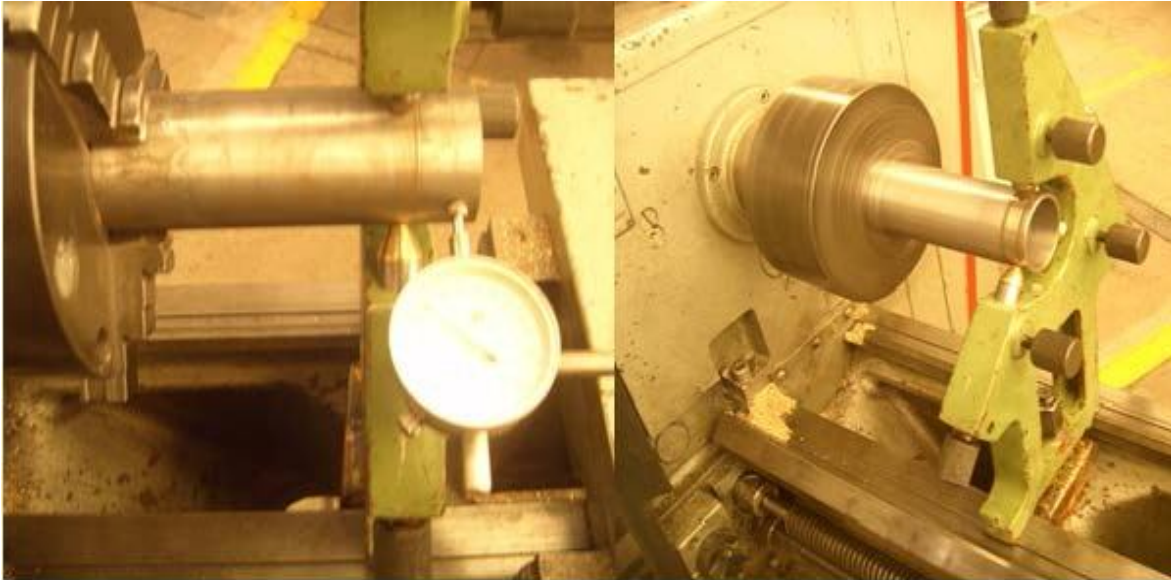
Figura 4.11 Maquinado con luneta fija.
