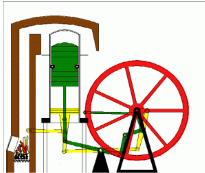
Figura 1.1 Diseño del primer motor Stirling. Fuente: www.moebius-bcn.com motor Stirling.
