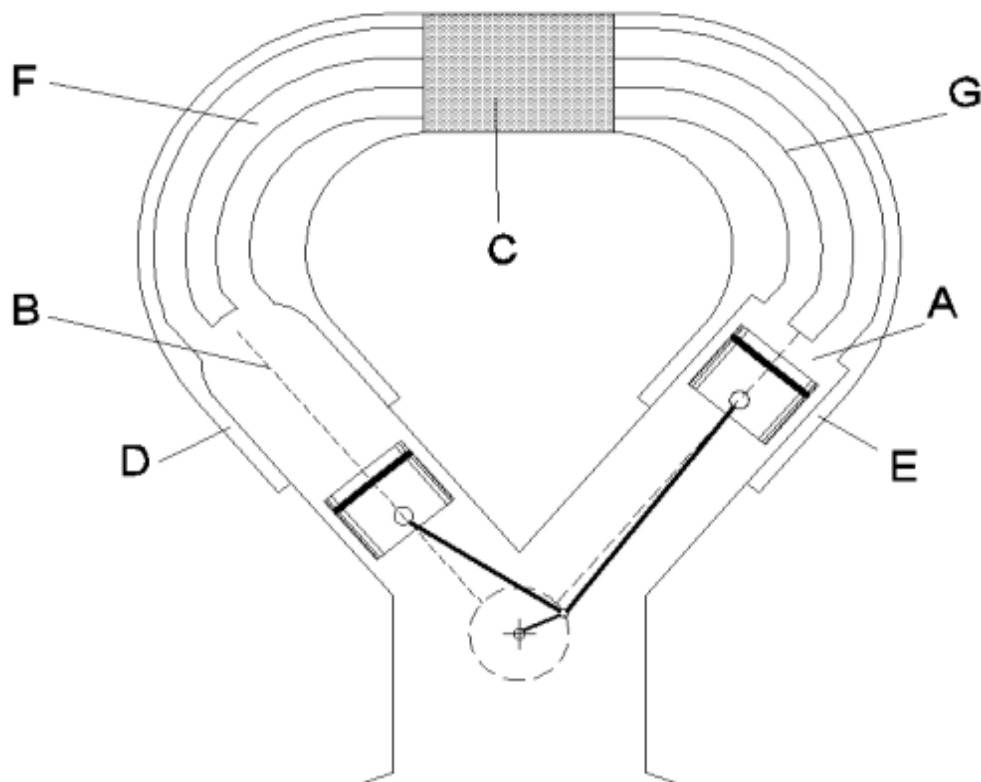
Figura 2.1 Motor Stirling tipo Alfa.
