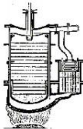
Figura 1.3 Mejoras al motor de doble-efecto en 1840. Fuente: www.biblio-sepi.esimez.ipn.mx/.../
