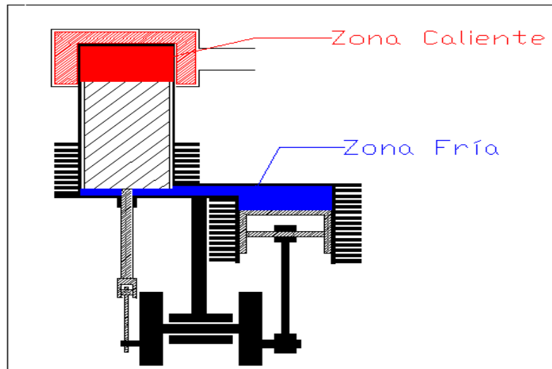
Figura 1.16 Motor Stirling tipo gamma Fuente: http://personales.able.es/jgros/gamma.htm .
