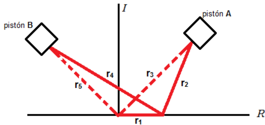
Figura 3.7 Cadena cinemática del mecanismo.
