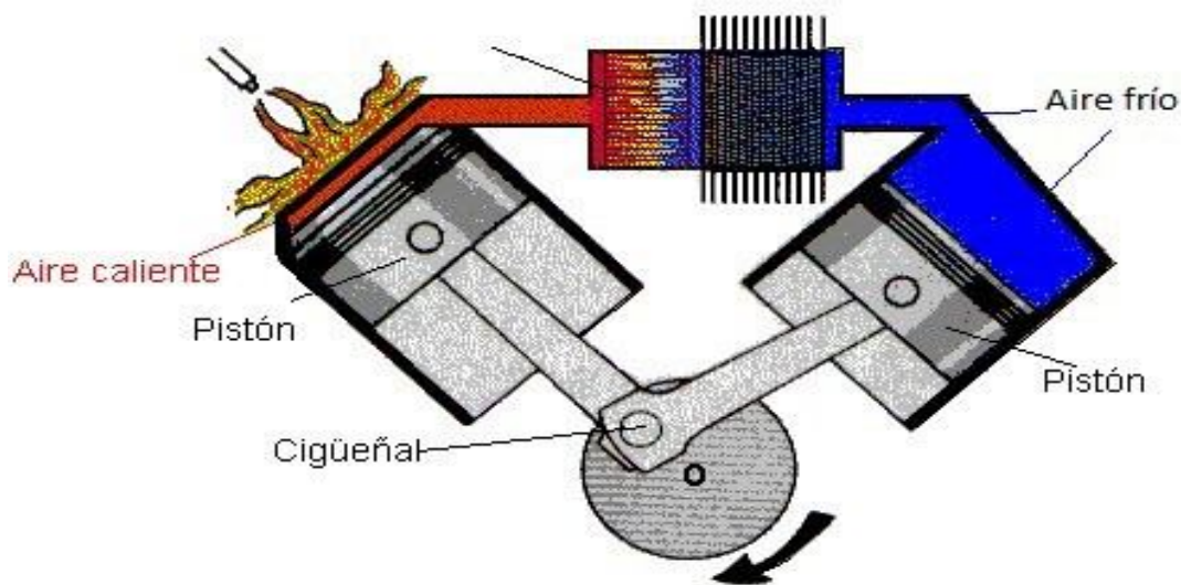
Figura 1.9 Funcionamiento del motor Stirling Fuente: http://members.tripod.de/peterfette/howdo.htm
