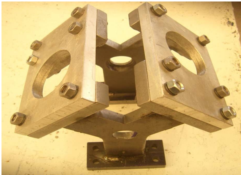
Figura 4.41. Base ensamblada del motor.
