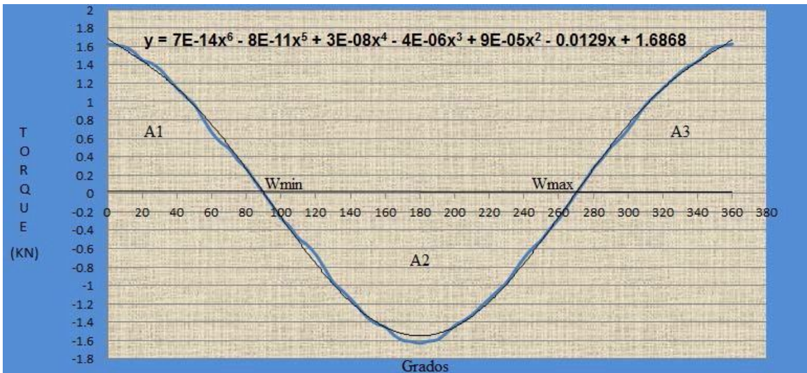
Gráfica 3.3. Polinomio característico de la función de torque.
