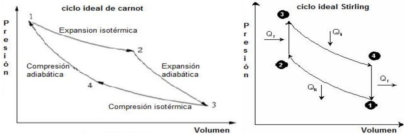
Figura 2.18 Ciclo de Carnot P-V vs Ciclo Stirling P-V.
