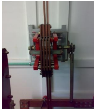
Figura. 2-26 Seccionadores de operación sin carga, para el bus de salida positivo y negativo.
