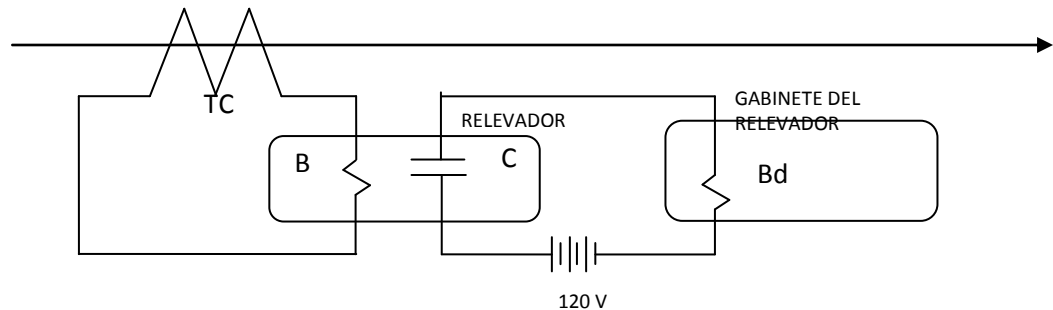
Figura. 3-5 Relevador.
