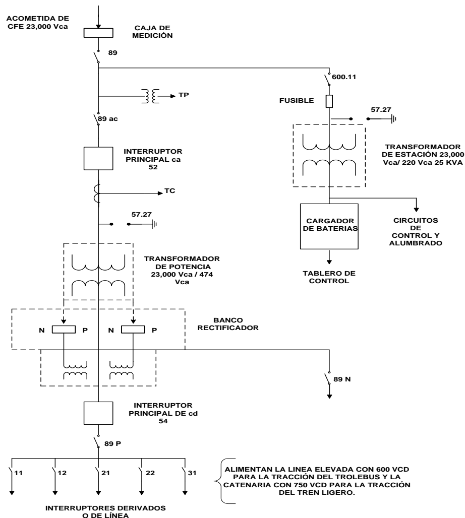
Figura. 3-12 Diagrama Unifilar de una Subestación Rectificadora para Trolebús y Tren Ligero.
