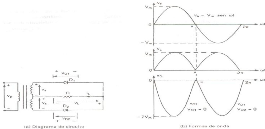
Figura. 2-3 Rectificador de onda completa con transformador con derivación central.
