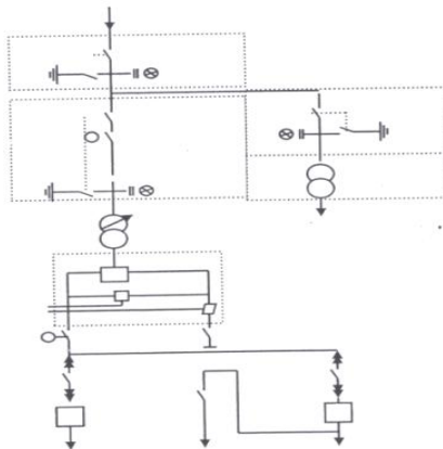
Figura. 2-10 Diagrama de Subestación tipo "TT".
