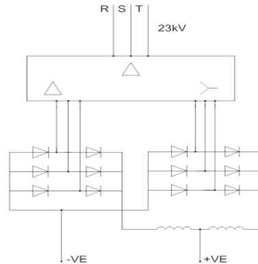
Figura. 2-16 Diagrama del Rectificador ENGLISH ELECTRIC 12 pulsos.
