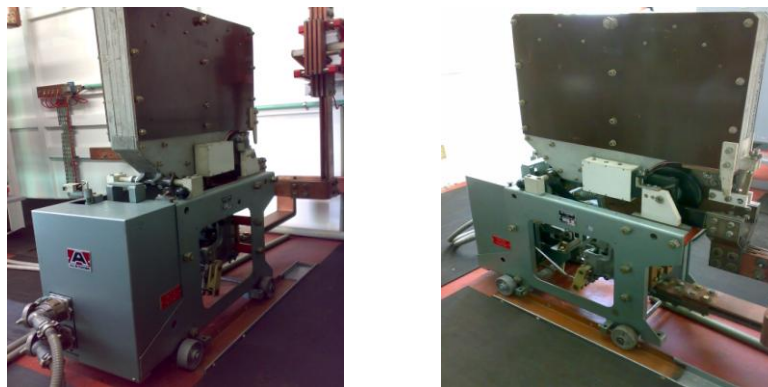
Figura. 3-9 Interruptor UR-54.
