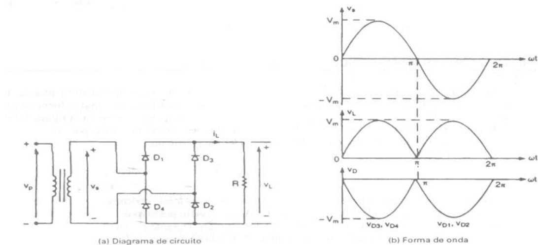
Figura. 2-4 Rectificador puente de onda completa.
