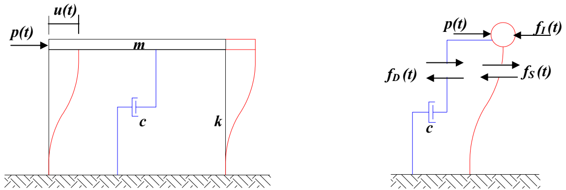
Sistema de un grado de libertad
