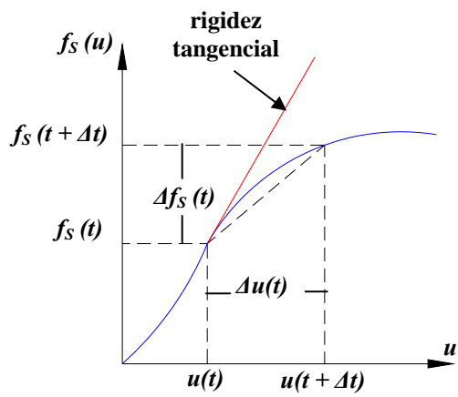
Rigidez no lineal
