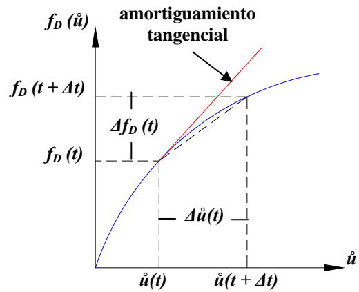
Amortiguamiento no lineal
