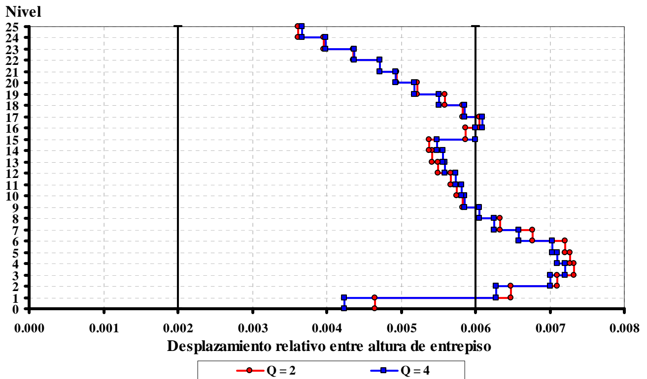
Fig 5.11 Comparación de relaciones de desplazamientos horizontal relativo inelásticos entre altura de entrepiso del marco del eje B del edificio de 25 niveles para Q= 2 y 4 con \gamma_p \leq 0.002 y 0.006
