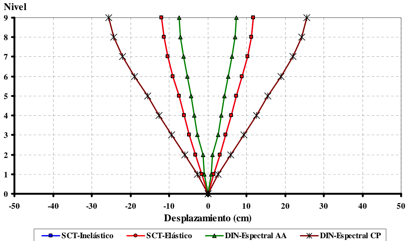
Fig 4.9 Desplazamientos horizontales máximos totales del edificio de 9 niveles para Q=2 con \gamma_p \leq 0.004 y 0.012
