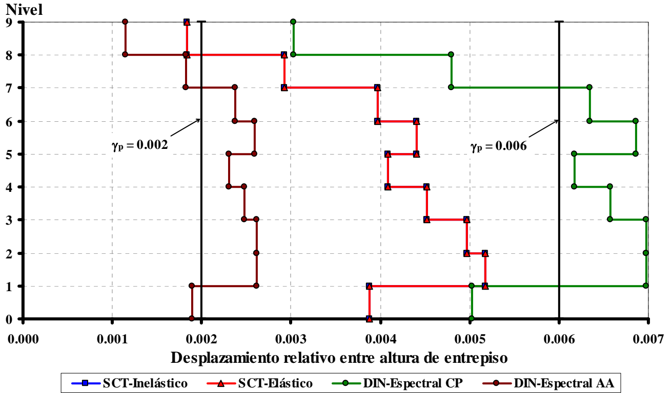
Fig 4.26 Relaciones de desplazamientos horizontales relativos entre altura de entrepiso del marco del eje B del edificio de 9 niveles para Q=2 con \gamma_p \leq 0.002 y 0.006
