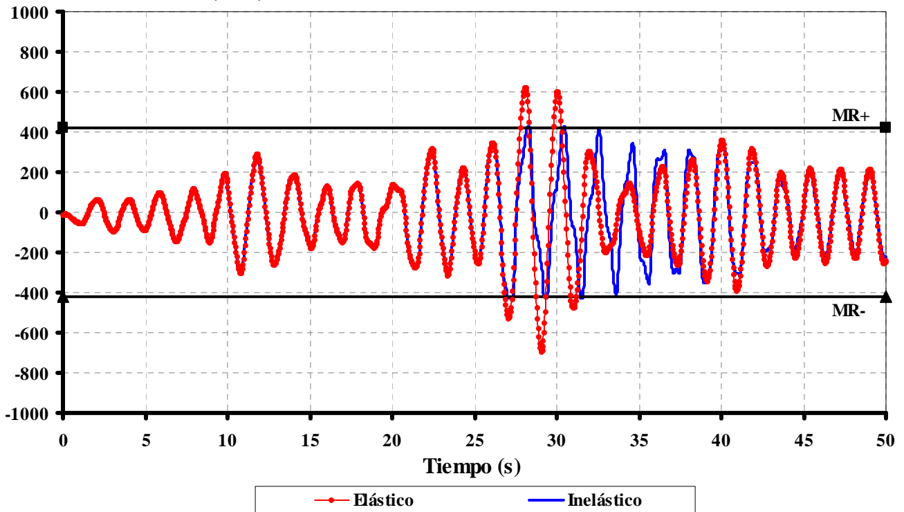
Fig 4.55 Historia de momentos flexionantes y resistencias del extremo izquierdo de la viga 1 del marco del eje B del edificio de 25 niveles para Q=2 y \gamma_p \leq 0.004
