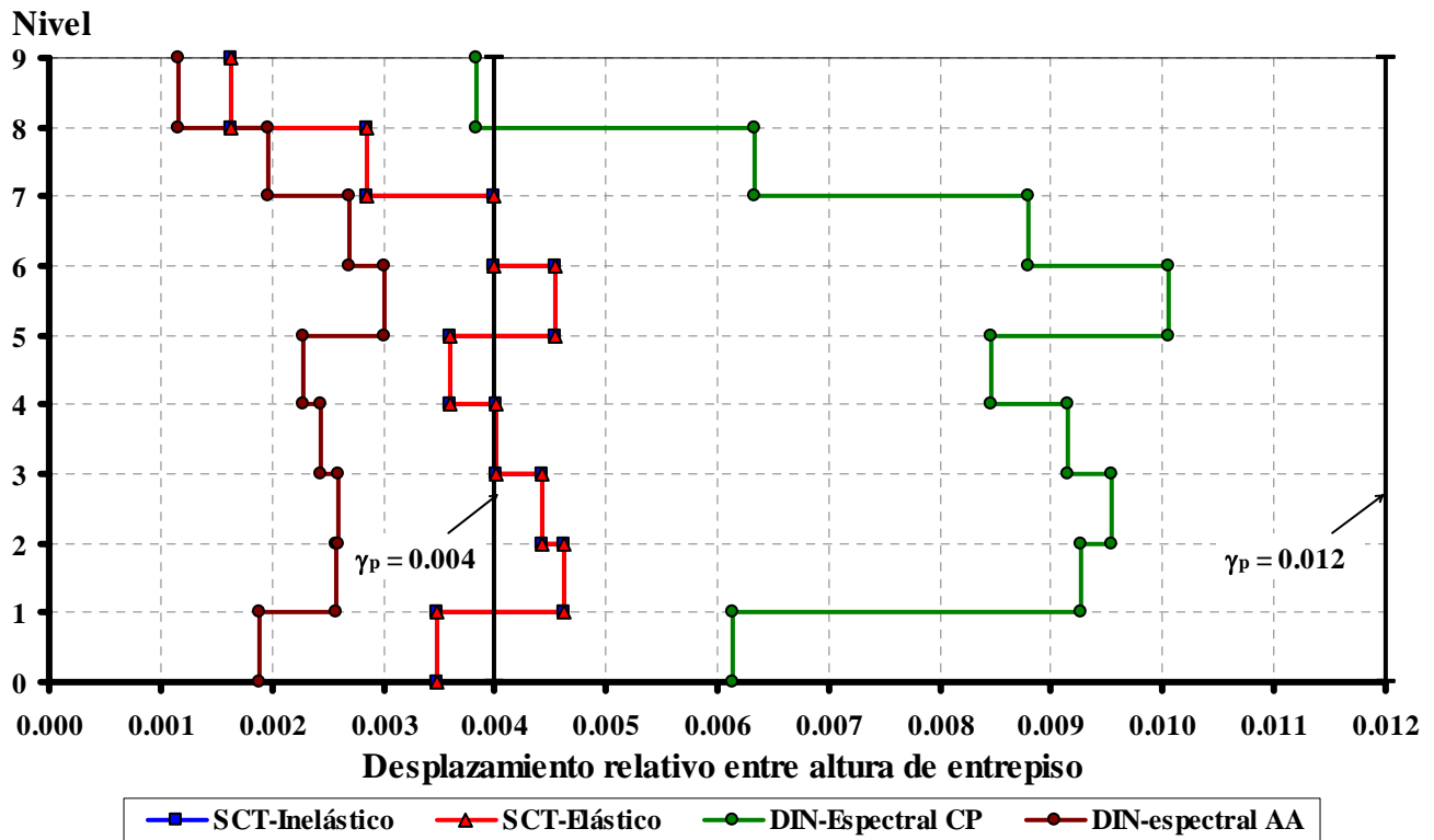
Fig 4.27 Relaciones de desplazamientos horizontales relativos entre altura de entrepiso del marco del eje B del edificio de 9 niveles para Q=2 con \gamma_p \leq 0.004 y 0.012
