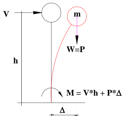
Fig 2.7 Efectos P-Δ
