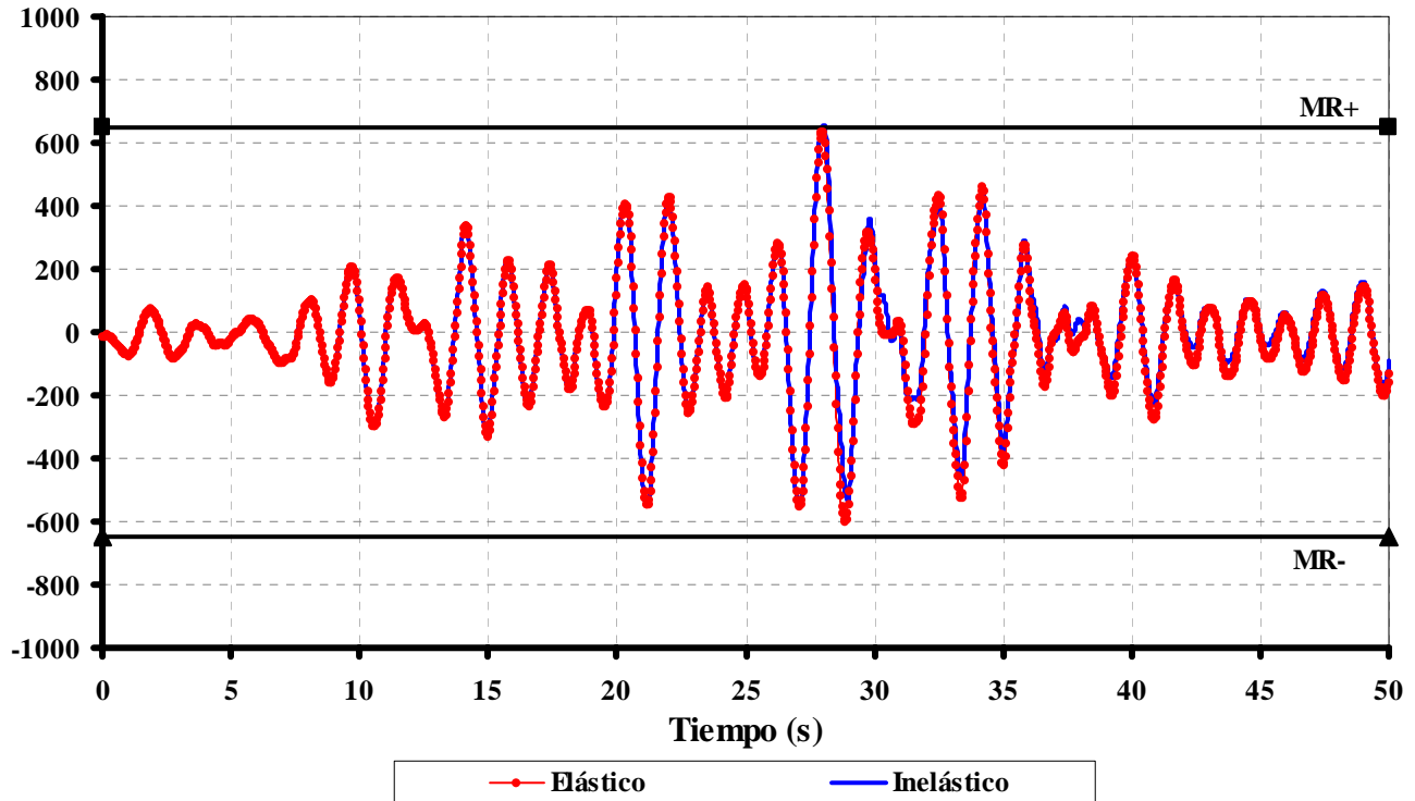
Fig 4.54 Historia de momentos flexionantes y resistencias del extremo izquierdo de la viga 1 del marco del eje B del edificio de 25 niveles para Q=2 y \gamma_p \leq 0.002
