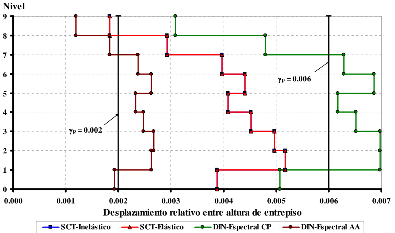
Fig 4.28 Relaciones de desplazamientos horizontales relativos entre altura de entrepiso del marco del eje B del edificio de 9 niveles para Q=4 con \gamma_p \leq 0.002 y 0.006
