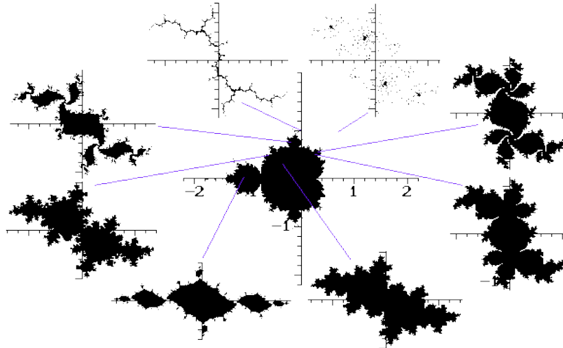
Variedad de los conjuntos de Julia
