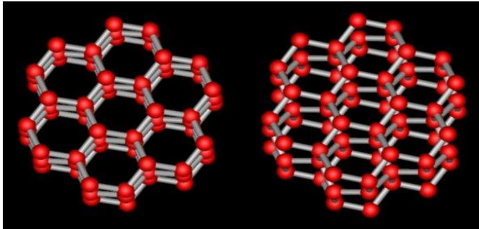
Ordenamiento de las moléculas de agua en un copo de nieve
