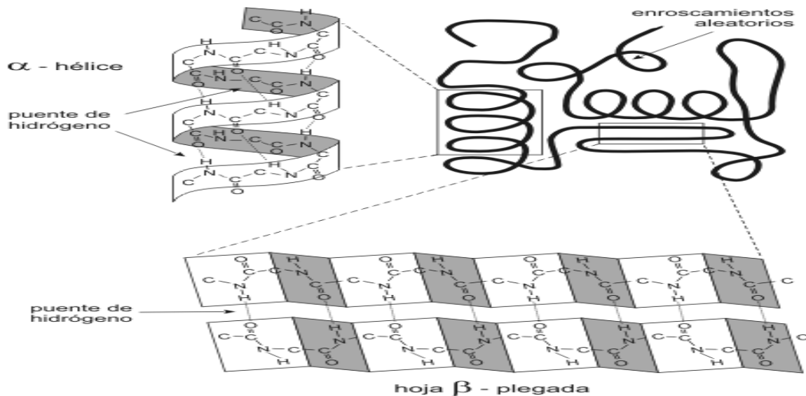
Estructura secundaria
