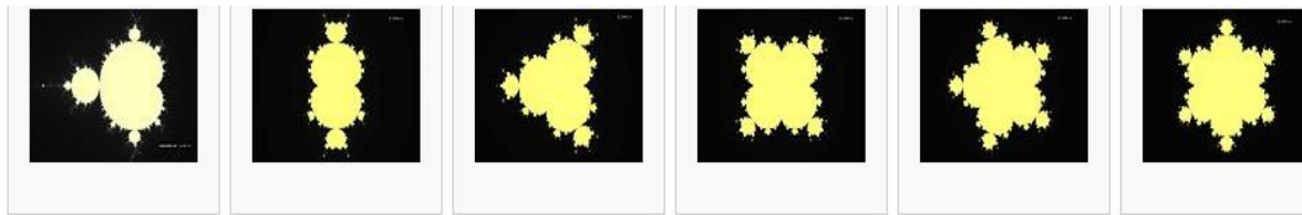
Fractal de Mandelbrot
