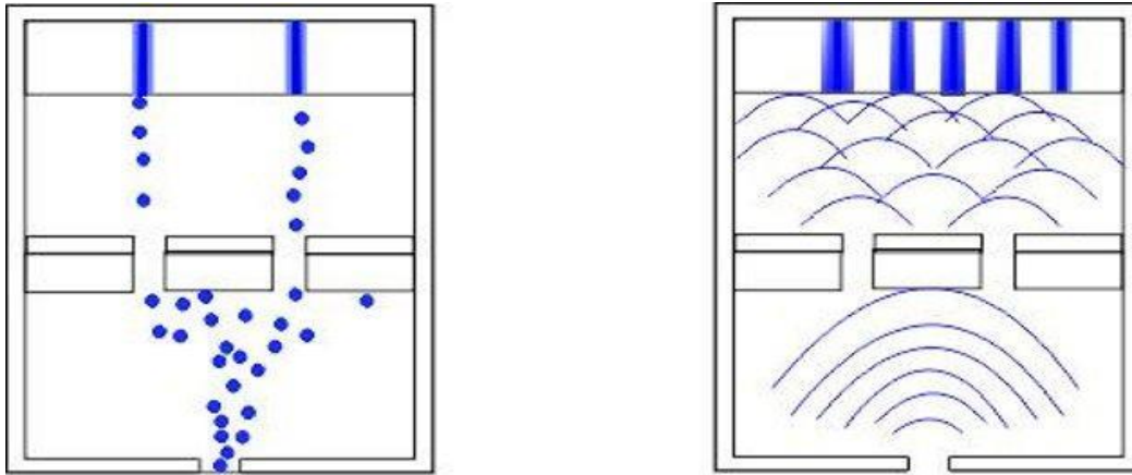
Experimento Young. En el diagrama de la izquierda, así se tendría el patrón con materia macroscópica como con canicas, y en el segundo con ondas.
