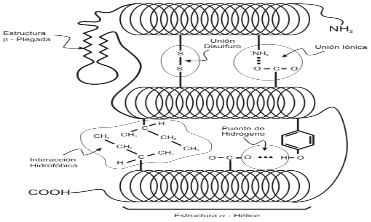
Estructura terciaria
