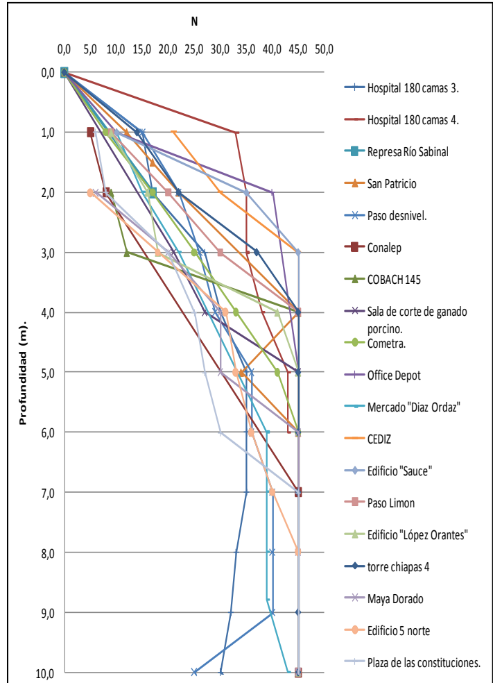
Fig. 3.9. Perfiles de número de golpes (N) de la prueba (SPT), en relación a la Profundidad.
