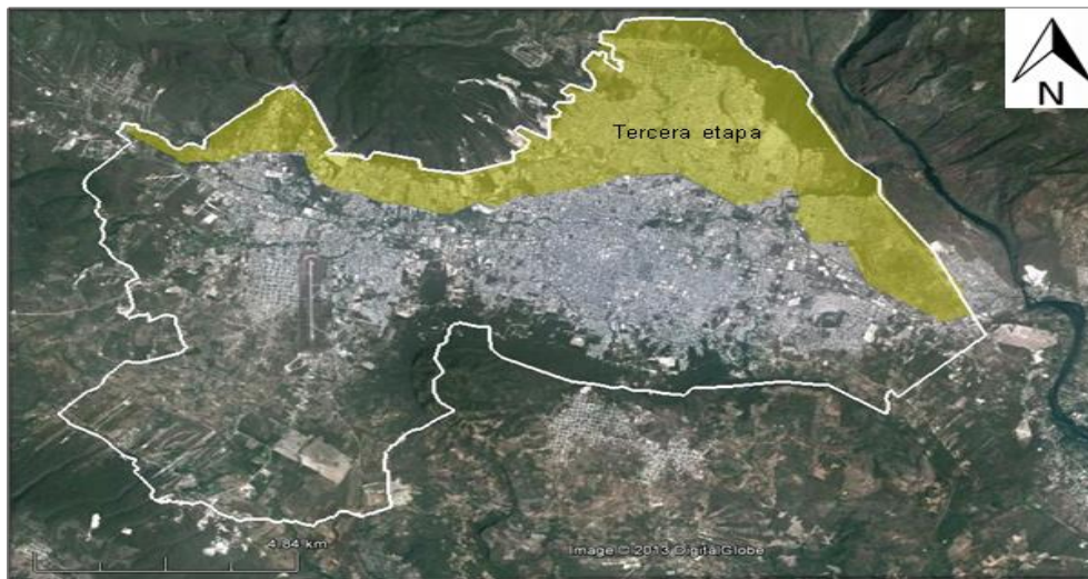
Fig. 3.3. De color amarillo se muestra la región que corresponde a la tercer campaña de monitoreo sísmico.
