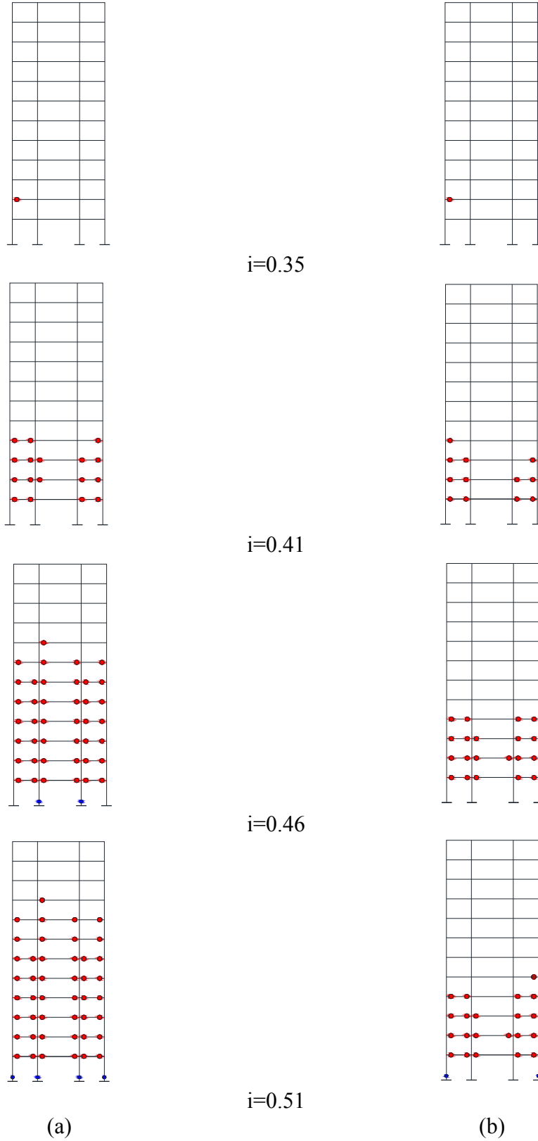
Figura 4.25 Niveles de daño ER12(a) MESID, (b) IDA
