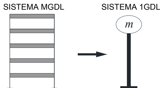
Figura 3.12 Sistema equivalente de 1GDL
