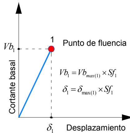
Figura 3.10 Rama elástica de la curva de capacidad
