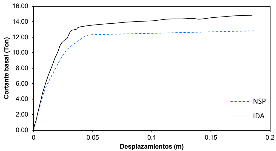
Figura 2.8 Comparación curva IDA y NPS
