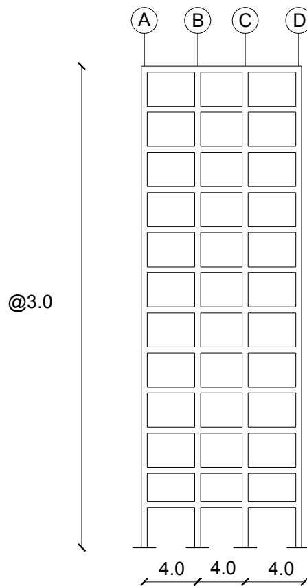
Figura 4.5 Modelo de 12 niveles de acero
