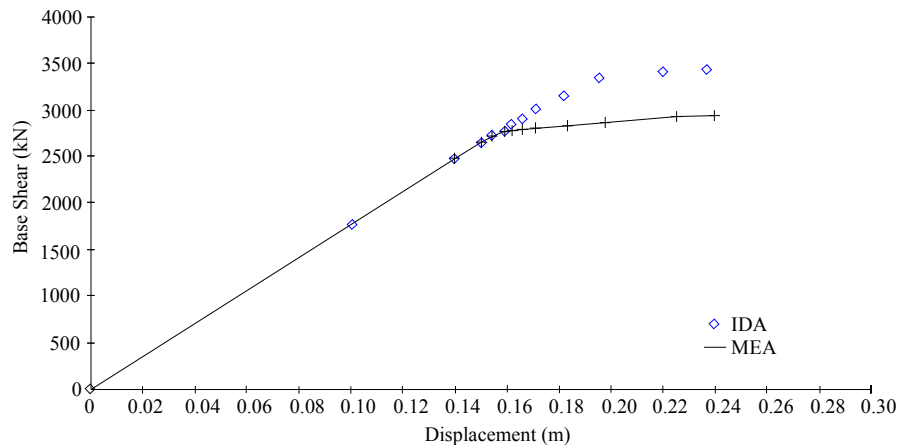
Figura 4.2 Comparación Curvas de capacidad
