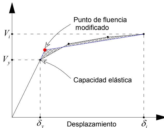
Figura 3.13 Punto modificado de la curva de capacidad
