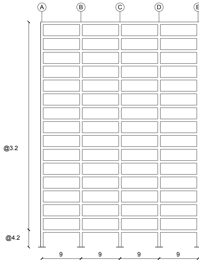
Figura 4.7 Modelo de 16 niveles de concreto reforzado
