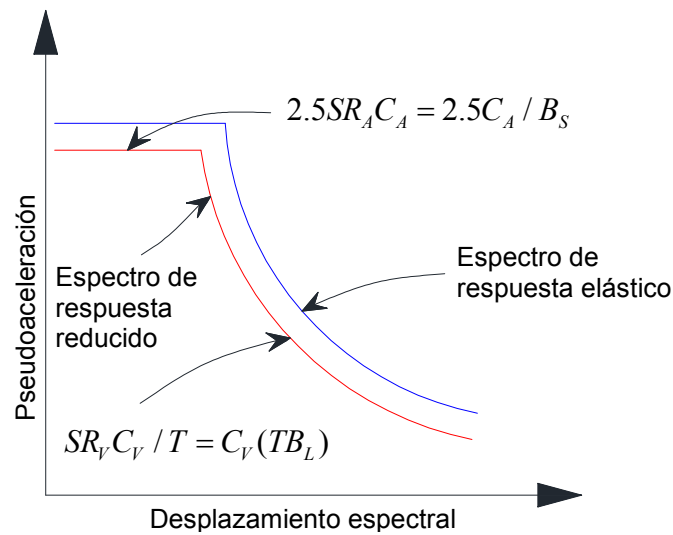
Figura 2.13 Espectro de capacidad reducido
