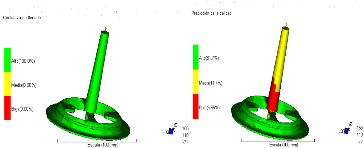
Fig. 3.31 Confianza de llenado Fig. 3.32 Predicción de la calidad
