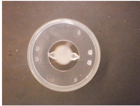
Figura 4.73 Reducción máxima de fisura en la pieza actuador del dosificador.
