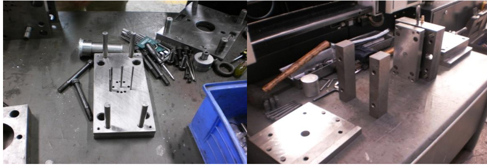
Figura 3.23 Ensamble de Placa de expulsores (izq.) y placas paralelas las cuales contienen a las placas de expulsores (der)
