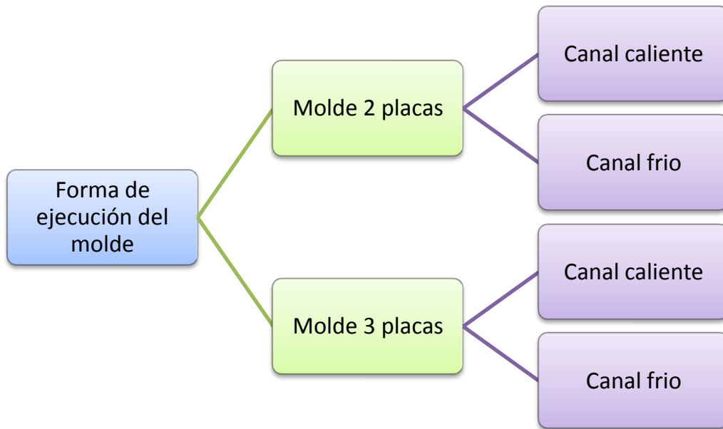
Figura 2.32 Ejecución del molde[18]
