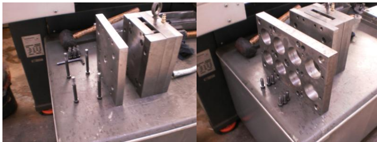
Figura 3.24 Placas de portamolde con tornillos de ensamble (izq.) y placa aumento para ajustar dimensiones a máquina (der)
