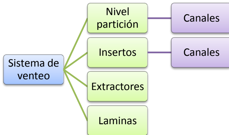
Figura 2.37 Sistema de venteo[18]
