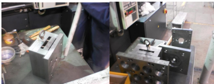
Figura 3.22 Ensamble de Portamolde (izq. base de placas de cavidades con placas de expulsores, der ensamble con placas de anillo centrador placas fijas)
