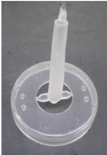
Figura 4.33 Moldeo de la pieza actuador del dosificador completa.
