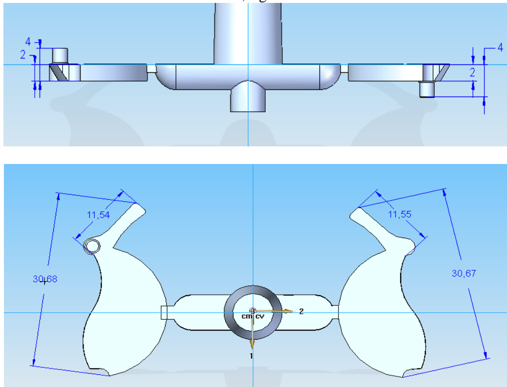
Figura 4.60 Dimensiones críticas para la pieza paleta X (izquierda) y paleta Y (derecha) del dosificador, unidades en [mm]
