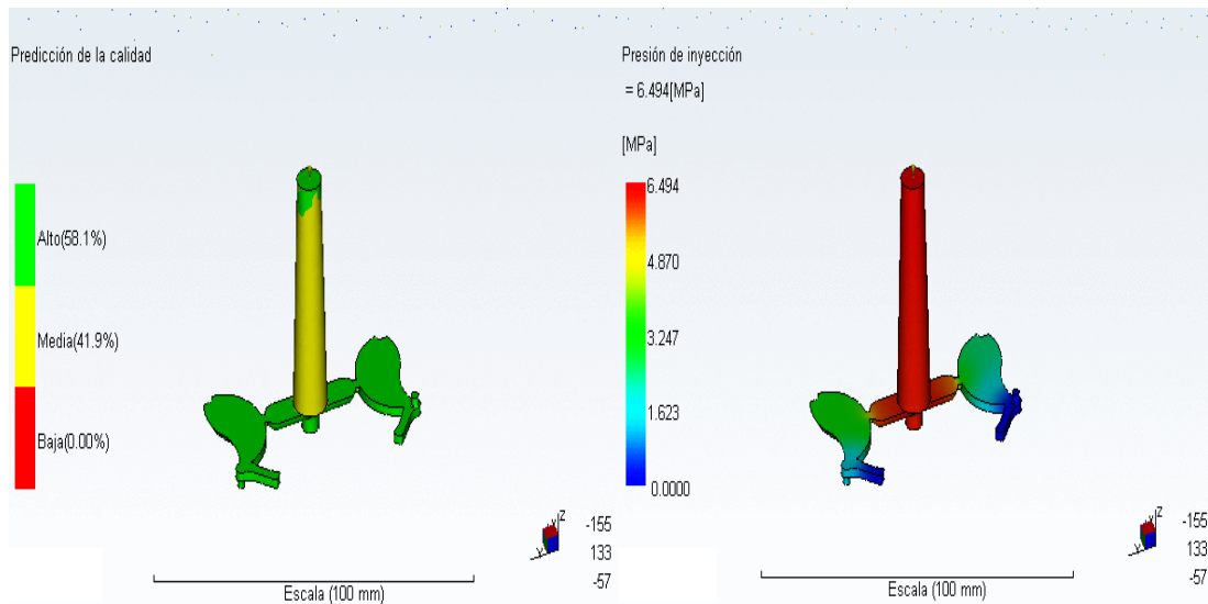
Figura 3.12 Predicción de la calidad
