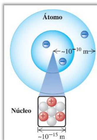
Figura 7 - Modelo atómico 10
