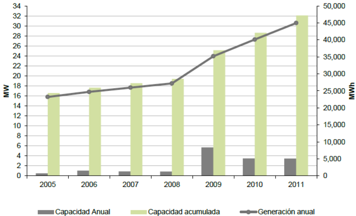
Grafica 5 - Evolución de la capacidad instalada y energía generada con sistemas FV en México 29
