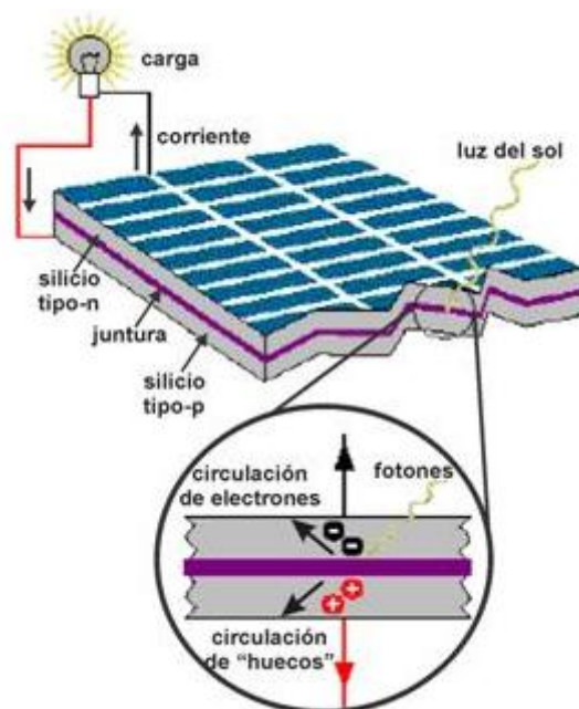
Figura 9 - Celda FV 12
