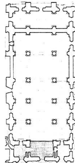
Ilustración 12 Planta de la Compañía de Jesús de Guanajuato, tipología 1A de las iglesias jesuitas. 54
