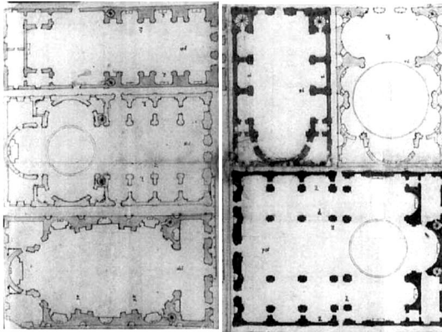
Ilustración 8 Plantas de iglesias jesuitas, de acuerdo con De Rosis 50
