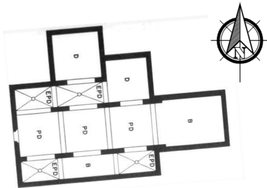
Ilustración 83 Planta esquemática de la iglesia de Belén 209
