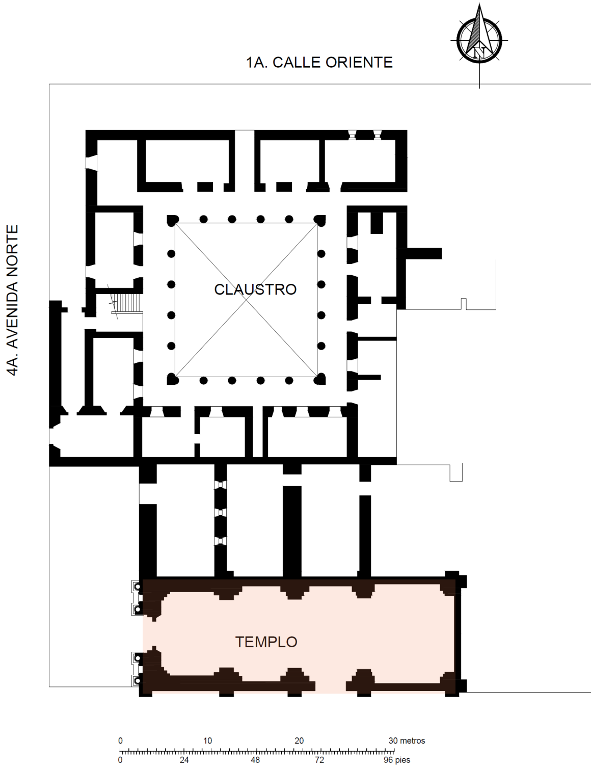
Ilustración 122 Planta Convento y Templo de Santa Teresa
