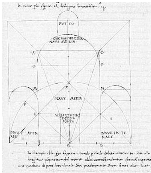
Ilustración 57 Proporción de una iglesia, de acuerdo con Francesco di Giorgio Martini
