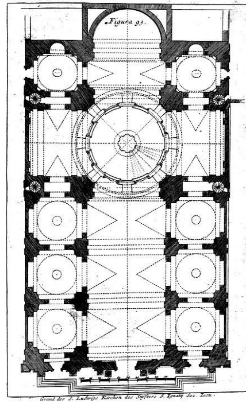
Ilustración 49 Planta de la St. Ludwigs Kirchen, obra de Orazio Grassi, que se encuentra en el tratado de perspectiva de Andrea Pozzo, y que corresponde a la tipología 1.
