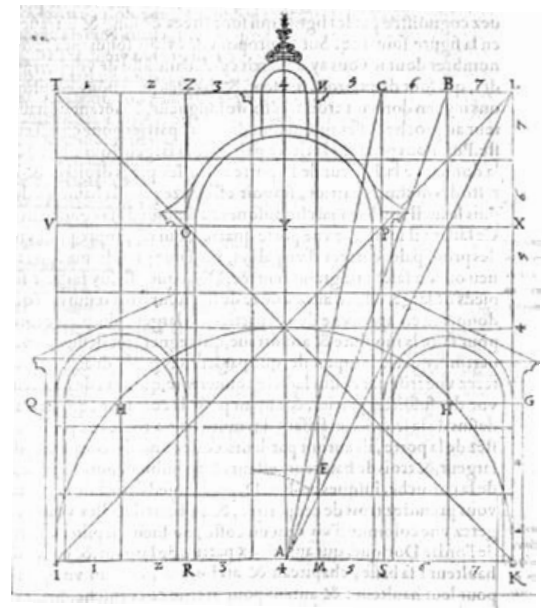
Ilustración 58 Proporción de un templo abovedado de acuerdo con Philibert de l'Orme, 1567.
