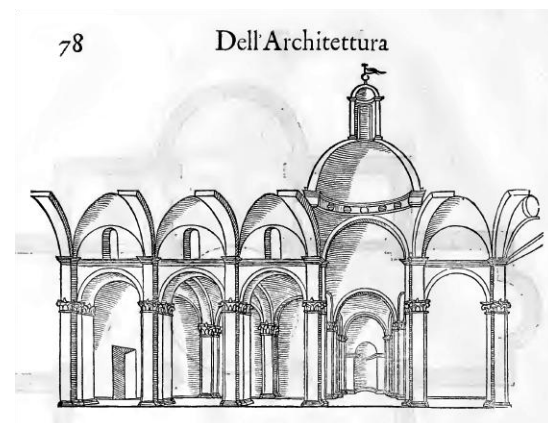
Ilustración 104 Planta, elevación y sección de un templo, de acuerdo a Cataneo
