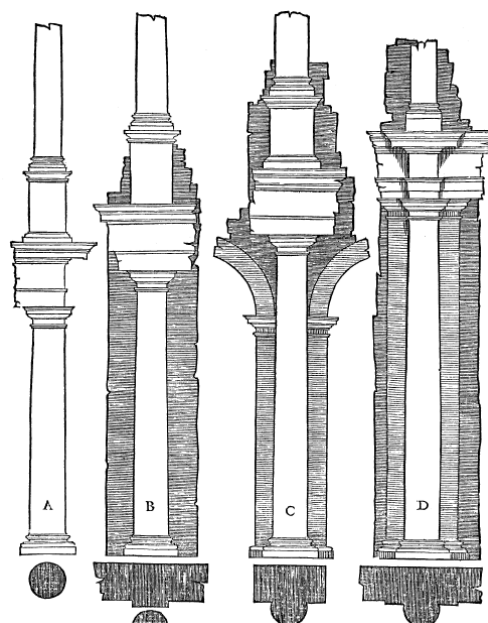
Ilustración 113 Libro cuarto lámina LXVIII, Resistencia de las columnas de acuerdo con su colaboración con el muro, según Serlio
