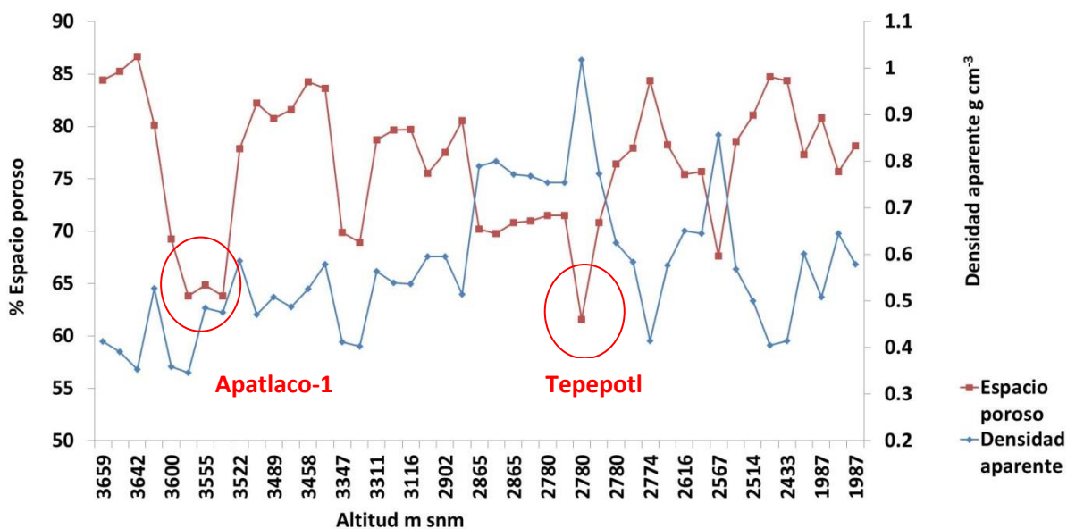
Figura 15. Relación entre densidad aparente y espacio poroso a través del gradiente altitudinal.
