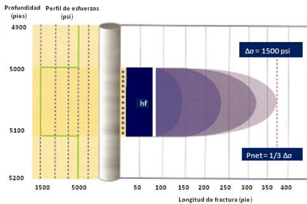
FIGURA 2.14.- Comportamiento de la altura y la longitud de una fractura en función de la presión neta y el diferencial de esfuerzos. 1
