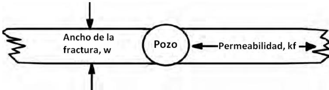
FIGURA 2.11.- Definición de conductividad de la fractura. 3
