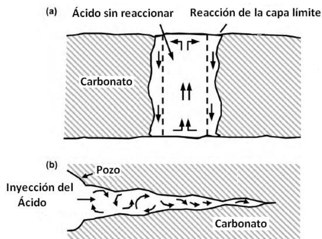
FIGURA 2.20.- Comportamiento del ácido fluyendo en la fractura. 4
