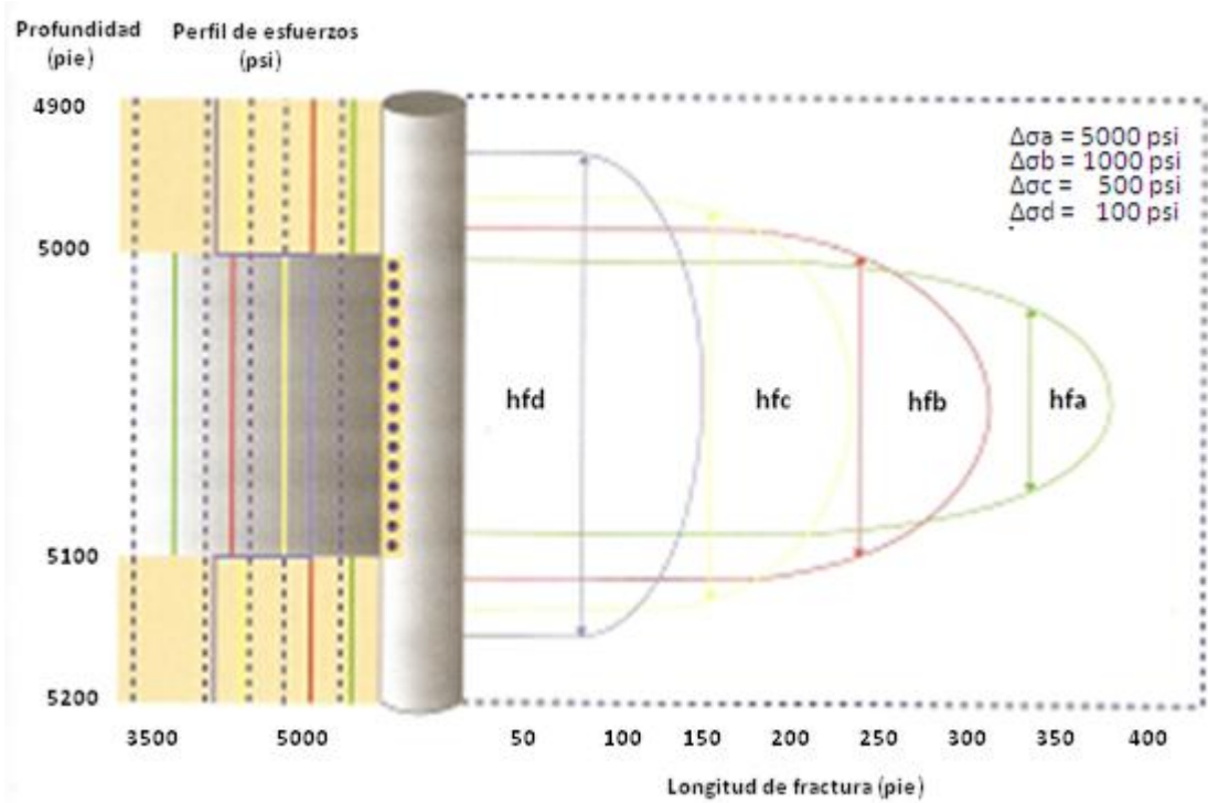
FIGURA 2.13.- Longitud y altura de una fractura vs perfil de esfuerzos. 1
