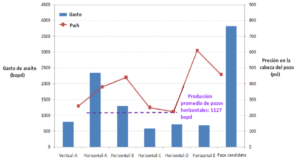
FIGURA 4.2.- Comparación del comportamiento de la producción de pozos verticales y horizontales en el mismo campo.
