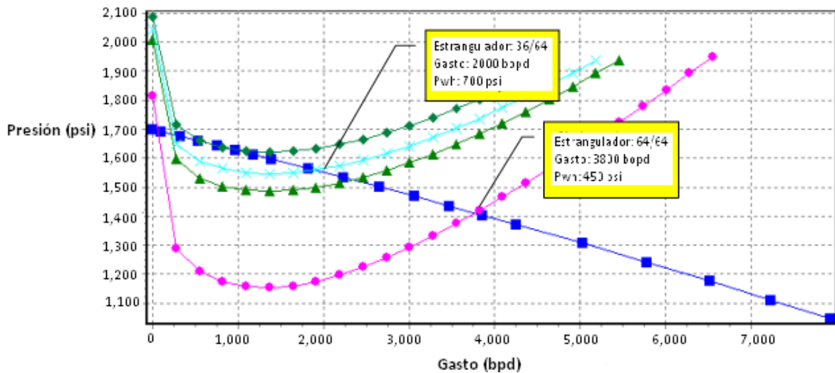
FIGURA 4.3.- Análisis Nodal indicando un IP de 13 bopd/psi.
