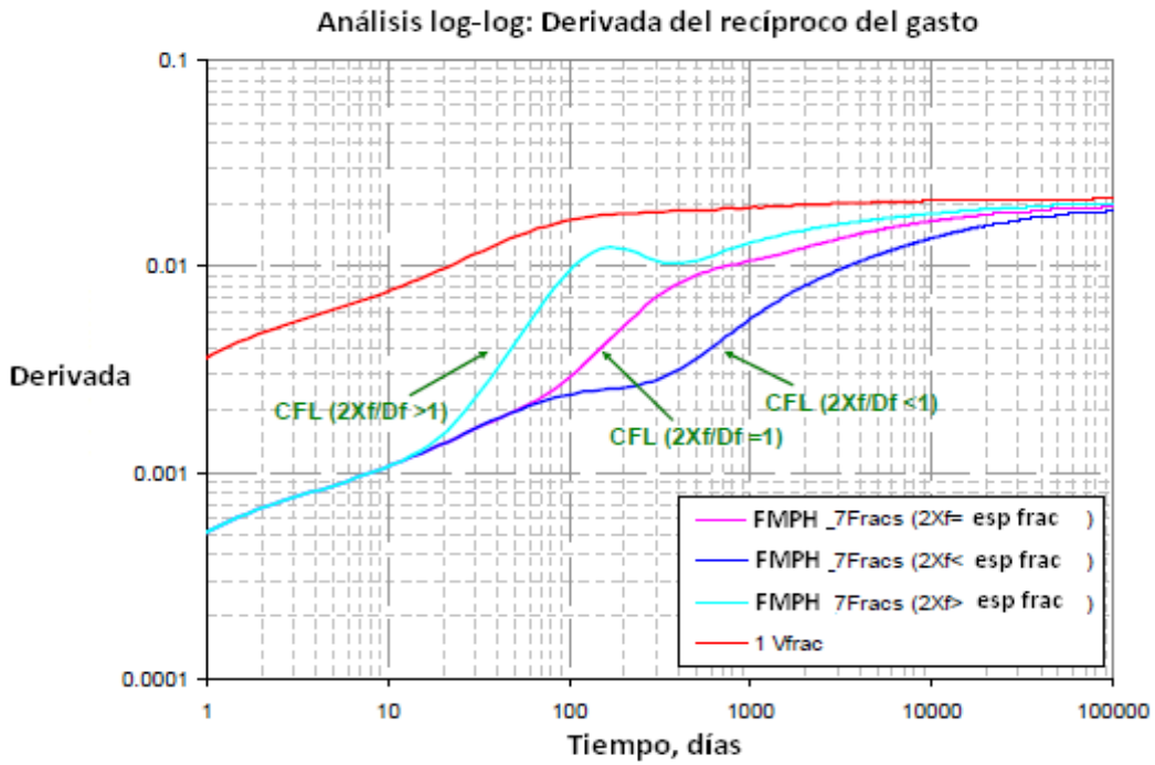
FIGURA 3.25.- FMPH con siete fracturas transversales. 20
