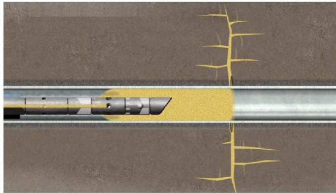
FIGURA 3.9.- Esta figura muestra la lechada concentrada de apuntalante siendo bombeada a través de la TF y se combina con el fluido de tratamiento acarreado el fluido sin apuntalante siendo bombeado por el espacio anular para formar una mezcla con la concentración deseada de apuntalante y el gasto de inyección total de fluido de tratamiento. Este proceso puede usarse en una perforación y con una desviación del bache de apuntalante o con una camisa mecánica de estimulación para fracturar cada una de las etapas pero intercaladas. 18
