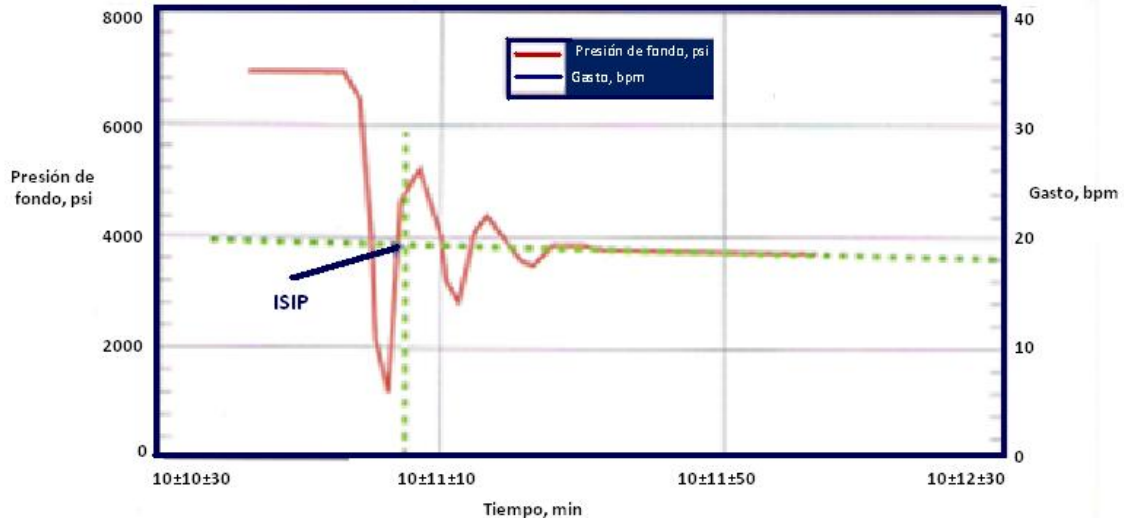
FIGURA 2.8.- Determinación de la presión instantánea al detener el bombeo (ISIP) 1
