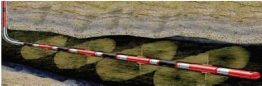
FIGURA 3.13.- Ejecución de SSP. 26
