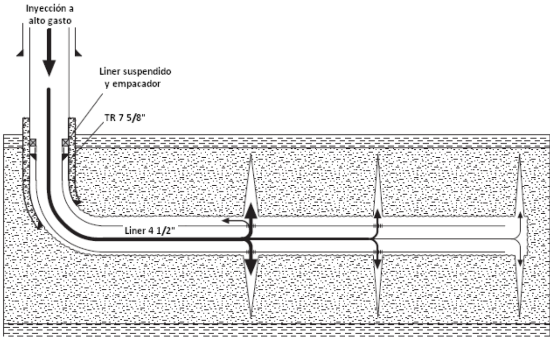
FIGURA 4.6.- Tercera etapa del re-fracturamiento con FDT
