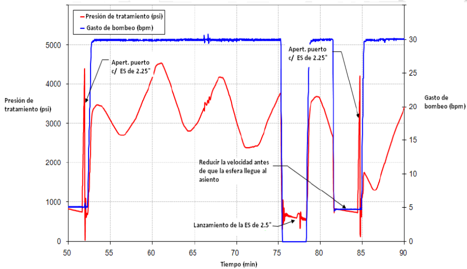
FIGURA 4.1.- Respuesta de la presión cuando las esferas son lanzadas hacia los asientos.
