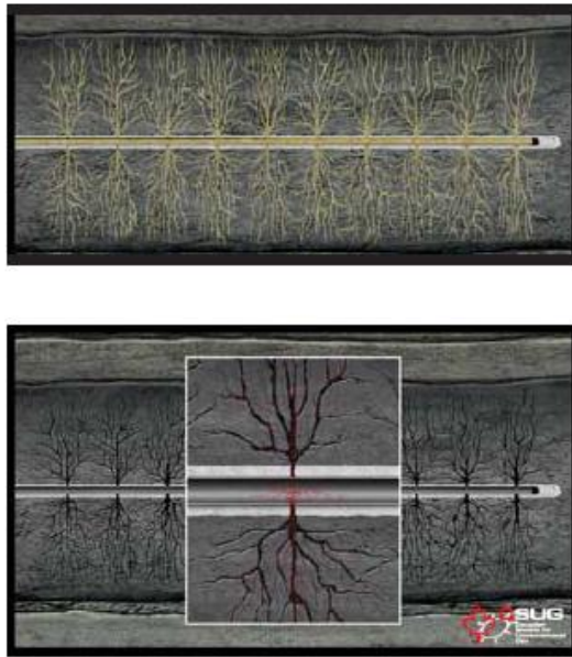
FIGURA 2.2.- Fracturamiento Multietapas. 7
