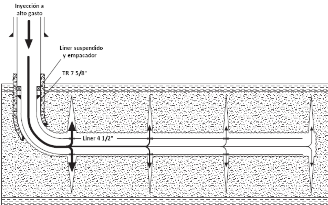
FIGURA 4.7.- Cuarta etapa del re-fracturamiento con FDT
