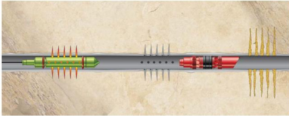
FIGURA 2. 7.- Ilustración del Perf & Plug, donde se utiliza un Bridge Plug para aislar las etapas que se van a fracturar y se perfora para crear las fracturas en las etapas deseadas. El número y tamaño de las perforaciones para cada etapa a menudo son limitados para asegurarse de que cada etapa reciba el fluido de tratamiento. 18
