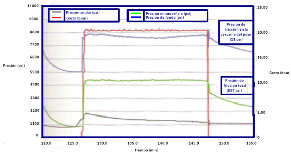
FIGURA 2.10.- Presiones de fricción total y en la cercanía del pozo para una prueba de calibración. 1
