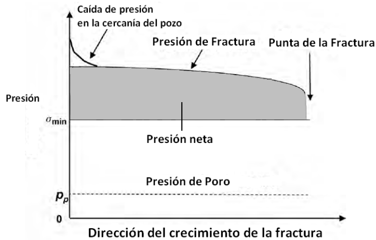
FIGURA 2.9.- Perfil de presión en una fractura apuntalada. 3
