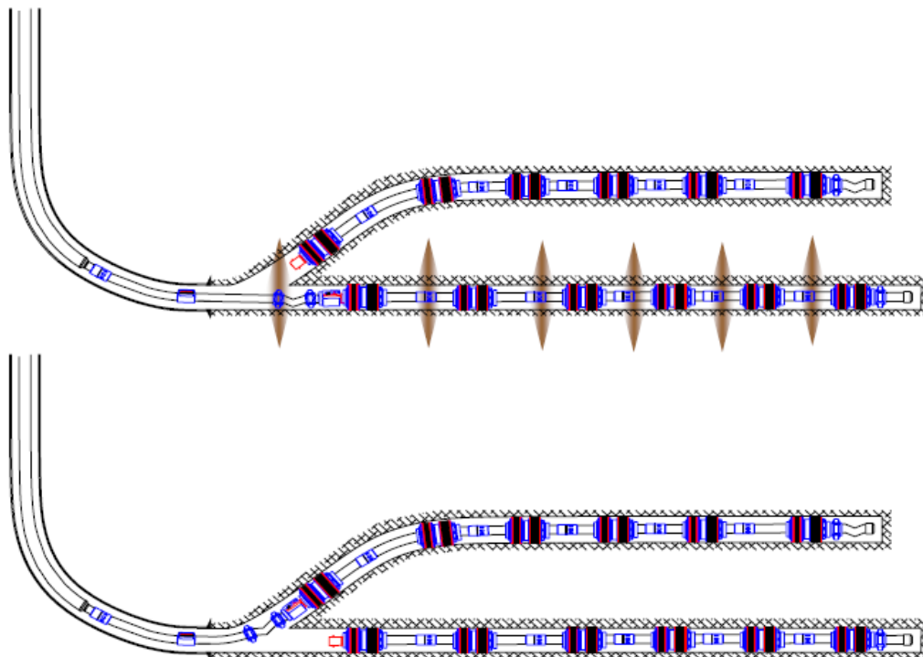
FIGURA 4.9.- Pozo multilateral con un fracturamiento de cinco etapas, esto en cada una de las extensiones del pozo multilateral.
