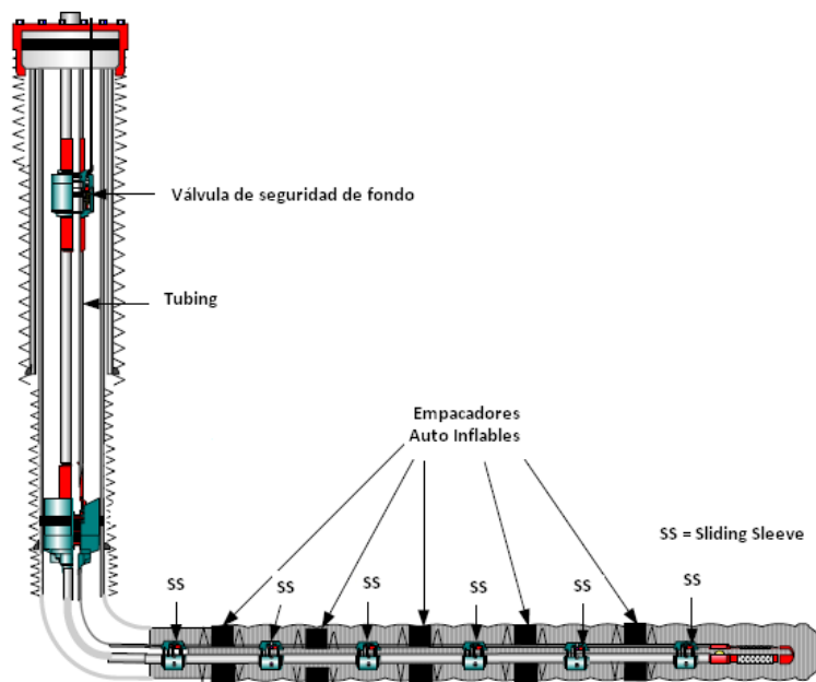
FIGURA 3.23.- Sistema de fracturamiento con aislamiento mecánico. 20
