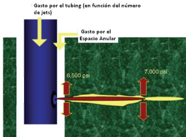
FIGURA 3.1.- Proceso hidrojet. 26
