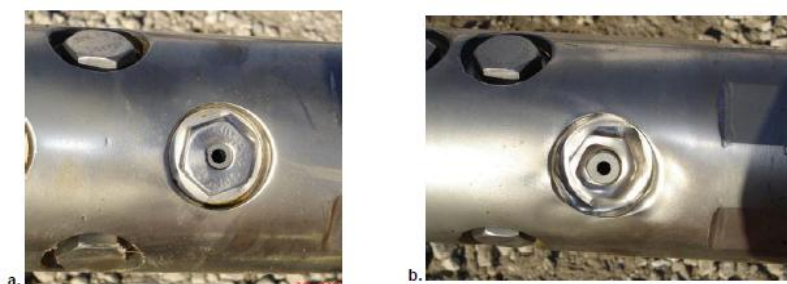
FIGURA 4.10.- a) Dos de los tres jets, mostrando muy poco desgaste. b) Uno de los tres jets tenía mucha erosión en el protector contra salpicaduras.
