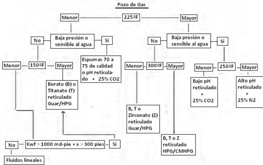
FIGURA 2.17.- Proceso de selección del fluido fracturante. 4
