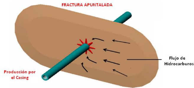
FIGURA 3.2.- Las perforaciones con el sistema hidrojet tienen un ID grande y no están dañadas, con los métodos convencionales de perforación pueden reducirse las restricciones en la producción. 11
