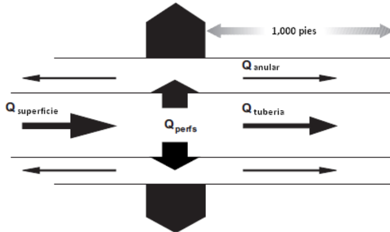
FIGURA 4.8.- Varios caminos de flujo que el fluido puede tomar cuando este llegue al intervalo perforado.
