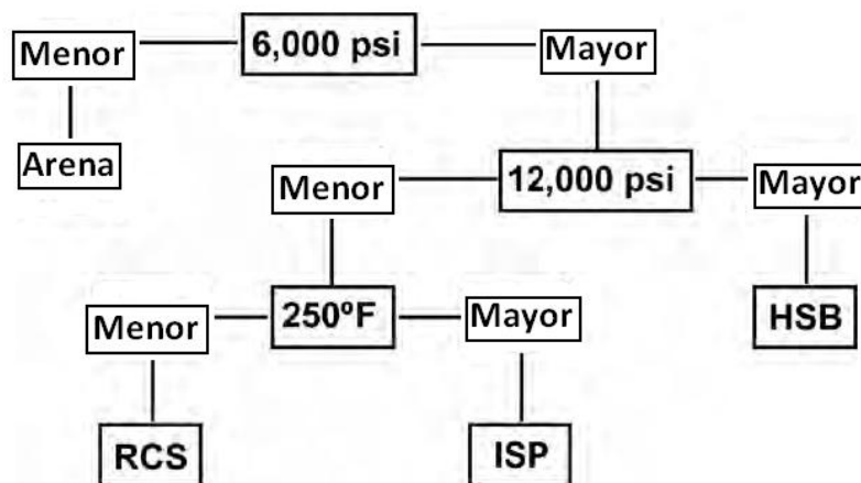
FIGURA 2.18.- Selección del apuntalante considerando la presión de cierre, Economides. 4
