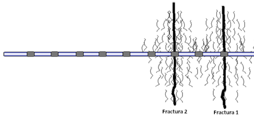
FIGURA 3.16.- Fractura principal con fracturas "stress-relief" no conectadas. 18
