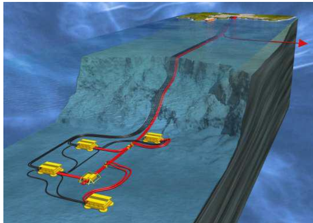
FIGURA 8 CONFIGURACIÓN SUBMARINA PARA LA EXPOLTAIÓN DEL CAMPO ORMEN LANGE.
