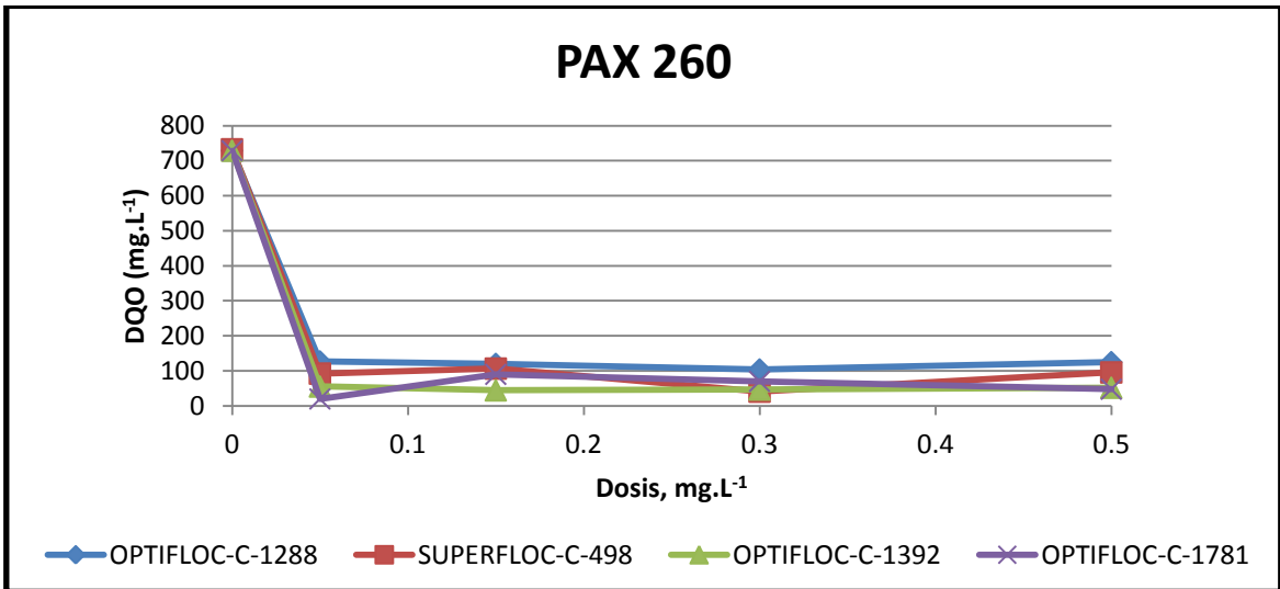
Gráfico H.1 Resultados de las pruebas con combinaciones de coagulantes y floculantes catiónicos para la remoción de DQO.
