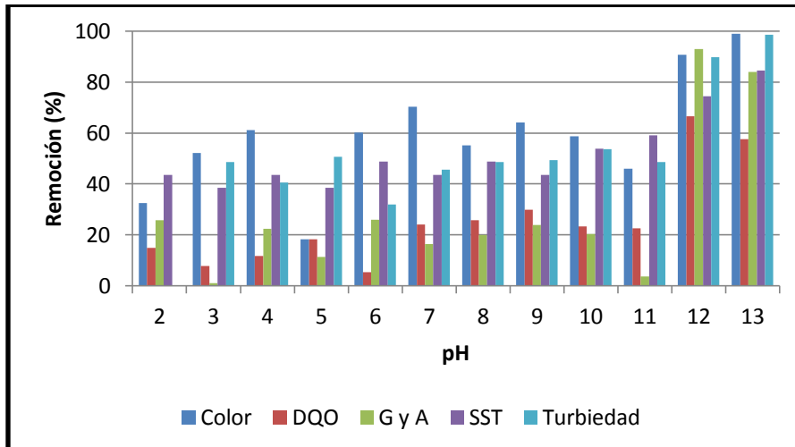
Gráfico 5. 2 Remociones obtenidas por la variación del pH sin adición de un coagulante.
