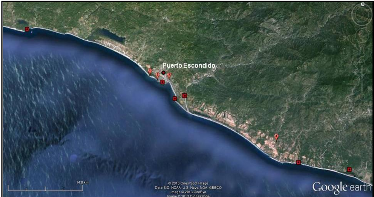
Fig. 1. 4 Imagen de la Sierra Madre del Sur y ubicación de sitios estudiados en las terrazas de la Región de Puerto Escondido, Oaxaca (Modificado de Google Earth, 2012)
