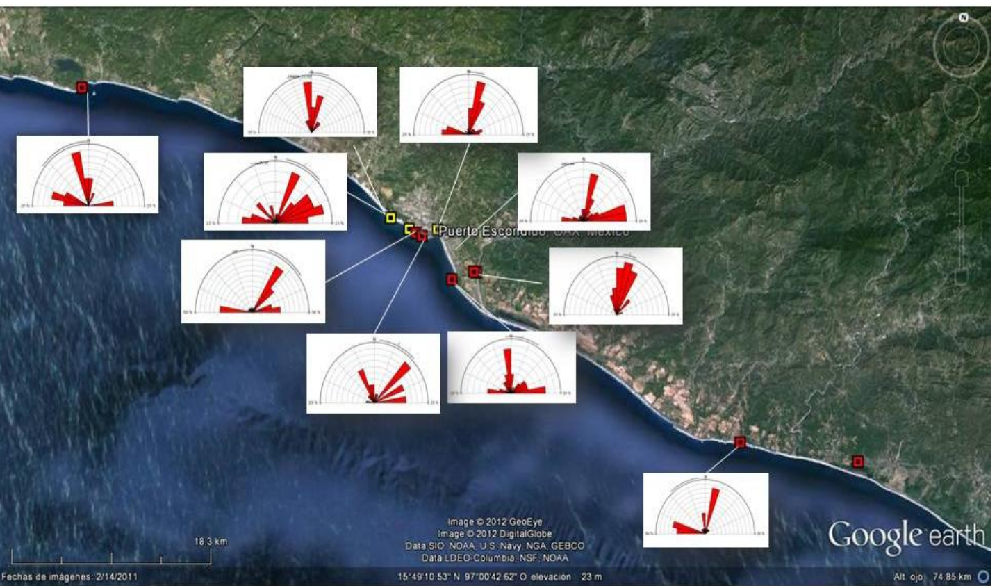
Fig. 4.48 Figura donde se muestran las rosetas estructurales de las direcciones de las fracturas de cada afloramiento.
