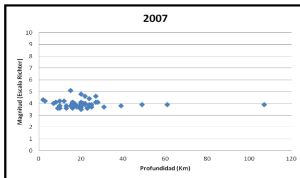
Fig. 4.42. Actividad sísmica en el año del 2007, en las Costas de Oaxaca.
