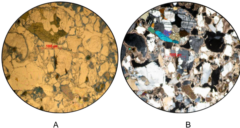
Figura 2.25 Microfotografías de la muestra de Playa Coral B Acantilado.
