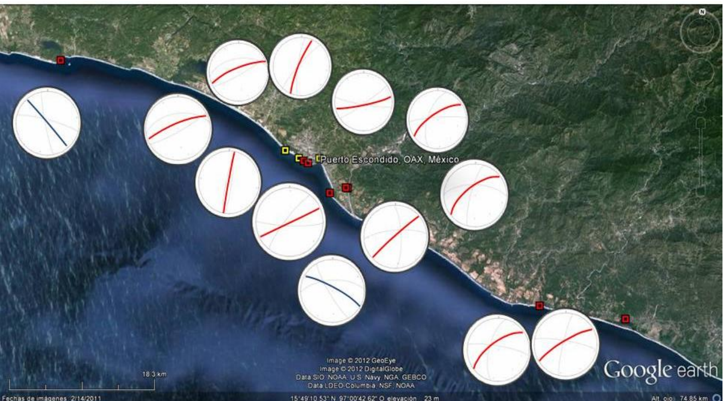
Fig. 4.49 Esquema con representaciones estereográficas se muestra la dirección de máximo esfuerzo como resultante de la familia de fracturas que se encuentra en cada afloramiento.
