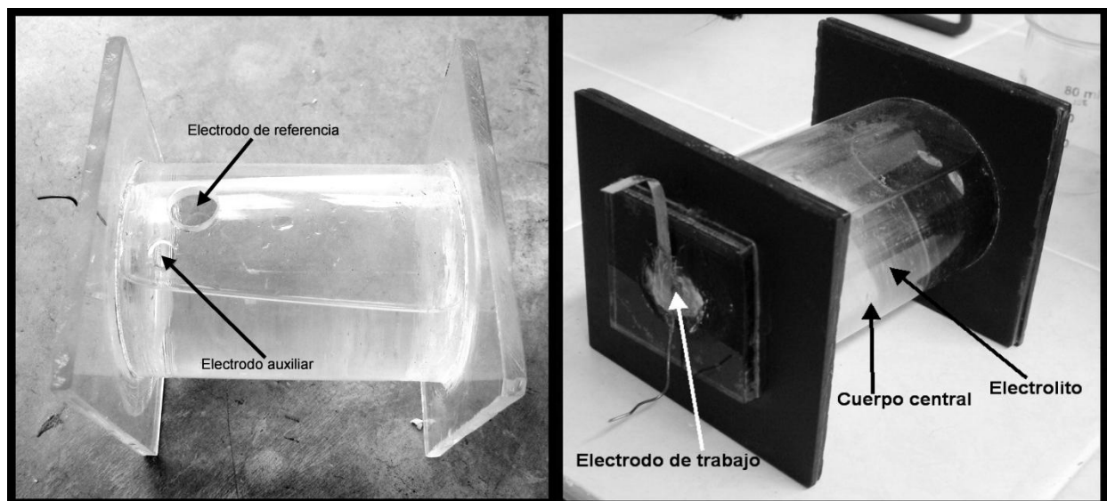
Figura 2.11 Vistas panorámicas de las celdas electroquímicas utilizadas.
