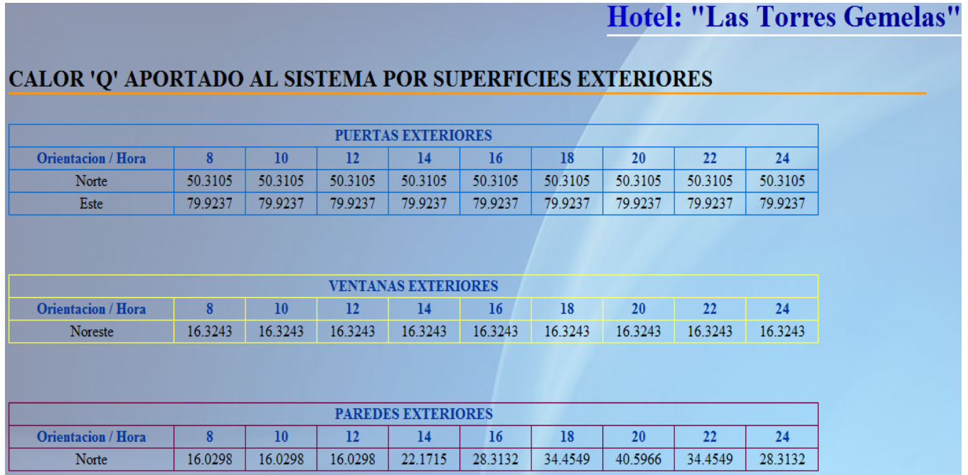
Figura 31. Calor aportado al sistema por superficies exteriores
