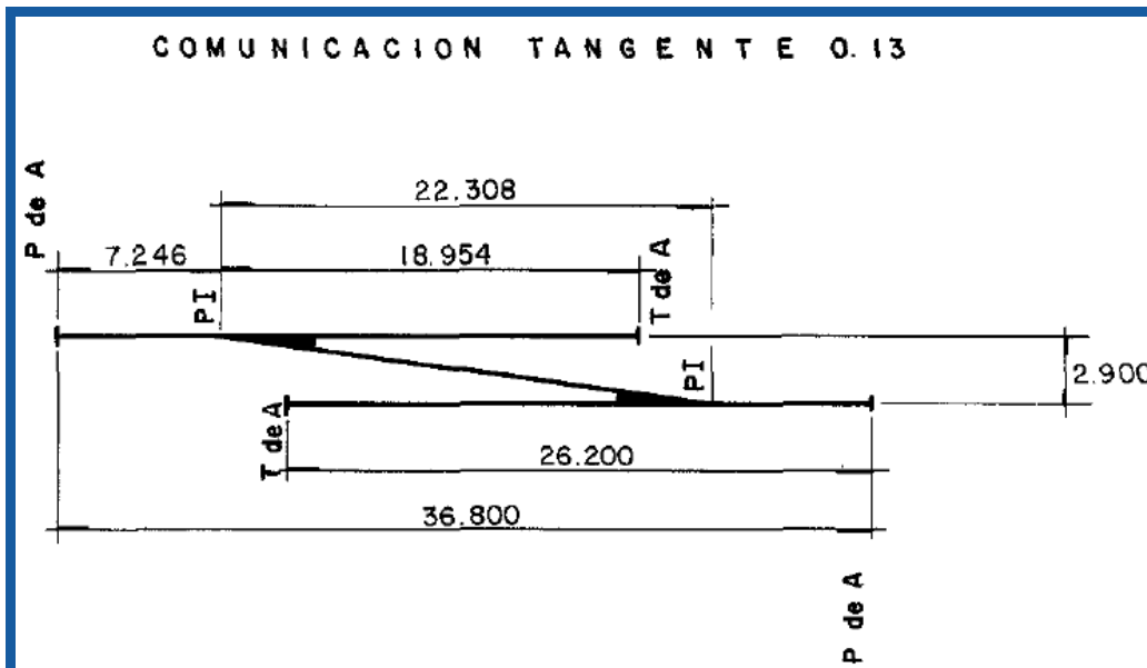
Esquema de aparato de vía (entrevía de 2.9 m) extraído del libro 2.02.02 Vías principales del la bibliografía “Especificaciones Para el Proyecto y Construcción de las Líneas del Metro de la Ciudad de México”
